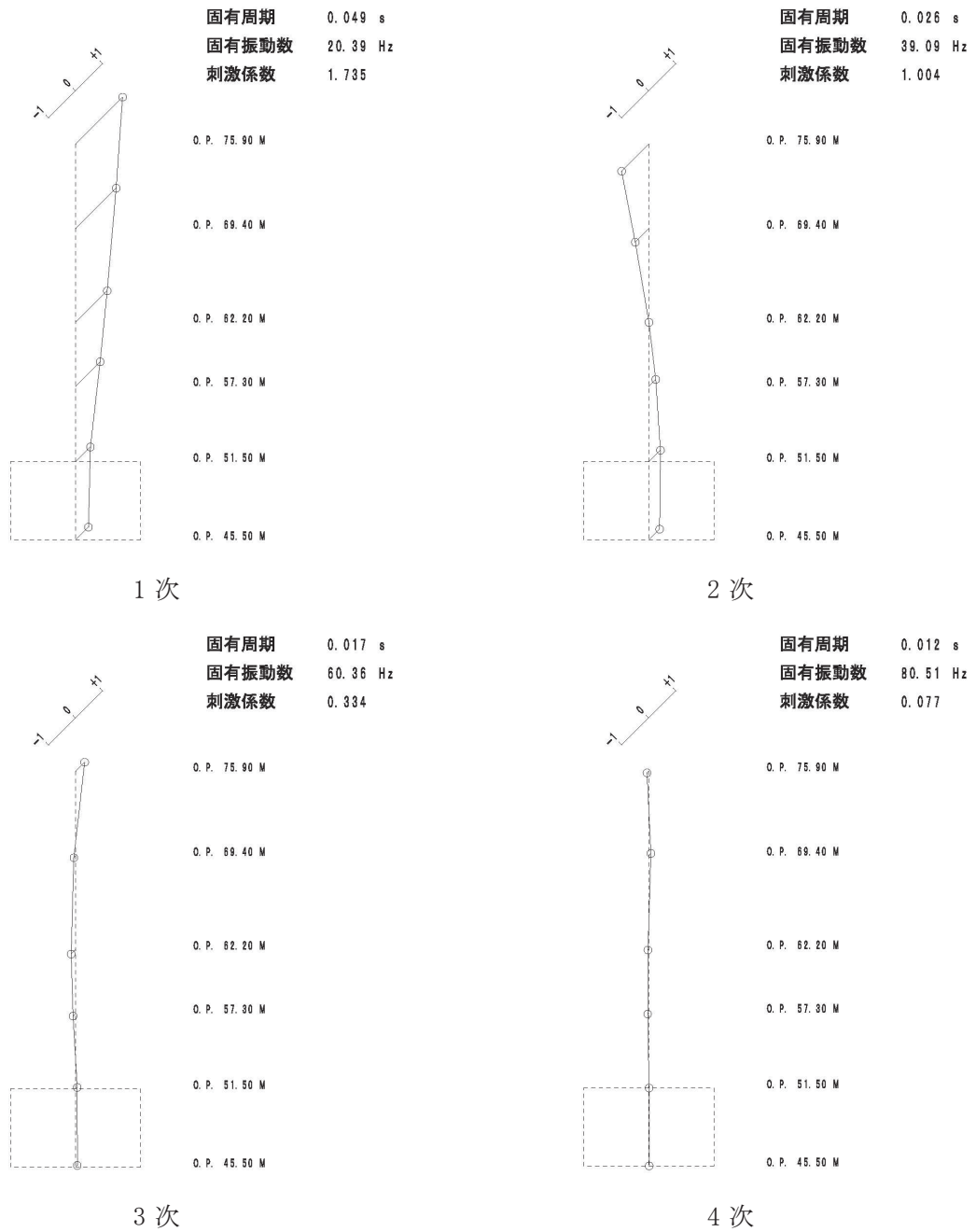
図 4-6 刺激関数図 (ケース 2) (UD 方向 1 次~4 次)
