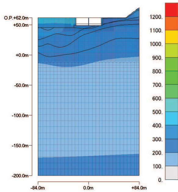
最大加速度分布 (最大値:626.69 cm/s 2 )
