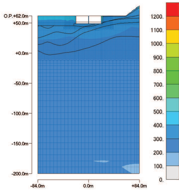
最大加速度分布 (最大値:712.77 \text{cm/s}^2 )
