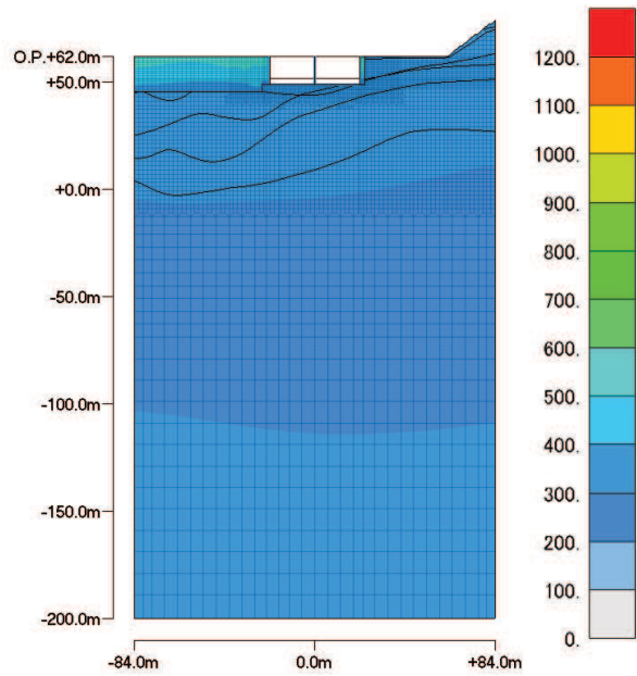
最大加速度分布 (最大値:713.4 cm/s 2 )
