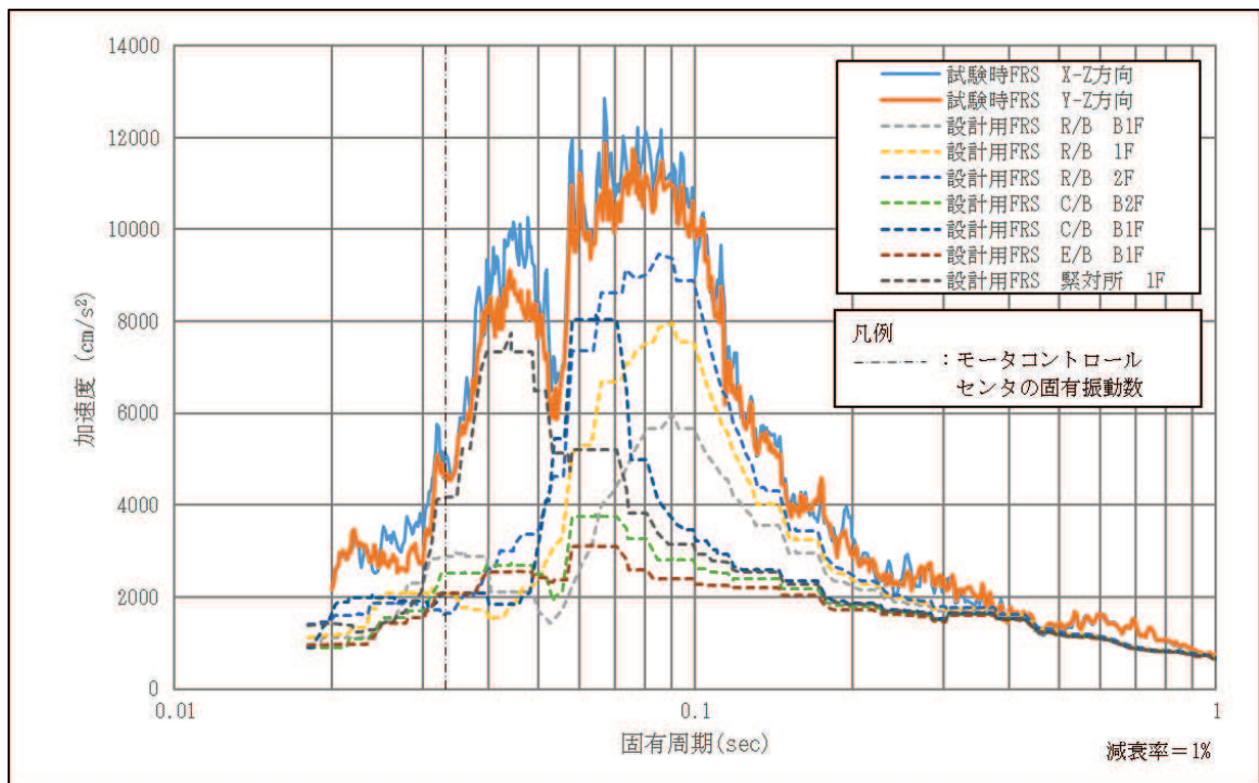
図 4-4 試験時 FRF と設計用 FRF との比較 鉛直方向 (モータコントロールセンタ) *
