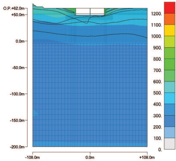
最大加速度分布 (最大値:921.23 \text{cm/s}^2 )
