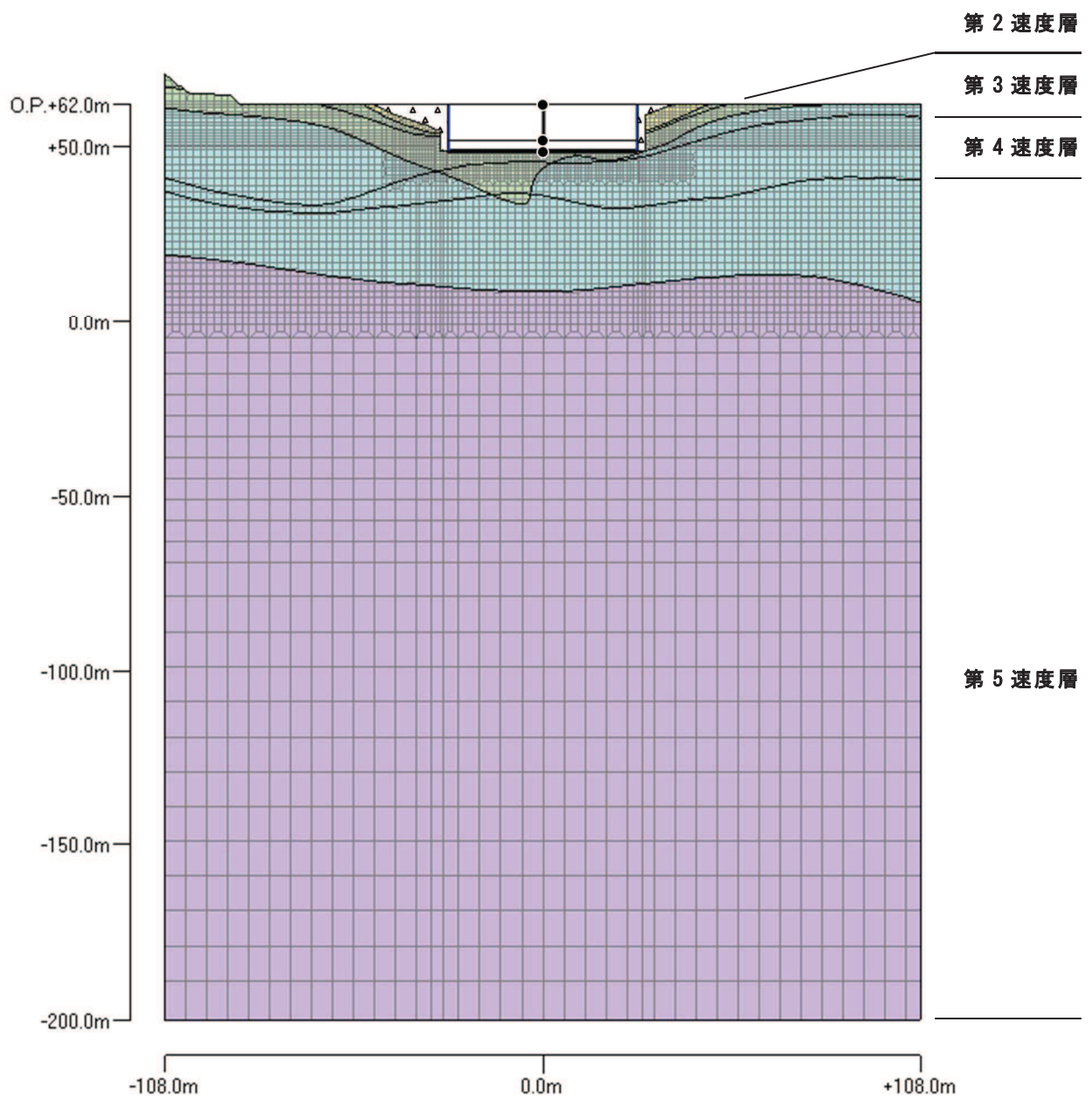
図 2.3.3-9(2) 第2 保管エリアの地震応答解析モデル (二次元)
