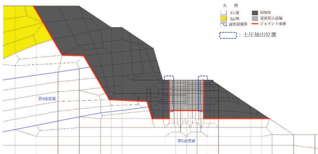
図 8.5-28 地震時増分土圧及び周面せん断土圧抽出位置
