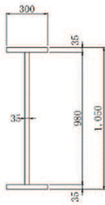
図 5.7-8 中央支柱の断面形状
