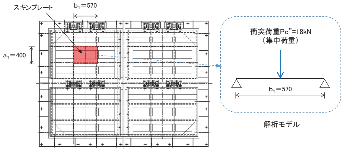
図 5.5-12 スキンプレートのモデル図
