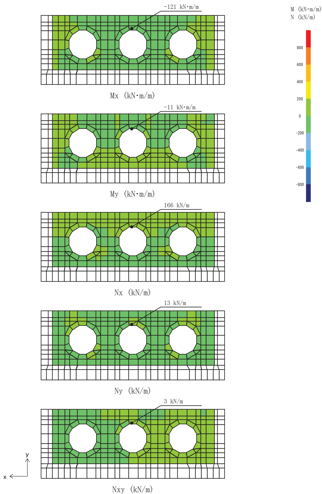
図 11.1-4 曲げ・軸力系の破壊に対して最も厳しい照査値となる解析ケースの断面力分布図 (東壁, 解析ケース③, S s - F 2 (-+), t=28.44s)
