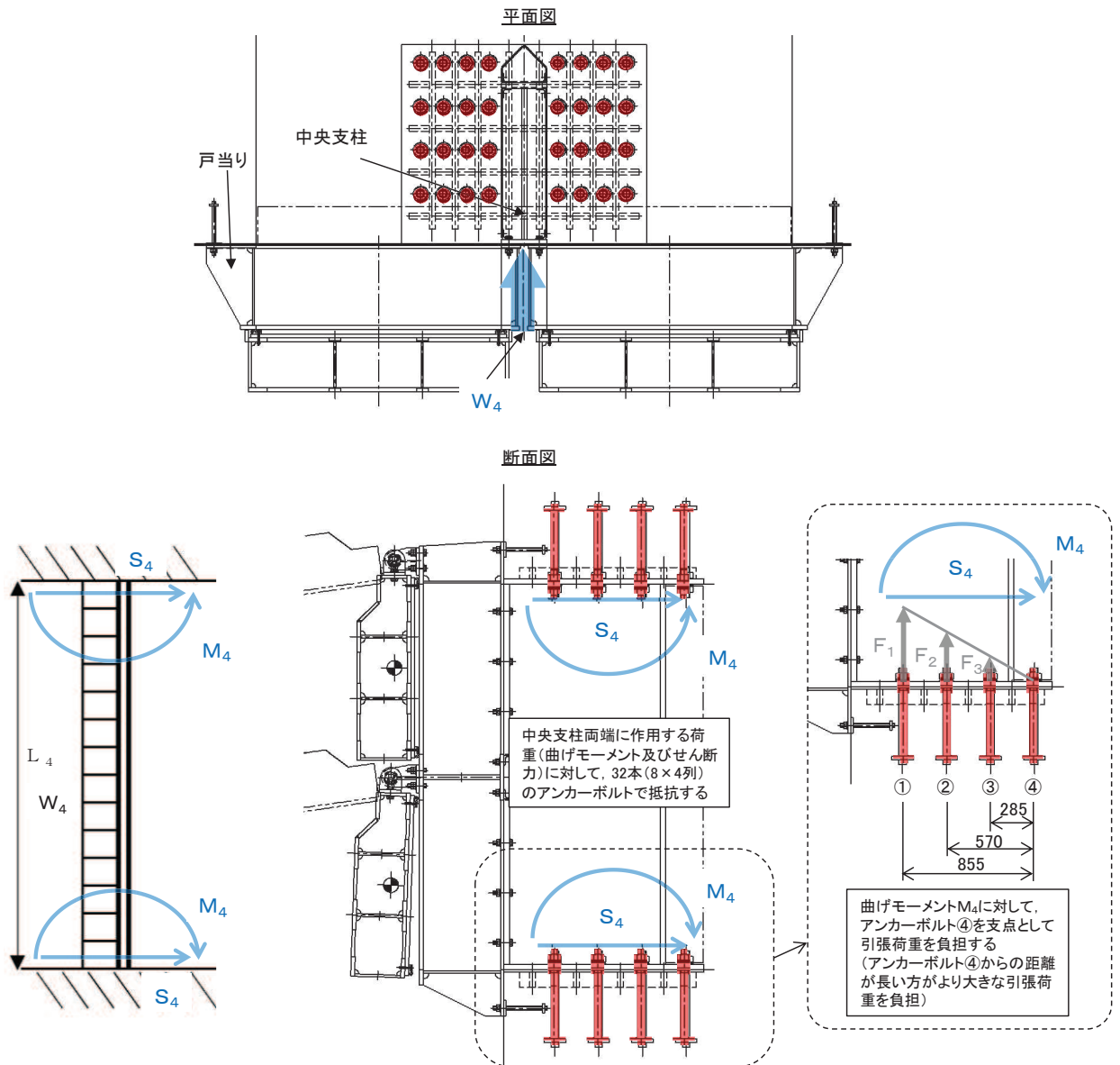
図5.5-4(2) 中央支柱（アンカーボルト）の構造図及びモデル図
