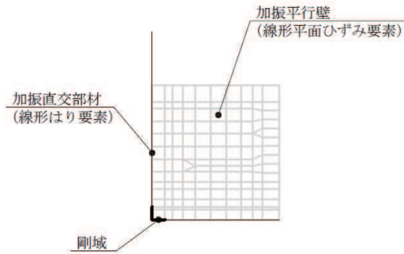
図 8.5-4 構造部材のモデル化
