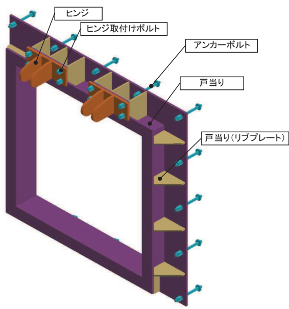
図 1-1(2) 構造概要図 (扉体及び固定部)
