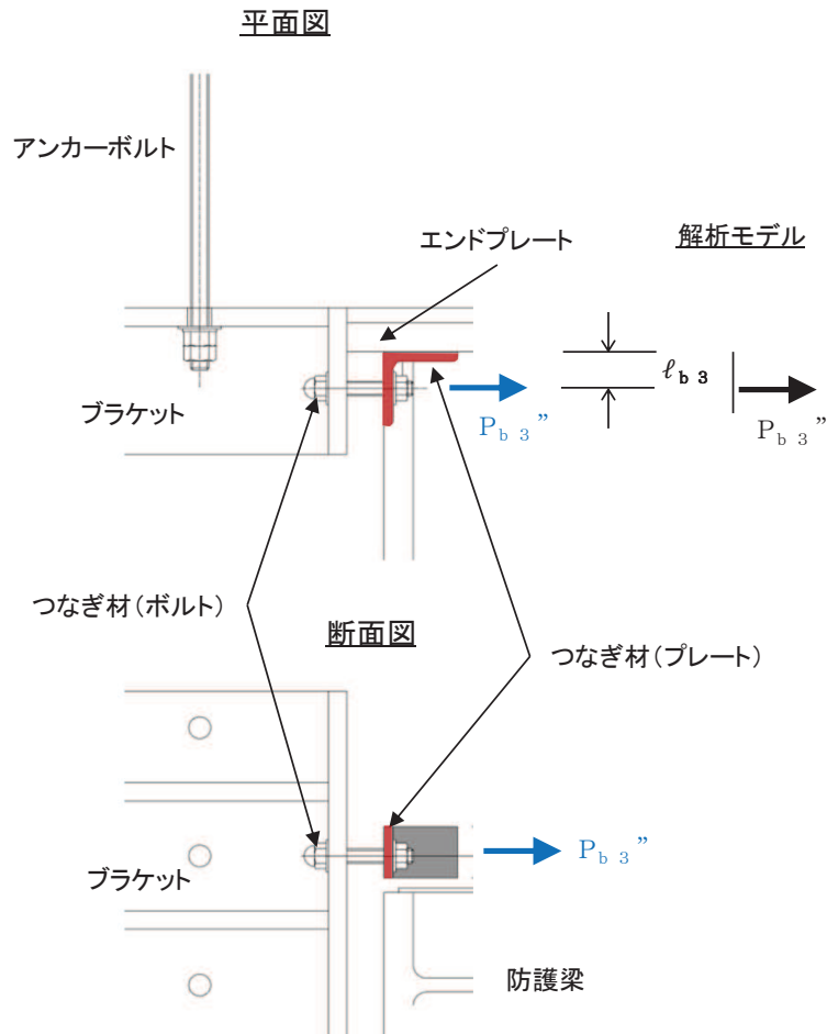
図 5.7-18 防護梁（つなぎ材（プレート））の寸法の小さい漂流物検討概要図
