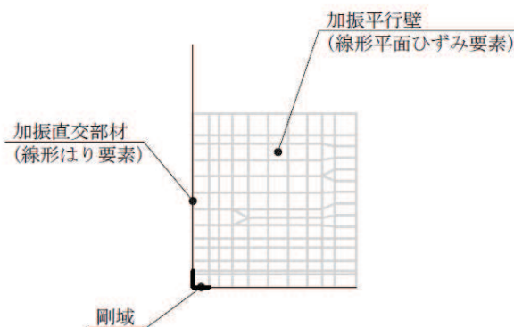
図 8.5-29 構造部材のモデル化
