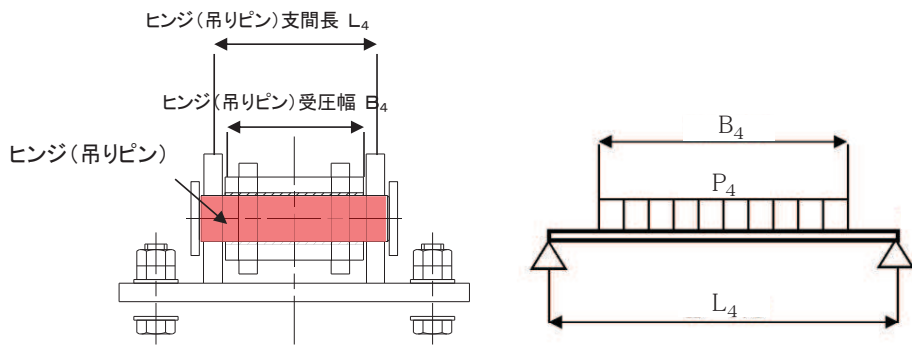
図 5.7-9(1) ヒンジ（吊りピン）の構造図（水路縦断方向）
