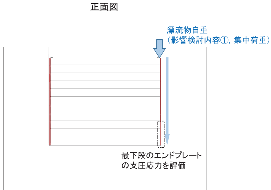
図 5.7-19 エンドプレートの引き波時の検討概要図
