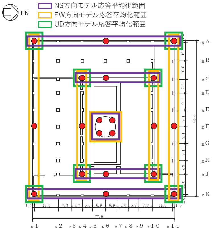
図 3-14(2) 代表節点の位置と応答平均化範囲 (0. P. 33. 2m)
