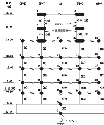
図 3-12(6) せん断スケルトンカーブ上の最大応答値 (NS 方向) (6/6)
