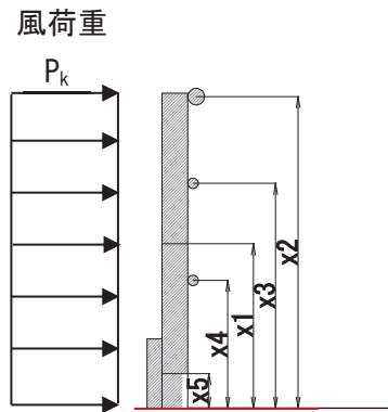
図 5-24 手摺支柱荷重 概要図
