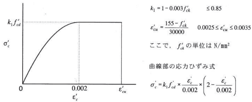
図 3.2.1 コンクリートの応力-ひずみ曲線
