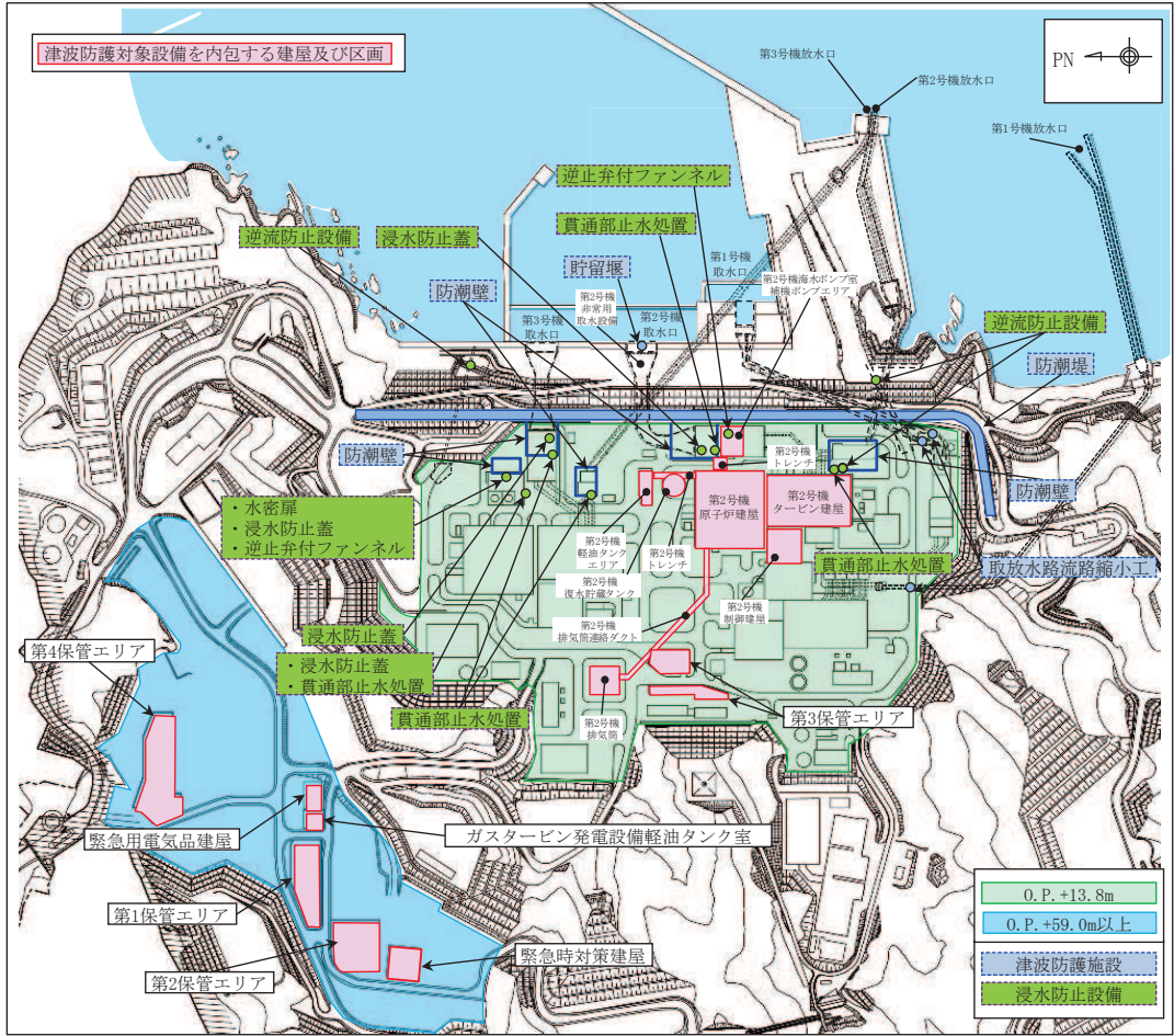
図 3-22 津波防護施設及び浸水防止設備の位置の概要図
