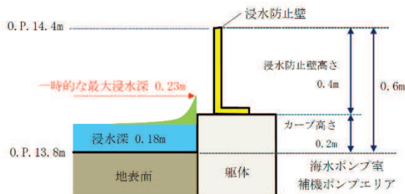
浸水イメージ (A-A 矢視)
