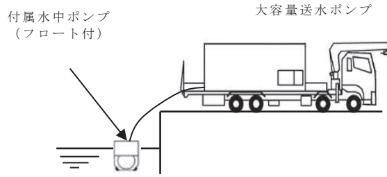
図 3-53 大容量送水ポンプ吸込みイメージ
