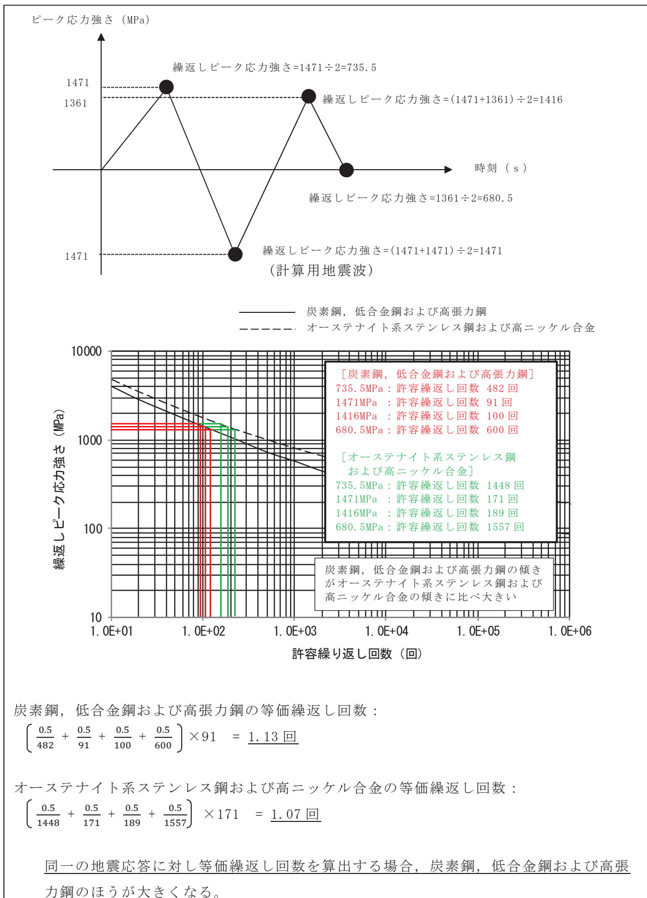
図 3-14 設計疲労線図の違いに対する等価繰返し回数の計算例
