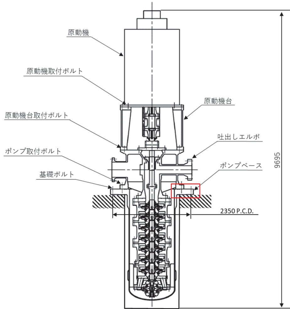
構造概要図
