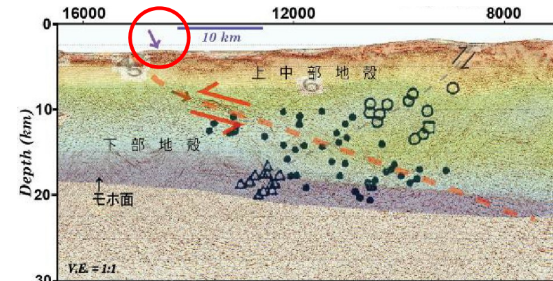
マルチチャンネル反射法地震探査によって得られた深度断面と 海底地震計による地震波速度構造と海陸統合処理によって得られた余震分布の比較 (小平(2013)に一部加筆)
