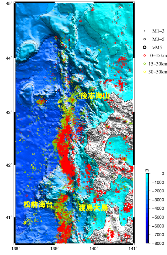
日本海東縁中部の震源分布
