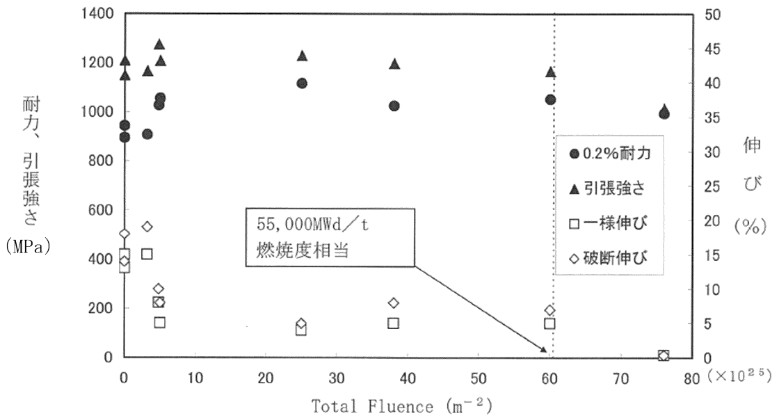
図 7-2 718 合金の照射による引張性質の変化 (35)
