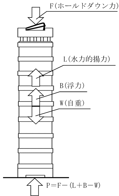
図 4-2 通常運転時荷重
