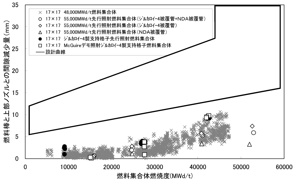
図 3-26 トータルギャップ減少量 (34)
