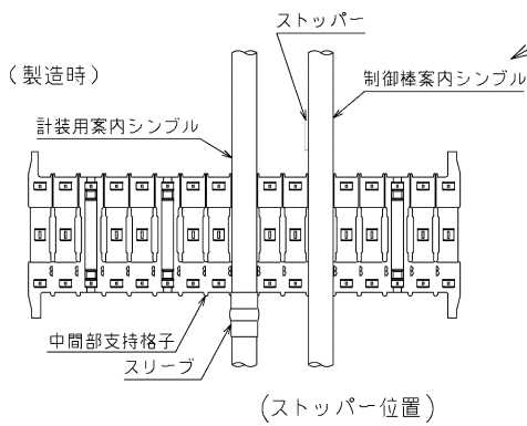
(中間部支持格子移動防止機構の概略図)
