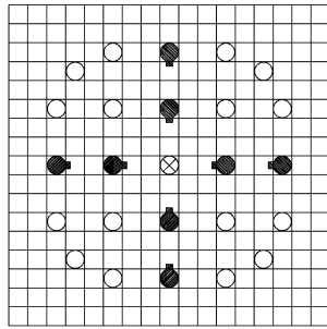
⊗ 炉内計装用案内シンプル ○ 制御棒案内シンプル ● ストッパー付き制御棒案内シンプル (支持格子内制御棒案内シンプル配置図)
