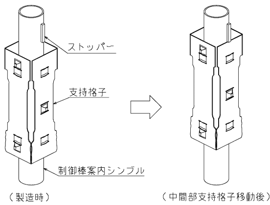
(中間部支持格子移動防止機構の概略図)
