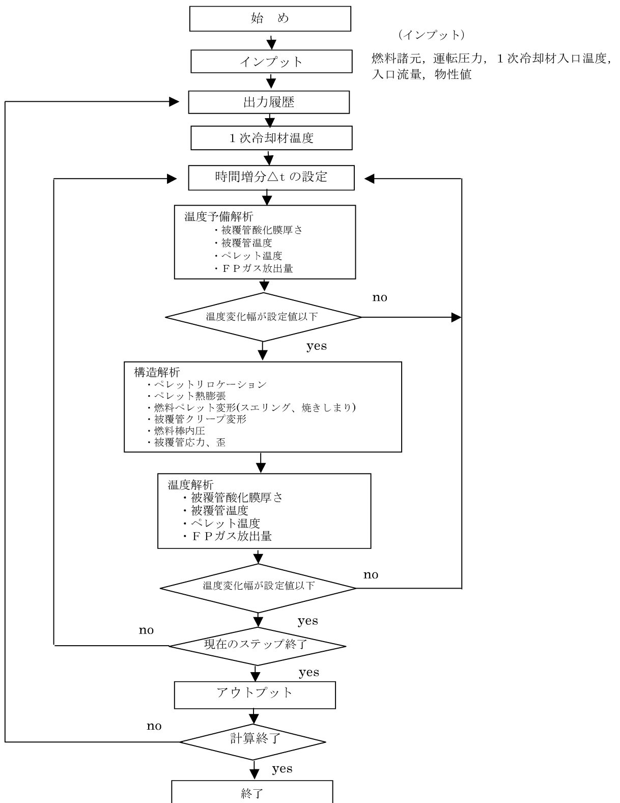
図 3-2 高燃焼度用 FPAC コードの流れ図
