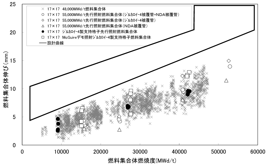
図 3-25 燃料集合体伸び (34)
