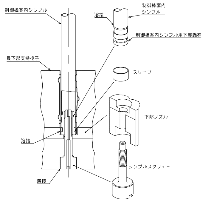
下部支持板(下部ノズル)との結合
