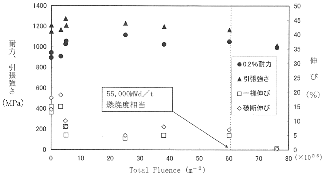
図 7-2 718 合金の照射による引張性質の変化 (35)
