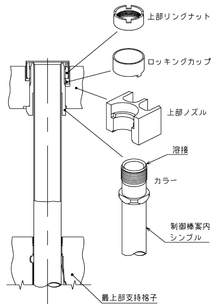
上部支持板(上部ノズル)との結合 (ストッパー付き制御棒案内シンプル)
