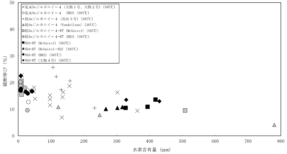
図 5-3 被覆管水素濃度と破断伸びの関係 (9) (20)
