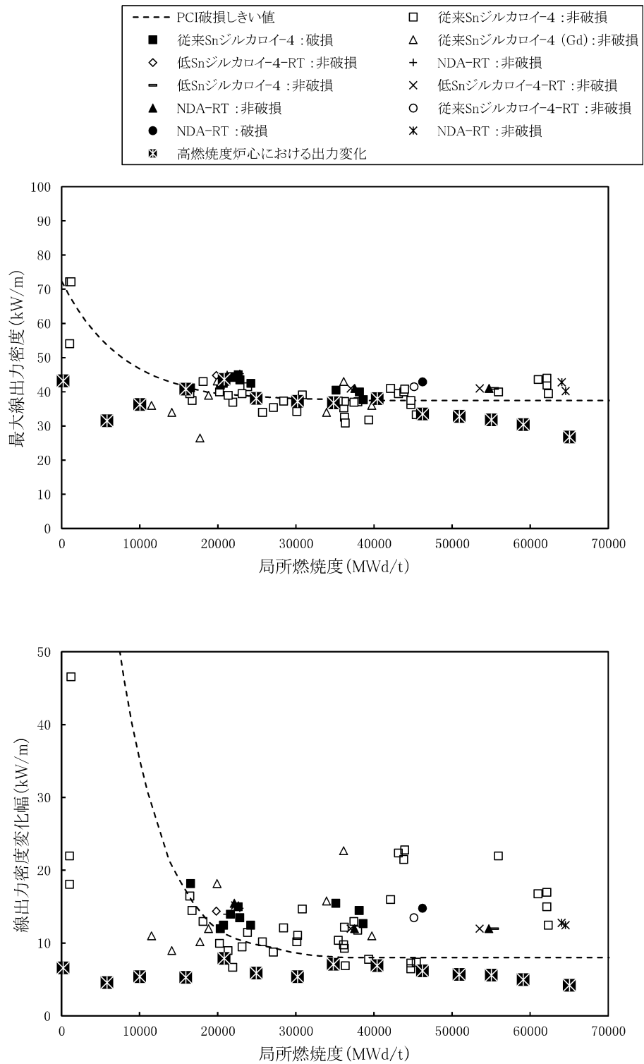
図 3-29 (1) 被覆管の出力ランプ試験結果 (最大線出力密度が最大の場合の出力変化)
