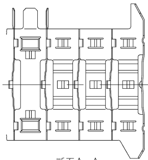
断面A-A
