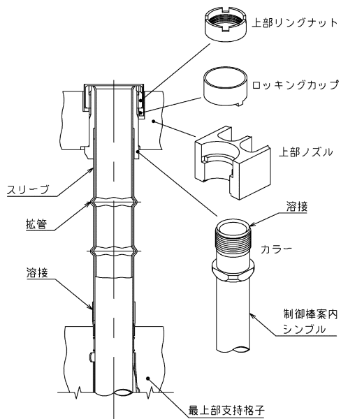
上部支持板(上部ノズル)との結合 (制御棒案内シンプル)
