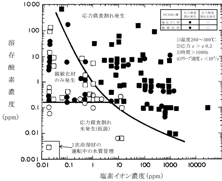
図 9-5 SUS304 鋼の応力腐食割れ発生におよぼす塩素イオン濃度及び溶存酸素濃度の限界量 (44)
