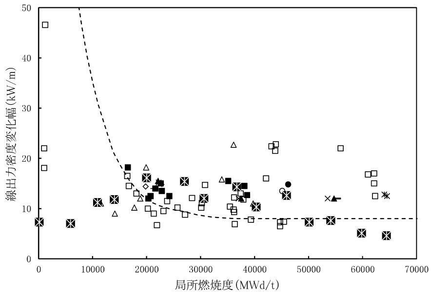
図 3-29 (2) 被覆管の出力ランプ試験結果 (線出力密度変化幅が最大の場合の出力変化)
