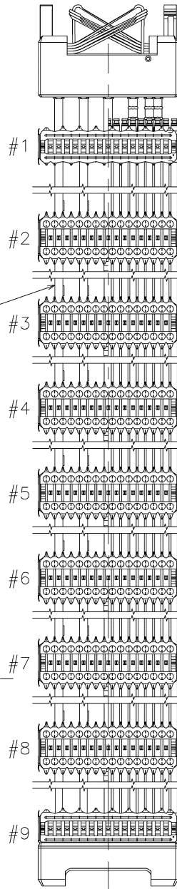
制御棒案内シムブル (ストッパー付き)
