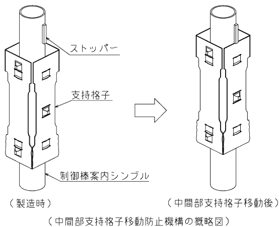
制御棒案内シムブル (ストッパー付き)
