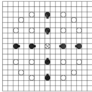
⊗ 炉内計装用案内シムブル ○ 制御棒案内シムブル ● ストッパー付き制御棒案内シムブル (支持格子内制御棒案内シムブル配置図)
