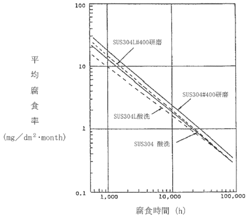
図 8-4 SUS304 鋼の溶存酸素を含まない 300°C の 0.92% ホウ酸水中における平均腐食率 (41)
