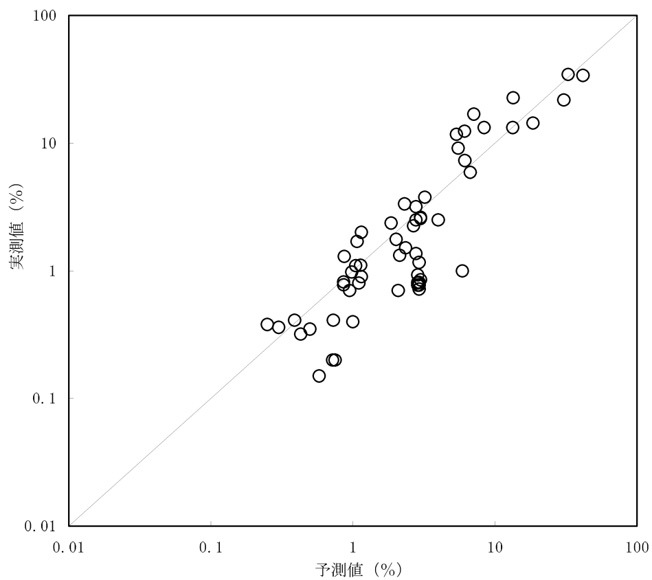
図 3-8 FP ガス放出率の計算値と実測値との比較
