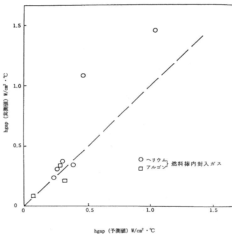
図 3-3 (2) ギャップコンダクタンス式の実測値との比較 (8)
