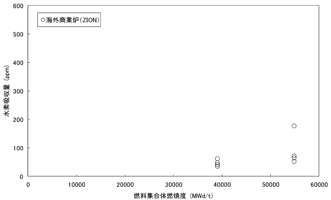
図 5-12 実機で照射された案内シンプルの水素吸収量データ (30)
