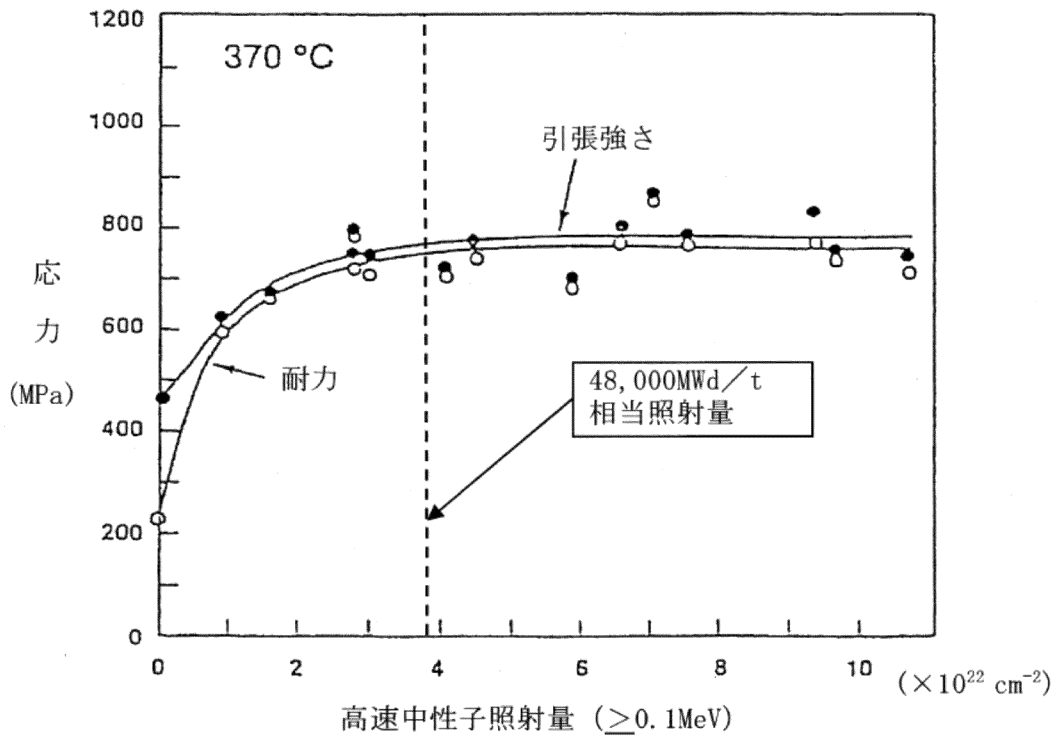
図 8-2 SUS304 鋼の照射による機械的性質の変化 (39) (照射温度 370°C、試験温度 370°C)
