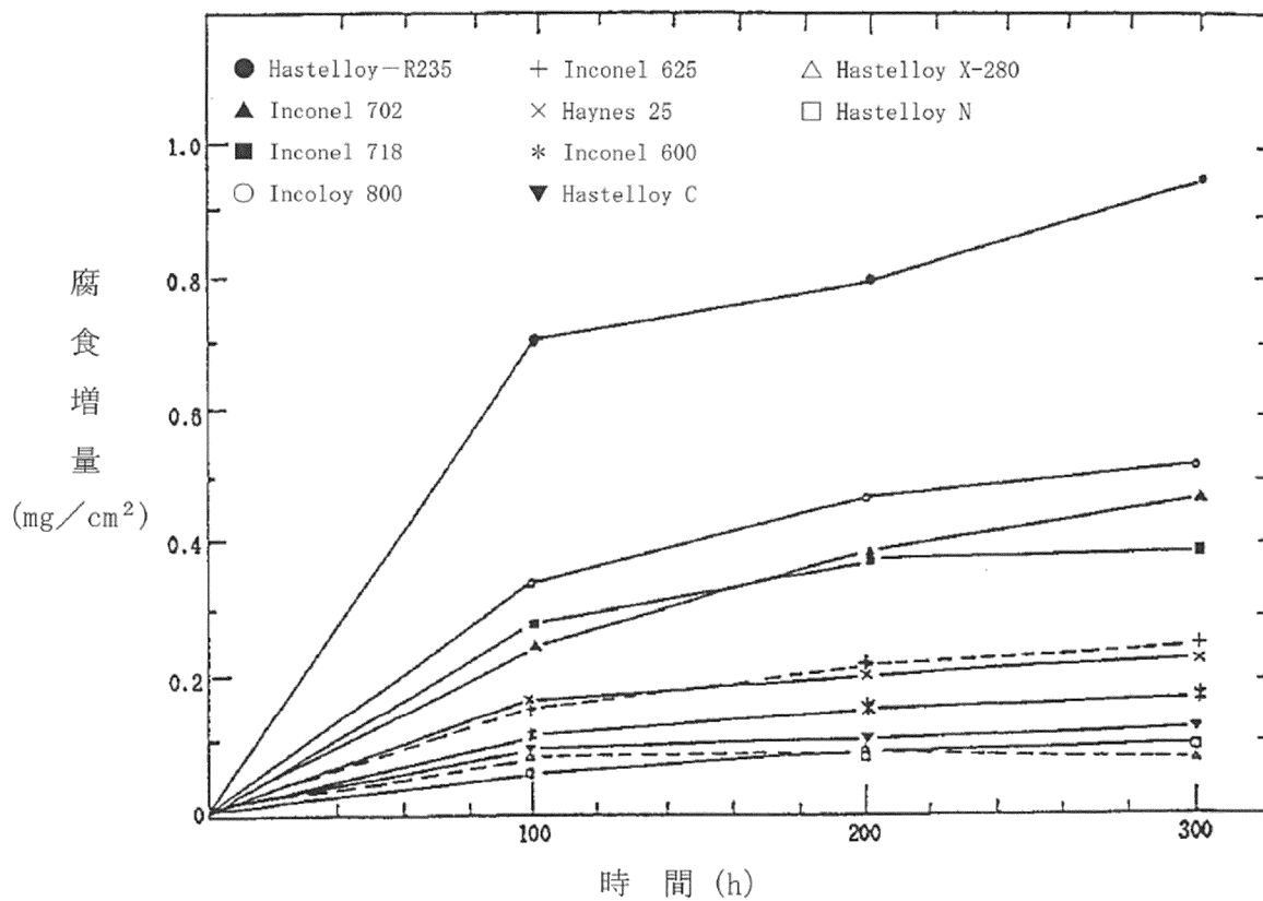
図 6-4 ニッケル基合金の腐食増量 (815°C) (35)
