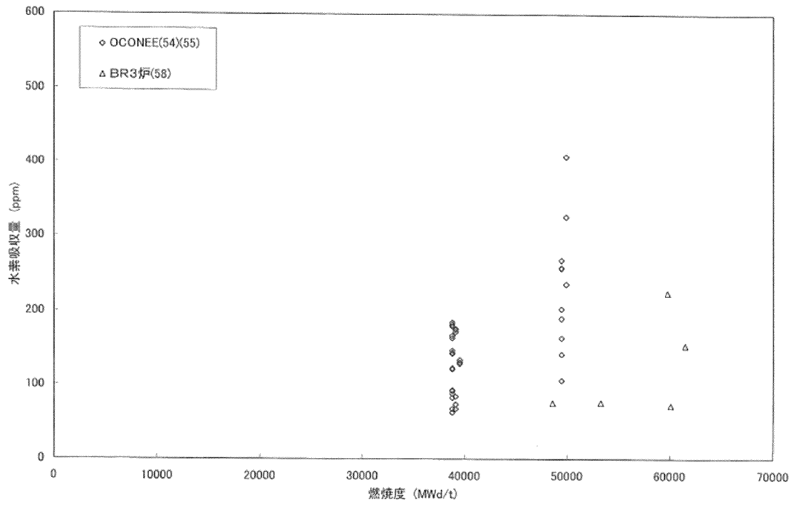
図 5-9 ジルカロイ-4 被覆管水素吸収量 (27) (28) (29)
