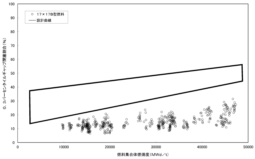
図 3-17 燃料棒間隔の閉塞割合
