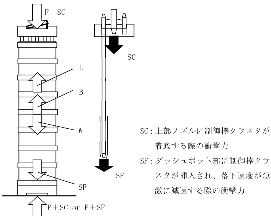
図 4-3 通常運転時及び運転時の異常な過渡変化時荷重
