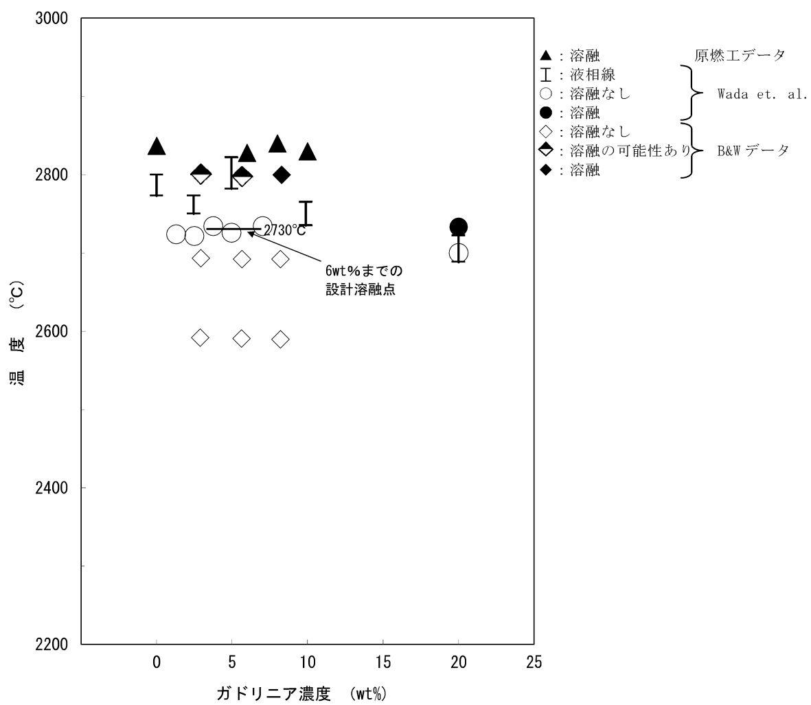
図 4-1 ガドリニア混合二酸化ウランペレットの溶融点 (17)
