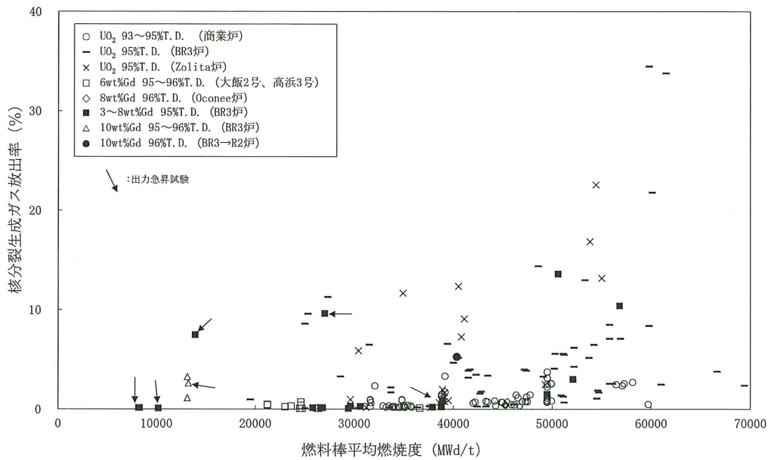
図 3-3(1) 二酸化ウランペレット及びガドリニア混合二酸化ウランペレットのFPガス放出率 (17)
