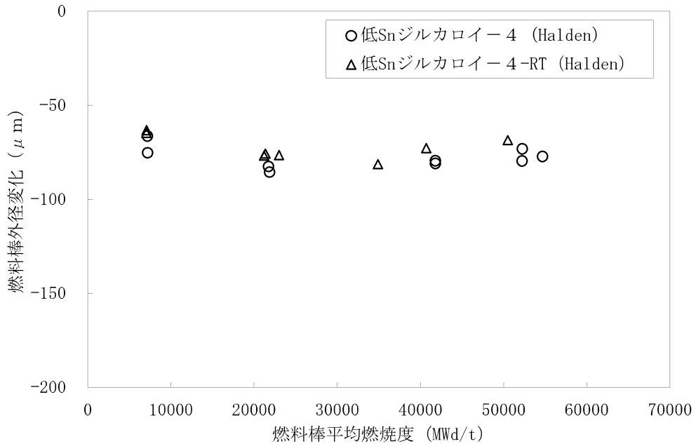
図 5-5 燃料棒外径変化 (実機照射セグメント燃料棒) (23)
