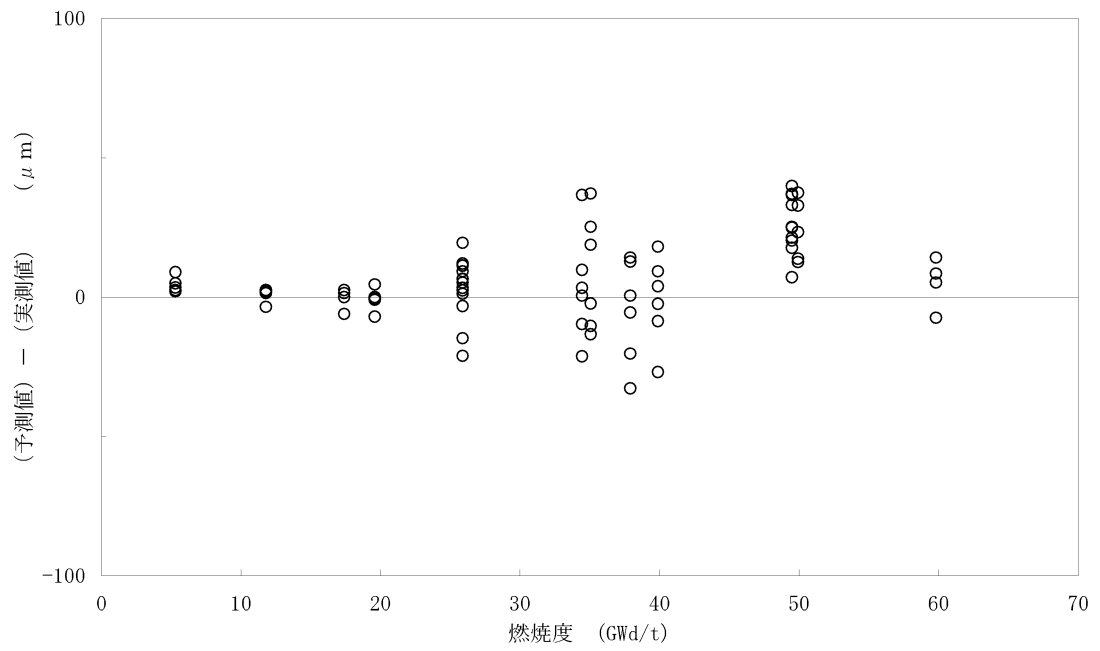
図 3-7 (3) 被覆管外径変化(内向きクリープ変形)の 予測値と実測値との差の燃焼度にもなう変化
