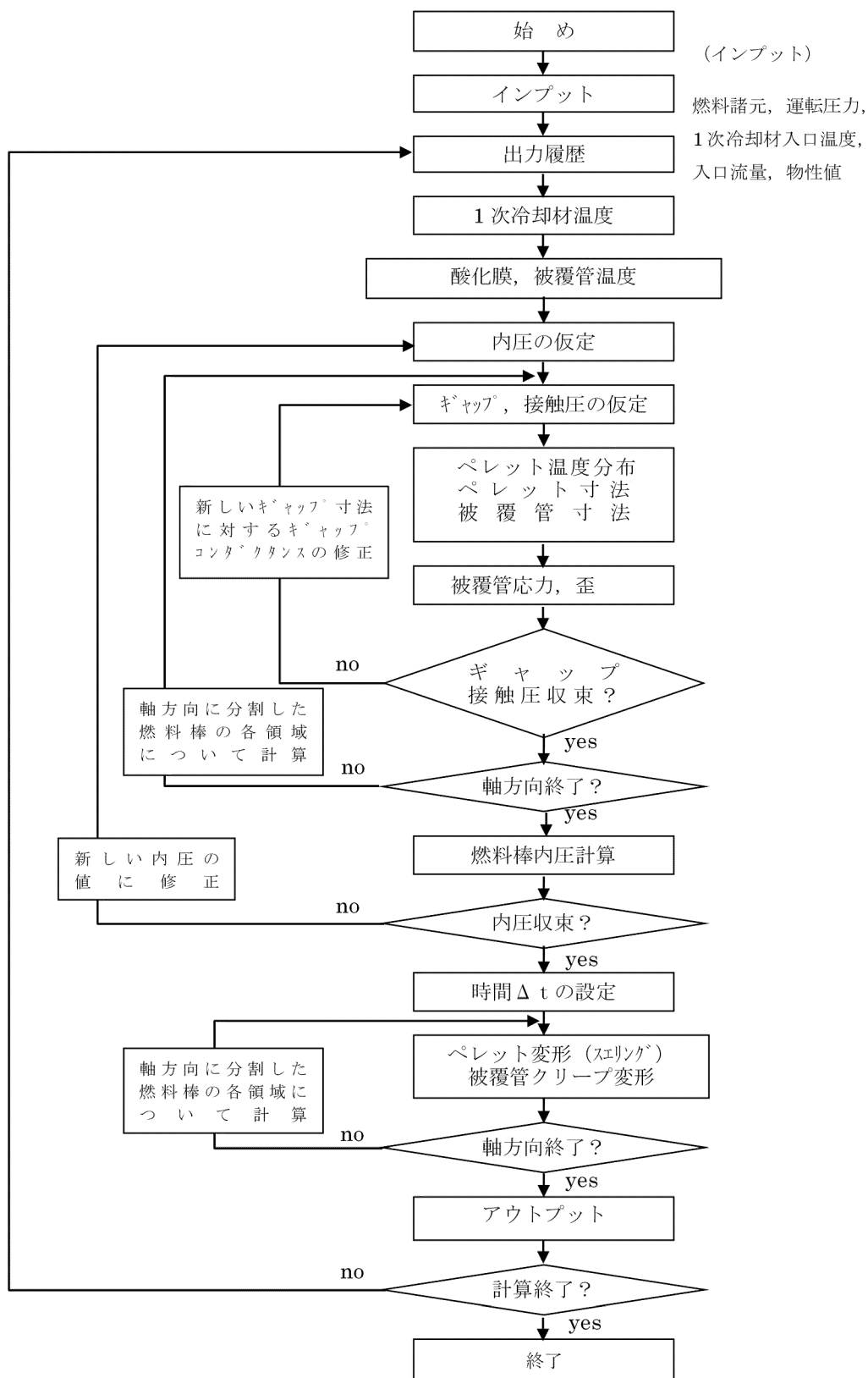
図 3-2 FPAC コードの流れ図
