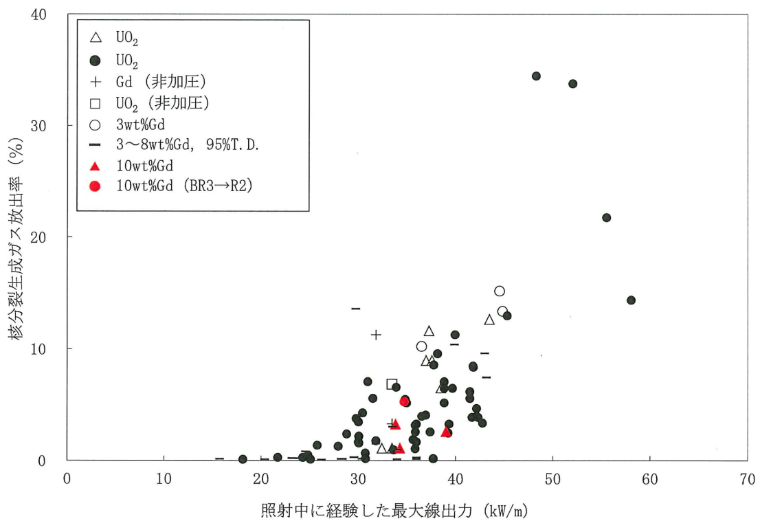
図 3-3(2) 二酸化ウランペレット及びガドリニア混合二酸化ウランペレットのFPガス放出率と線出力密度の関係 (17)
