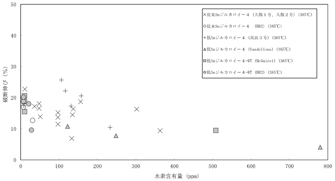
図 5-3 被覆管水素濃度と破断伸びの関係 (9) (23)
