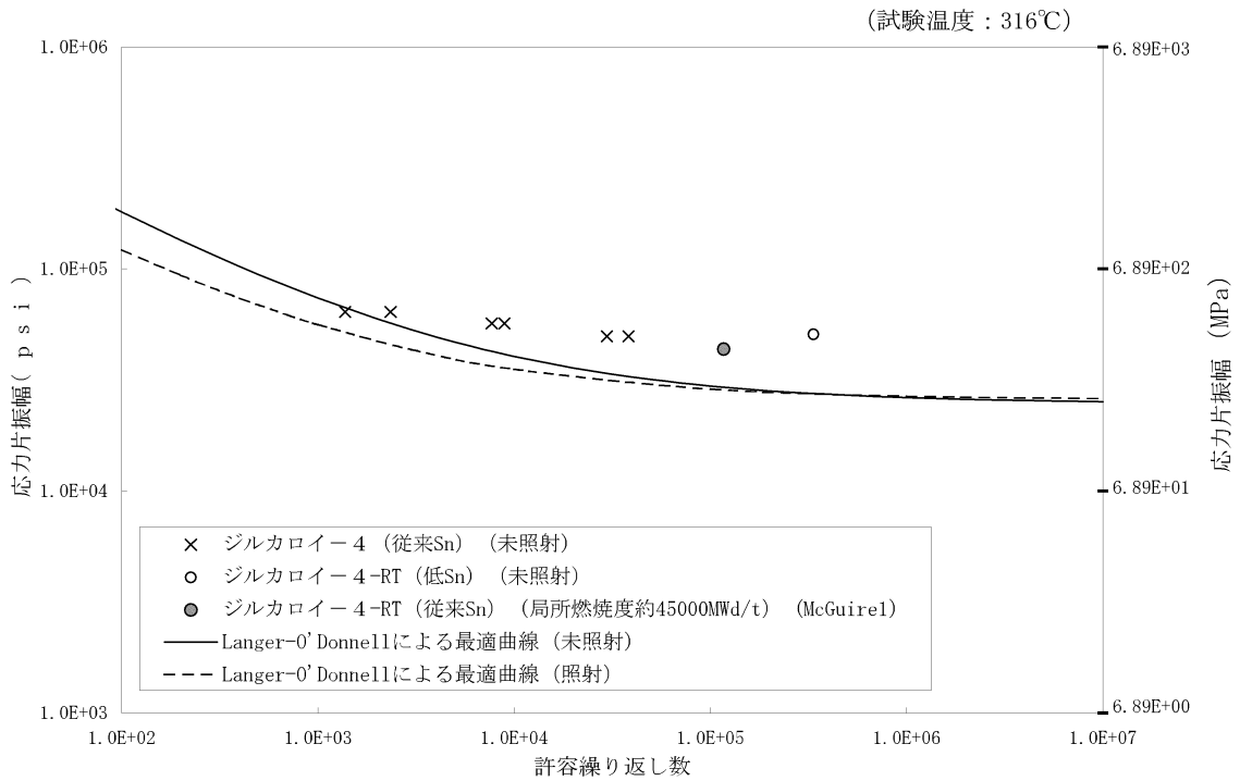
図 5-4 ジルカロイ-4 被覆管の疲労強度 (23)
