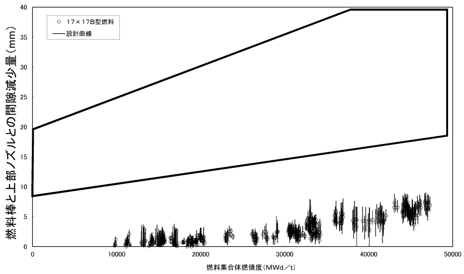
図 3-19 トータルギャップ減少量
