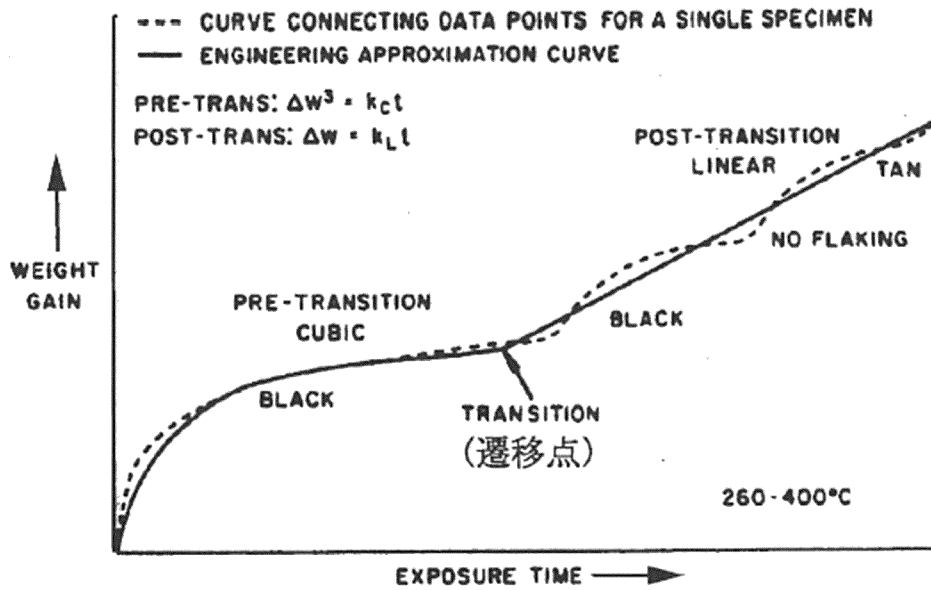
図 5-7 炉外腐食試験におけるジルカロイ-2 とジルカロイ-4 の典型的な腐食増量曲線 (26)
