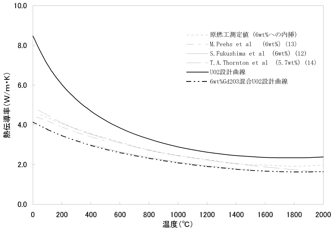
図 3-4 (2) ガドリニア混合二酸化ウランの熱伝導率 (95%T.D.) (12) (17) (18)
