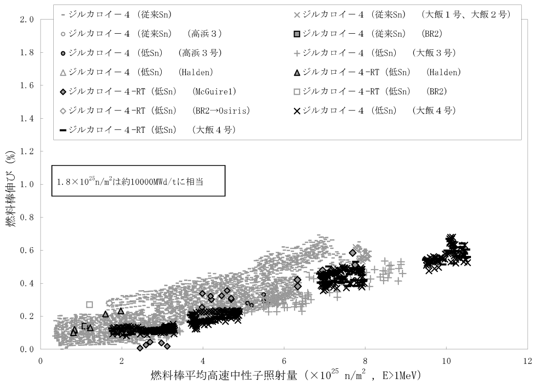
図 5-6 ジルカロイ-4 被覆管の照射成長 (23)
