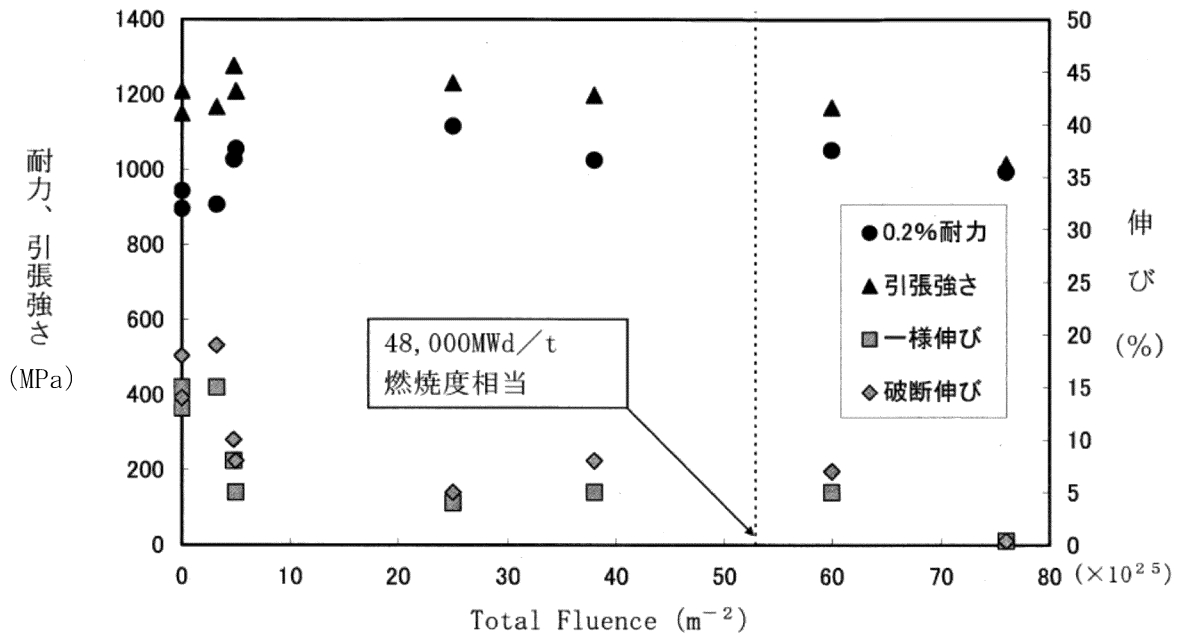
図 6-2 718 合金の照射による引張性質の変化 (33)
