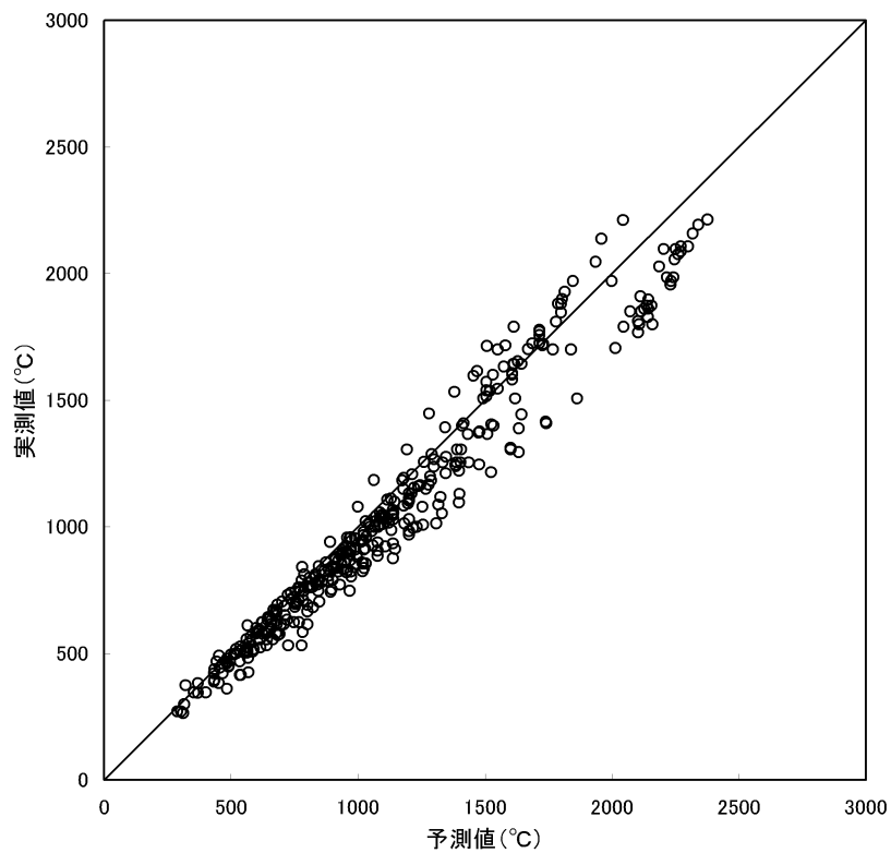
図 3-6 燃料中心温度の計算値と実測値との比較
