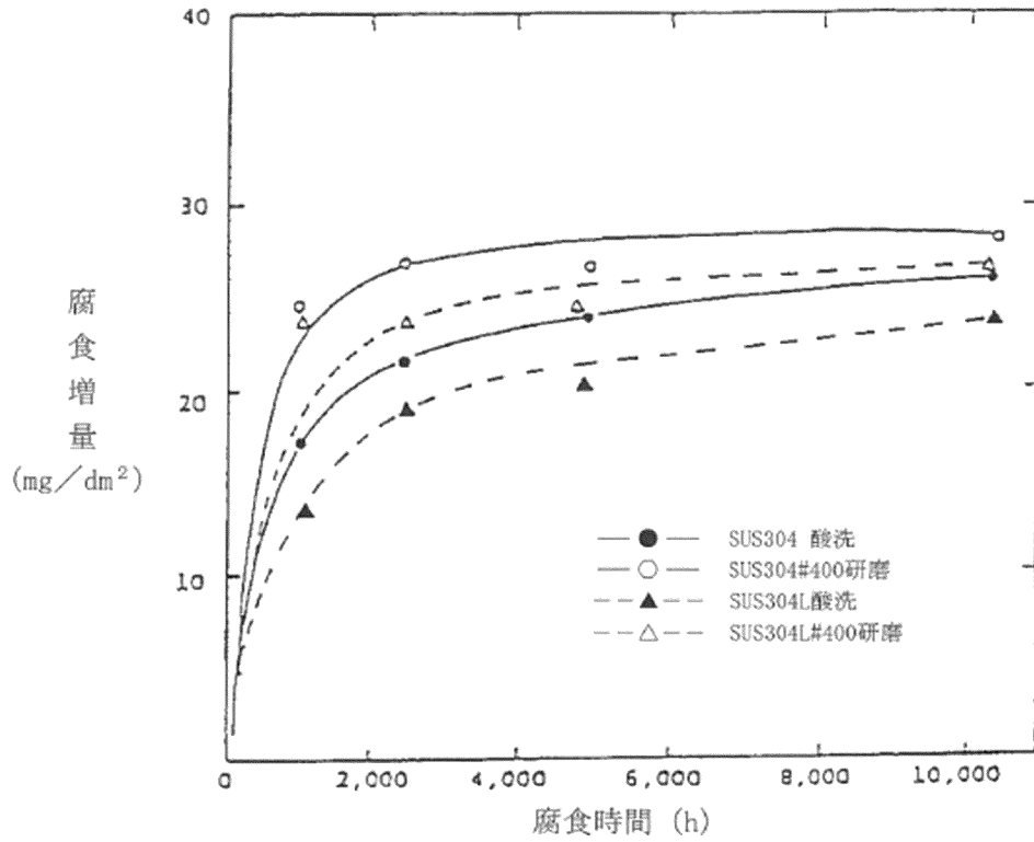
図 8-3 SUS304 鋼の高温水中腐食 (試験温度 300°C) (41)
