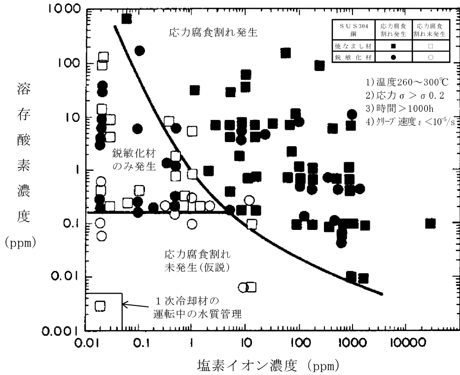
図 8-5 SUS304 鋼の応力腐食割れ発生におよぼす塩素イオン濃度及び溶存酸素濃度の限界量 (42)
