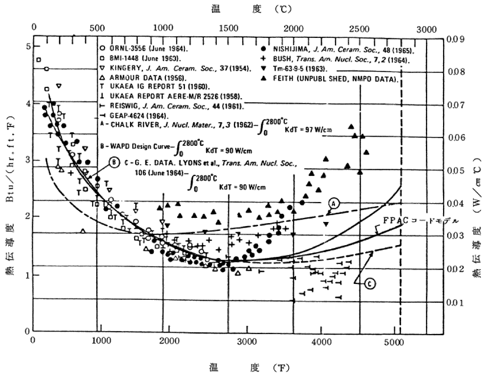
図 3-4 (1) 二酸化ウランペレットの熱伝導率 (95%T.D.) (16)
