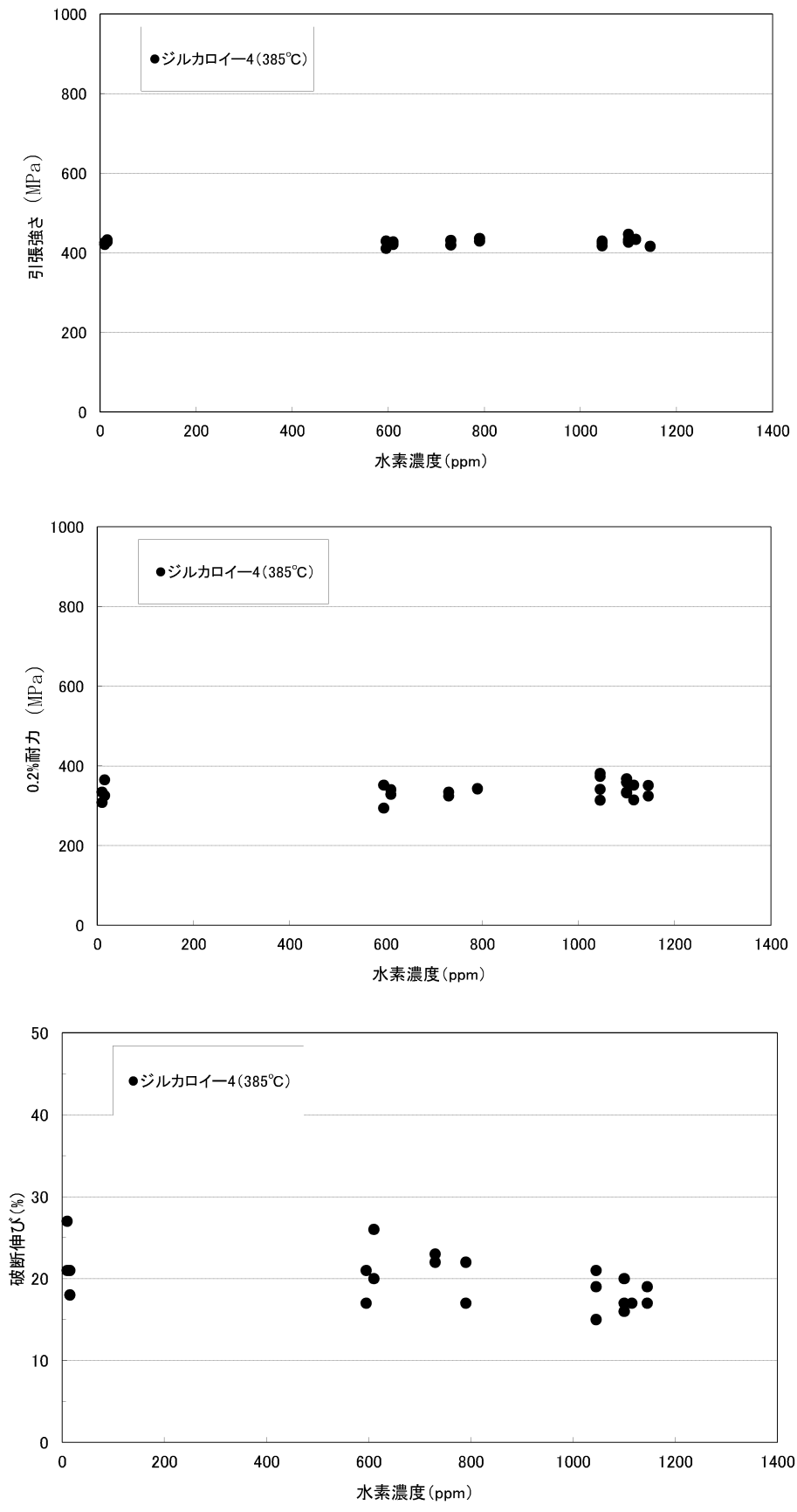
図 5-2 ジルカローイ-4 未照射被覆管の機械特性と水素濃度の関係 (23)
