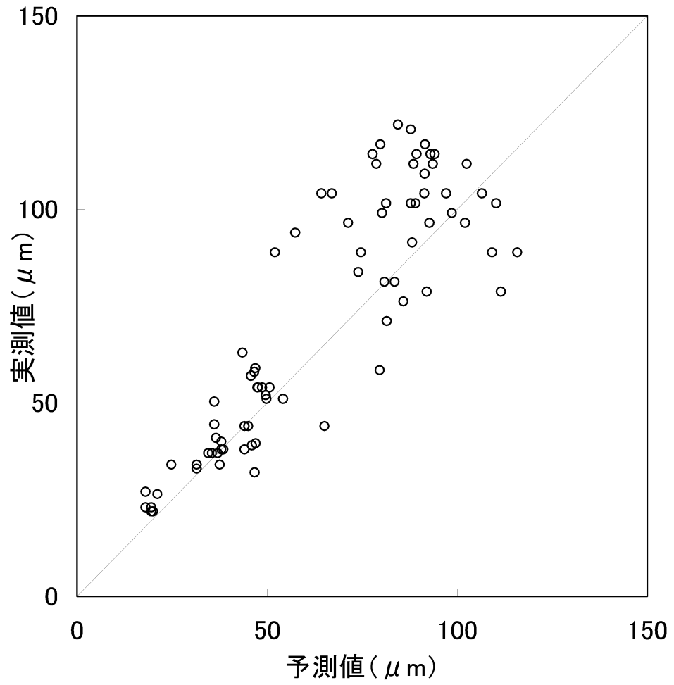
図 3-7 (5) 被覆管外径変化(内向きクリープ変形)に対する予測値と実測値との比較
