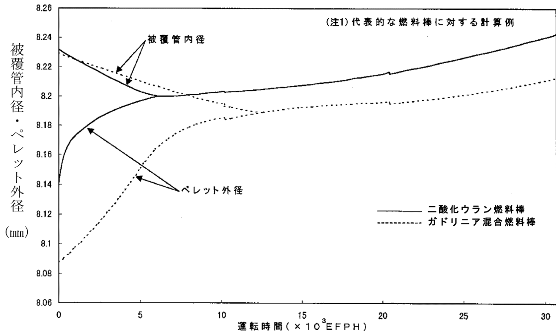
図 3-13 被覆管内径及びペレット外径変化
