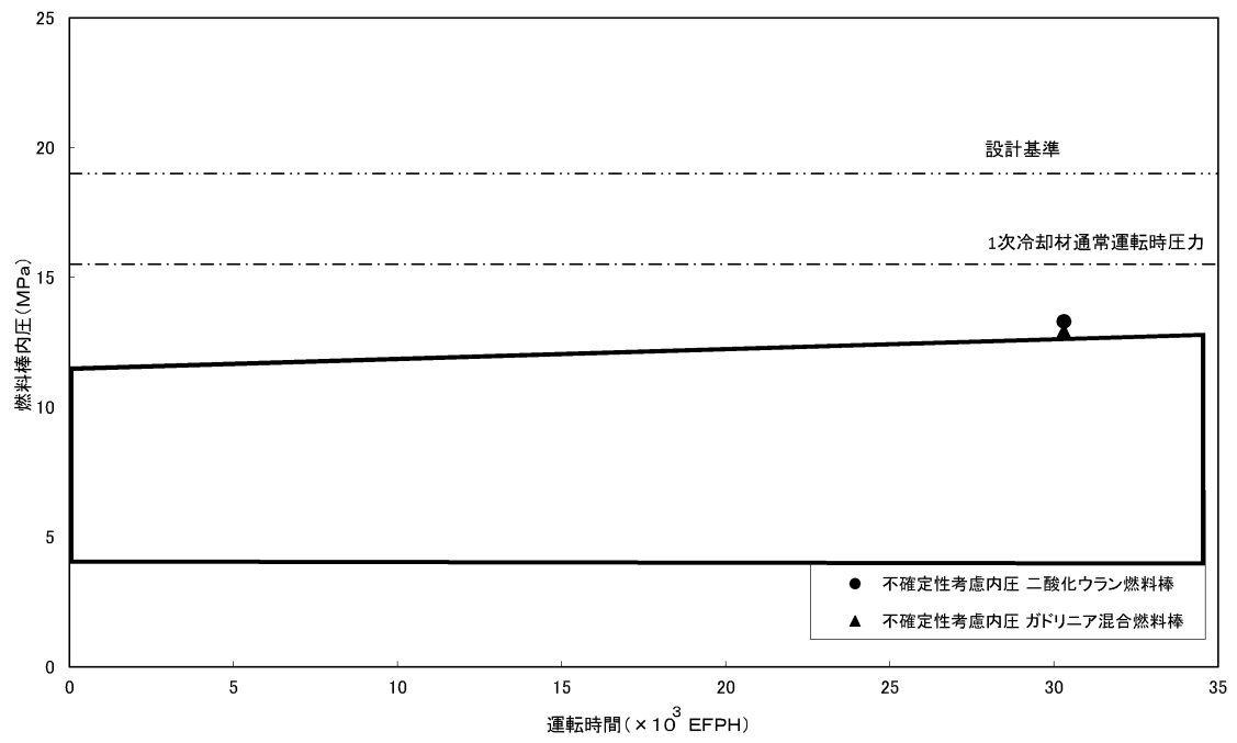
図 3-12 内圧評価上で最も厳しくなる燃料棒の内圧履歴（通常運転時）
