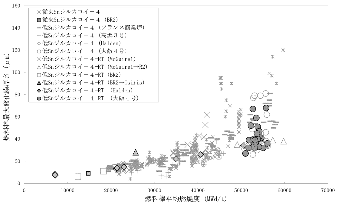
図 5-8 ジルカロイ-4 被覆管の炉内酸化膜厚さ (23)
