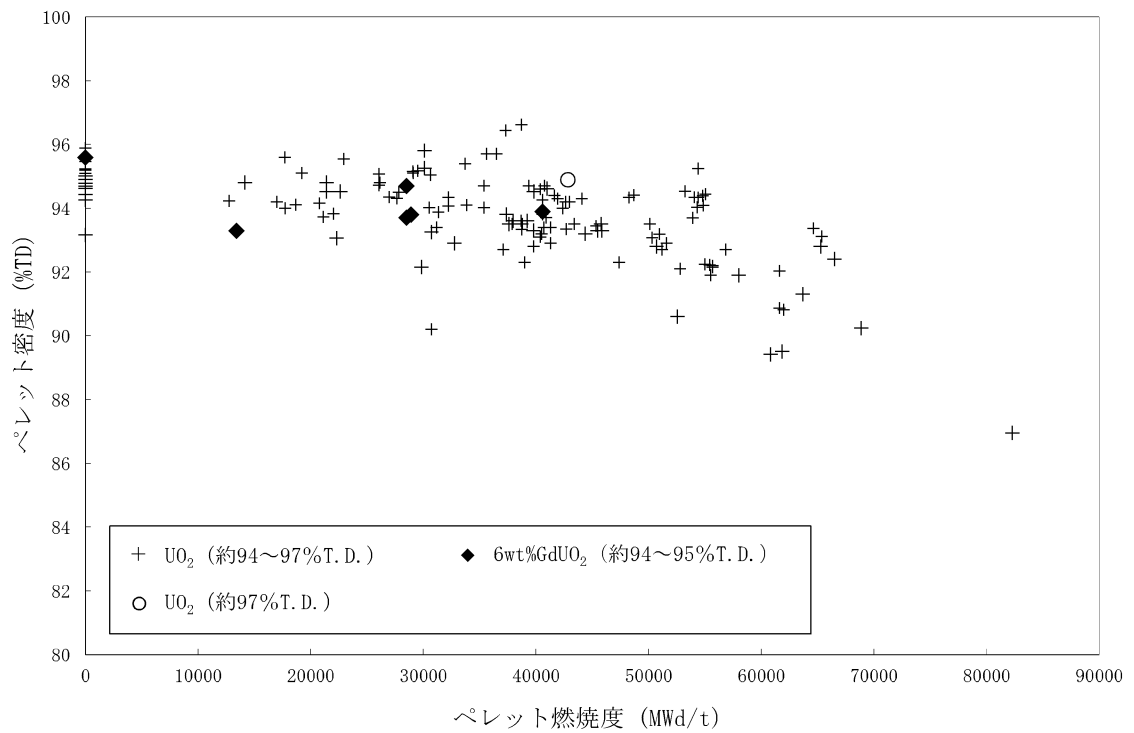
図 3-2 ペレット密度の燃焼に伴う変化 (17)
