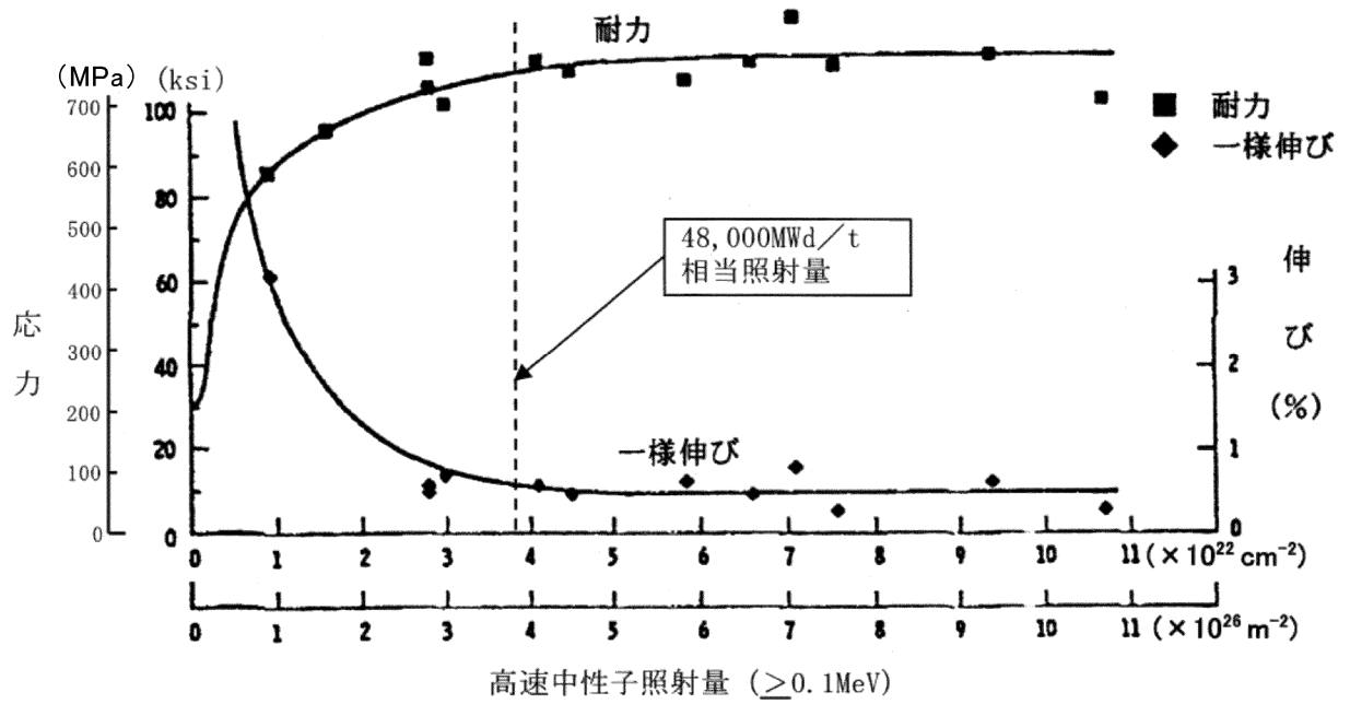
図 8-1 SUS304 鋼の照射による機械的性質の変化 (39) (照射温度 370°C、試験温度 370°C)
