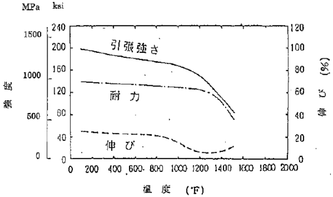
図 6-1 の温度による機械的性質の変化 (32)
