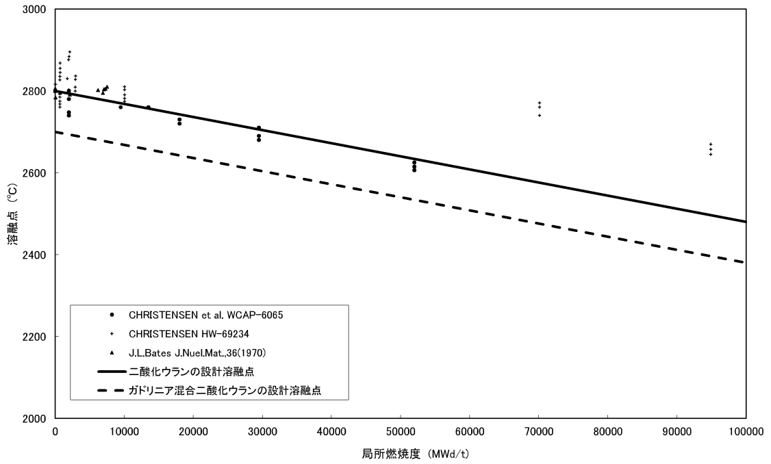
図 3-1 二酸化ウラン及びガドリニア混合二酸化ウランの溶融点 (14) (15) (16)
