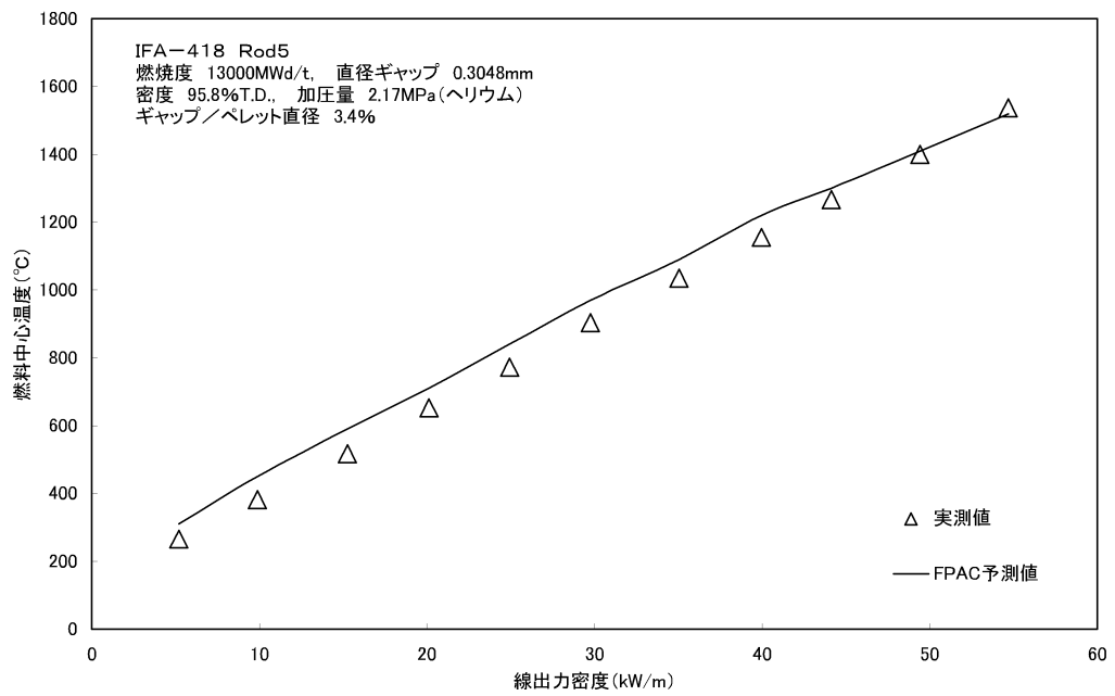
図 3-5 (1) 燃料温度の予測値と実測値との比較
