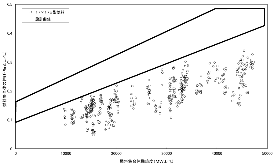
図 3-18 燃料集合体の伸び
