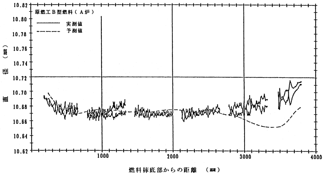
図 3-7 (2) 外径測定結果及び予測
