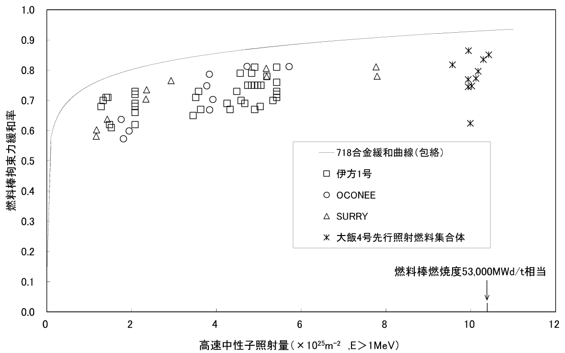
図 3-20 支持格子拘束力の緩和率実測データ
