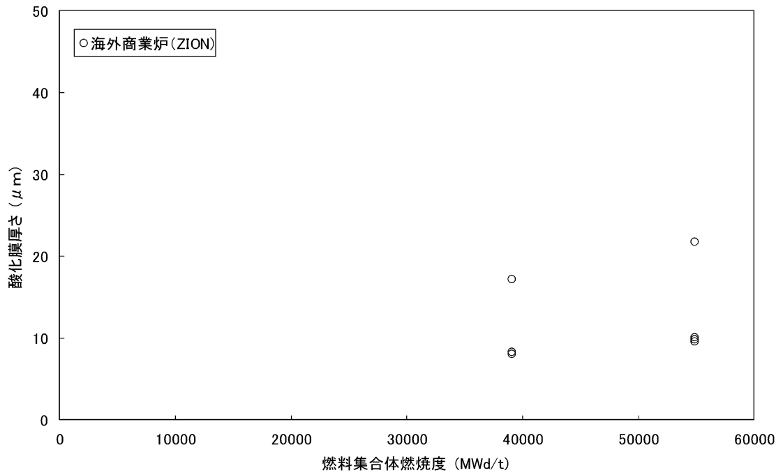
図 5-11 実機で照射された案内シンプルの腐食データ (30)
