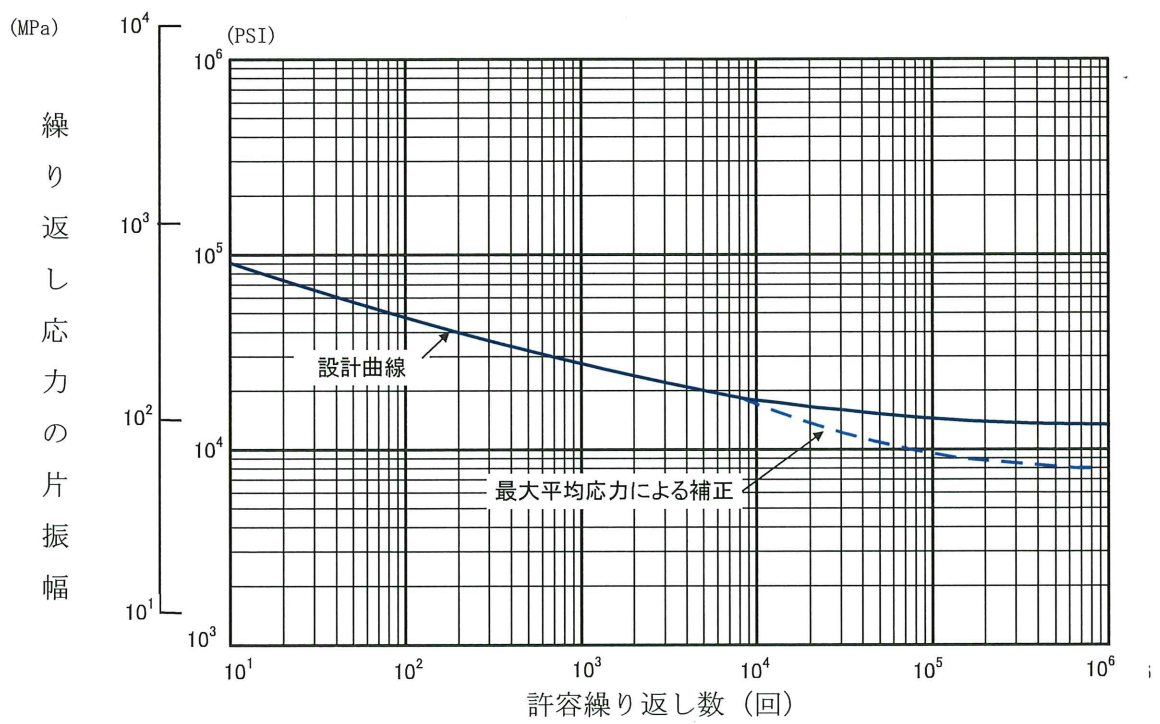
図 3-16 ジルカロイ-4 の設計疲労曲線 (29)
