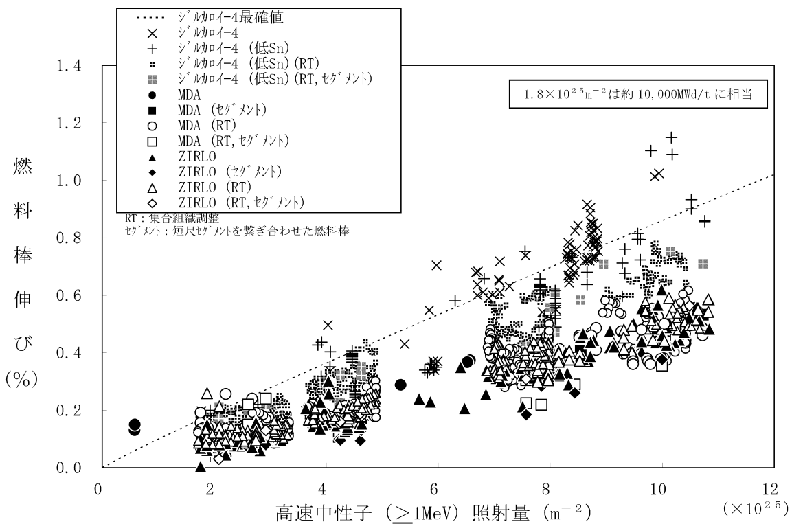
図 5-6 MDA 及び ZIRLO 被覆管の照射成長 (12)、(14)、(19)、(47) ~ (52)
