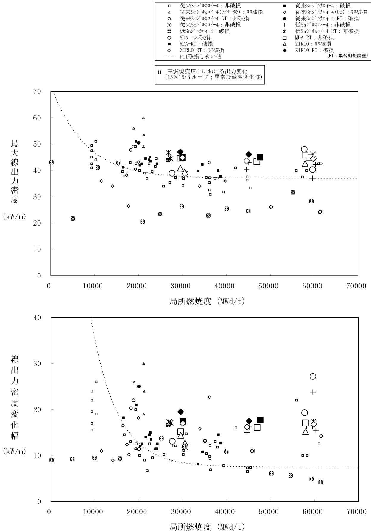
図 3-36 (2) 被覆管の出カランプ試験結果 (9)、(11)、(46)、(53)
