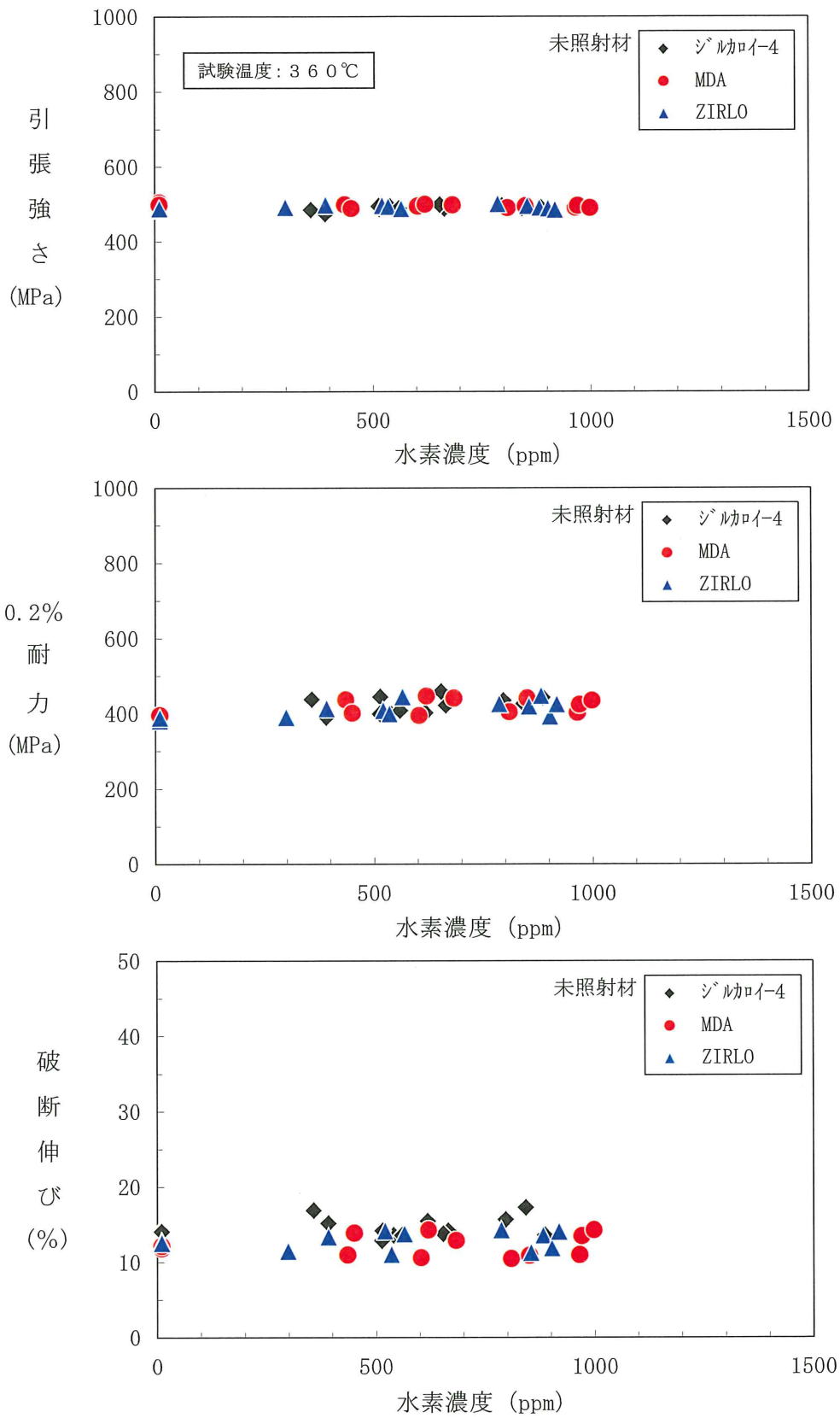
図 5-2 未照射被覆管の機械的特性と水素濃度の関係 (40)
