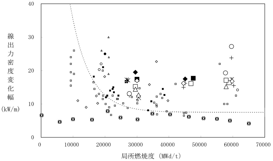
図 3-36 (1) 被覆管の出力ランプ試験結果 (9)、(11)、(46)、(57) (最大線出力密度が最大の場合の出力変化)
