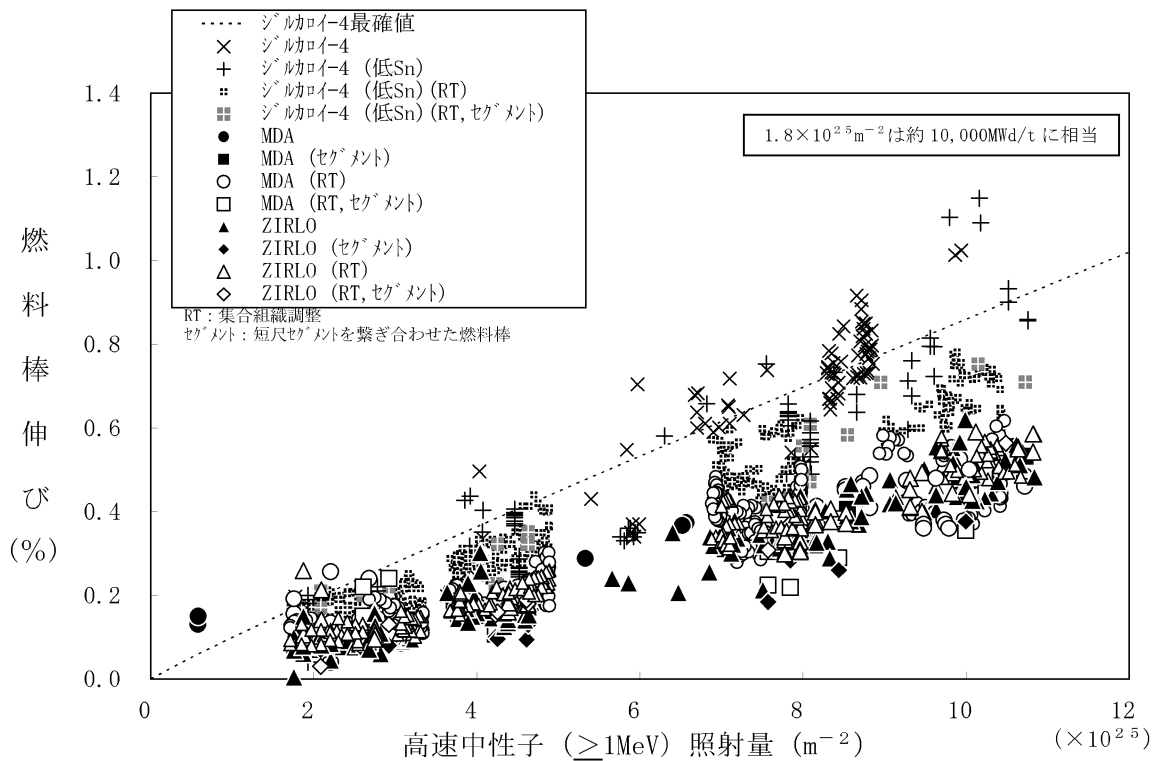
図 5-6 MDA 及び ZIRLO 被覆管の照射成長 (12)、(14)、(19)、(17) ~ (52)
