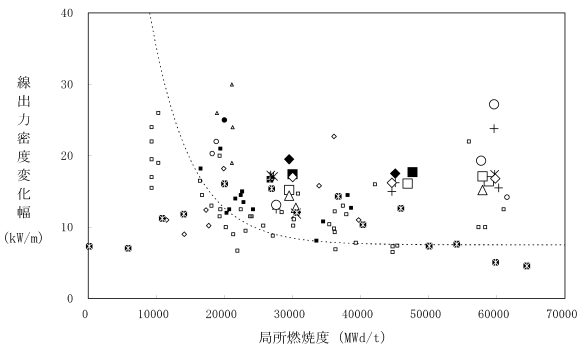
図 3-36 (2) 被覆管の出力ランプ試験結果 (9)、(11)、(16)、(57) (線出力密度変化幅が最大の場合の出力変化)
