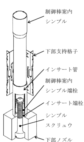
(c) 制御棒案内シンプル と下部ノズル及び 下部支持格子の結合
