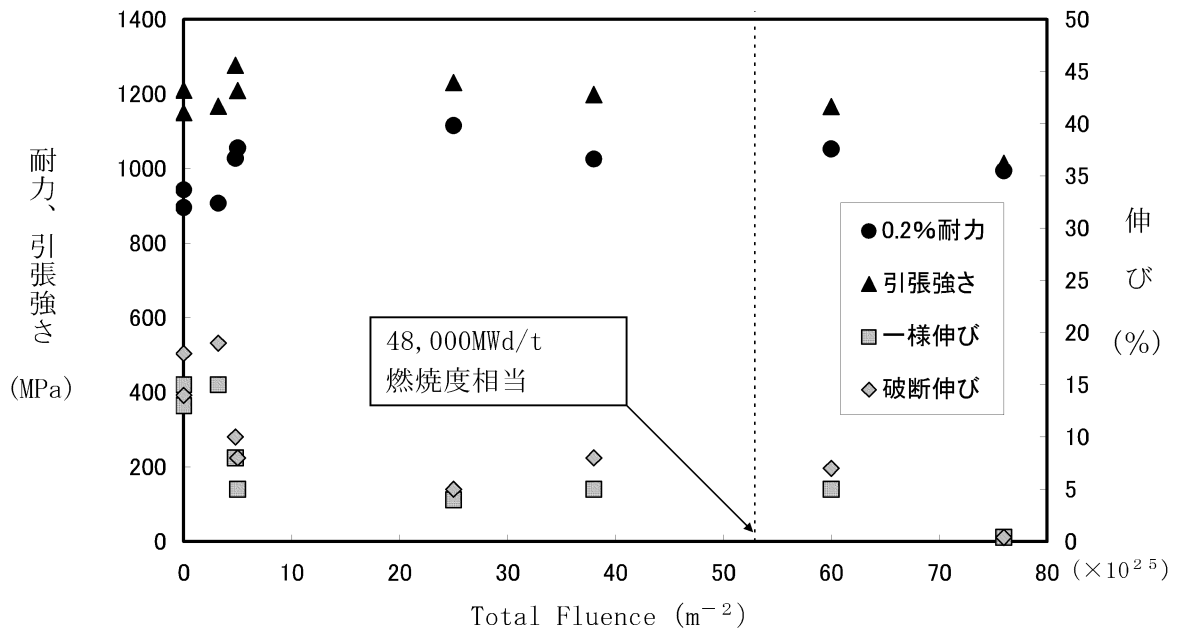
図 6-1 718 合金の照射による引張性質の変化 (56)
