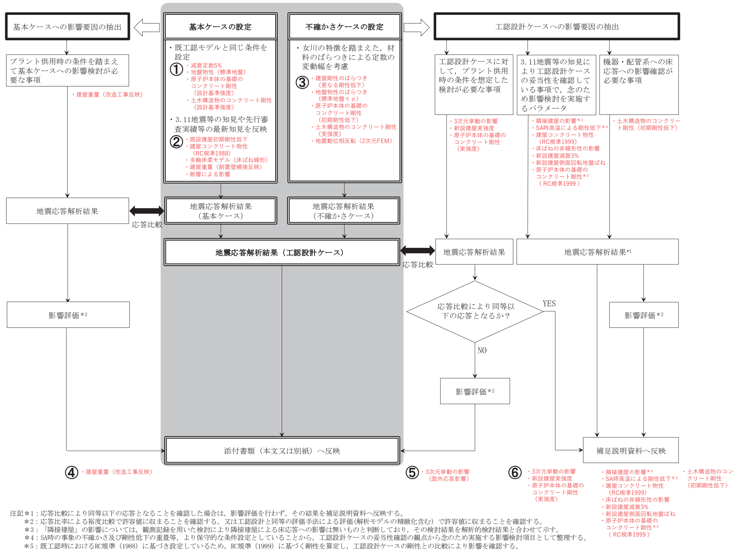
図1 女川2号機における地震応答に影響を及ぼす要因の抽出と今回工認における申請上の位置付けの整理フロー
