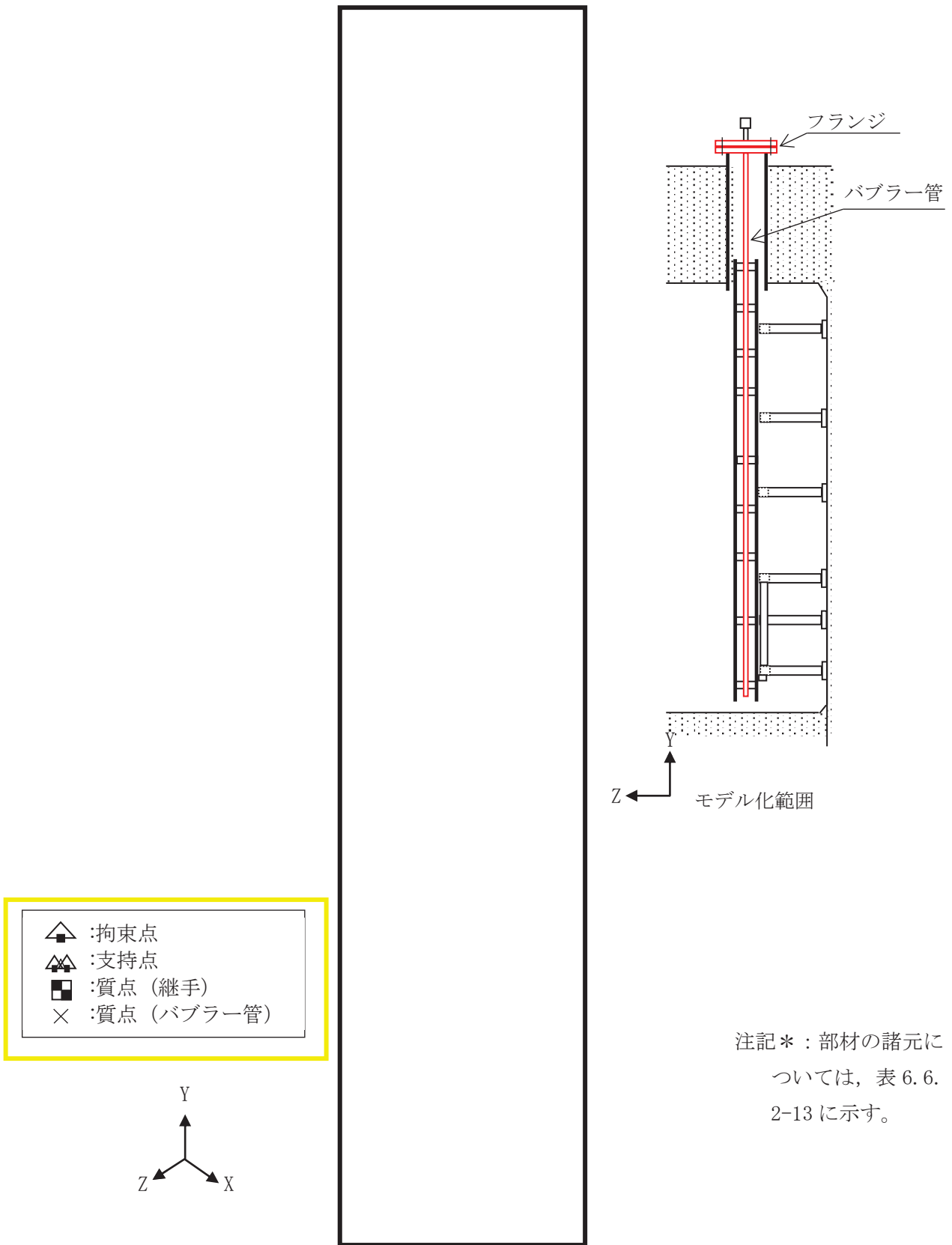
図 6. 6. 2-21 解析モデル (取水ピット水位)
