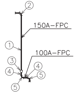
A~A矢视图
