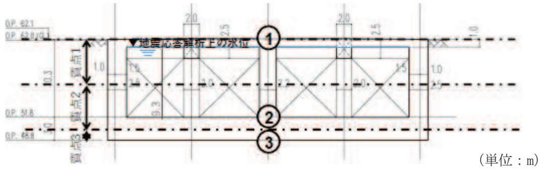
図 1-8(1) 淡水貯水槽の概略断面図 (NS 方向)
