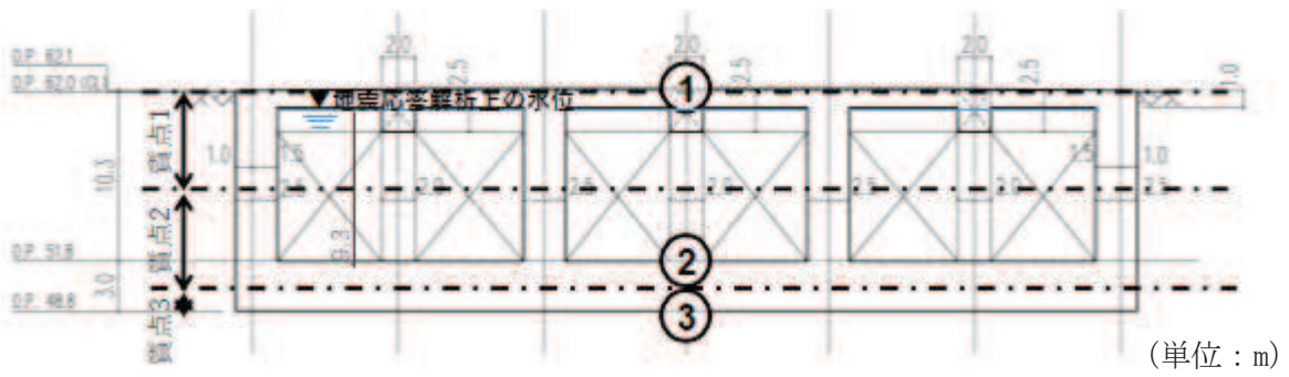
図 1-8(2) 淡水貯水槽の概略断面図 (EW 方向)
