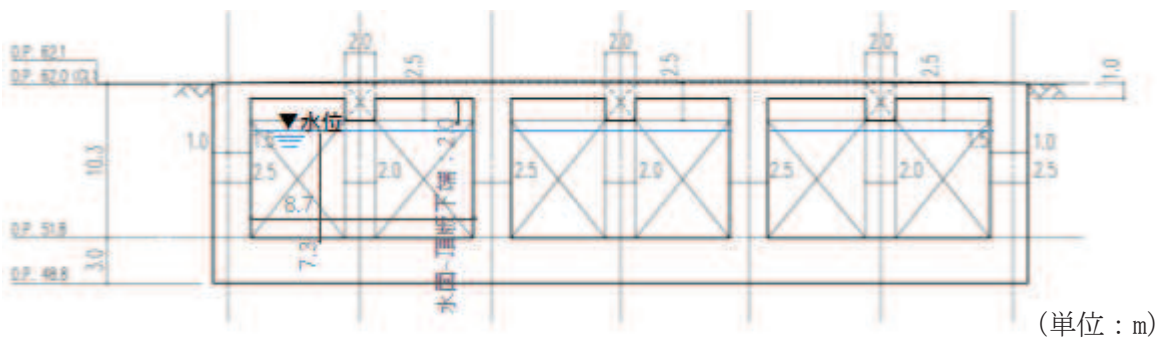
図 2-5 (2) スロッシングの振動方向長さ及び水深 (NS 方向)
