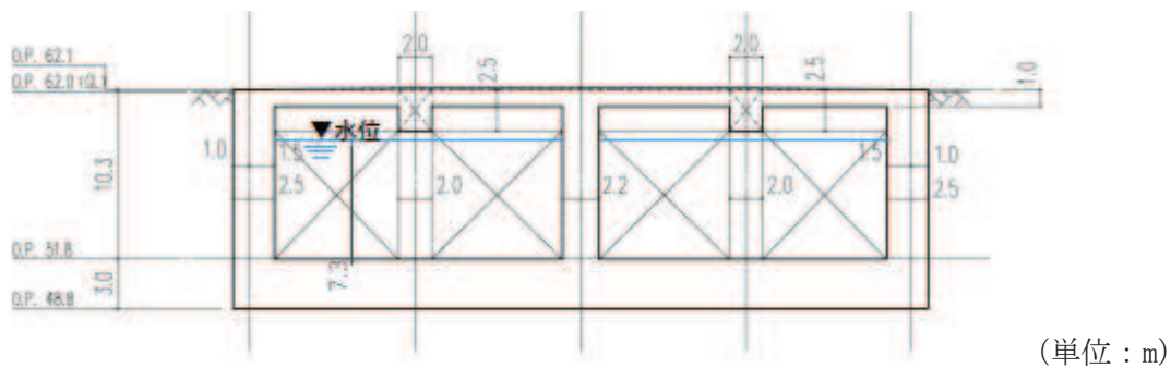
図 1-3(1) 淡水貯水槽の概略断面図 (A-A 断面 EW 方向)
