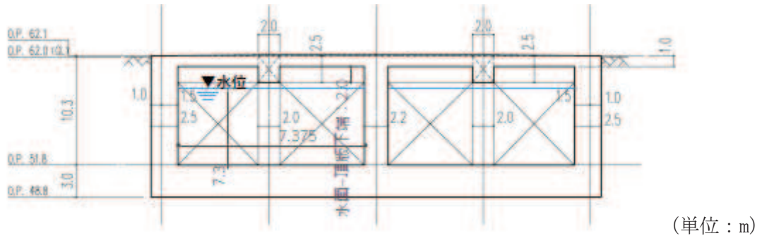
図 2-5 (1) スロッシングの振動方向長さ及び水深 (EW 方向)
