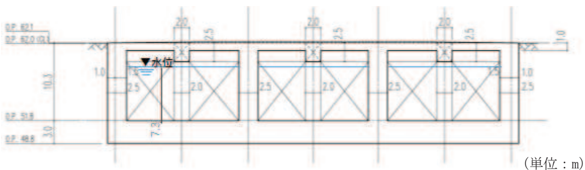
図 1-3(2) 淡水貯水槽の概略断面図 (B-B 断面 NS 方向)
