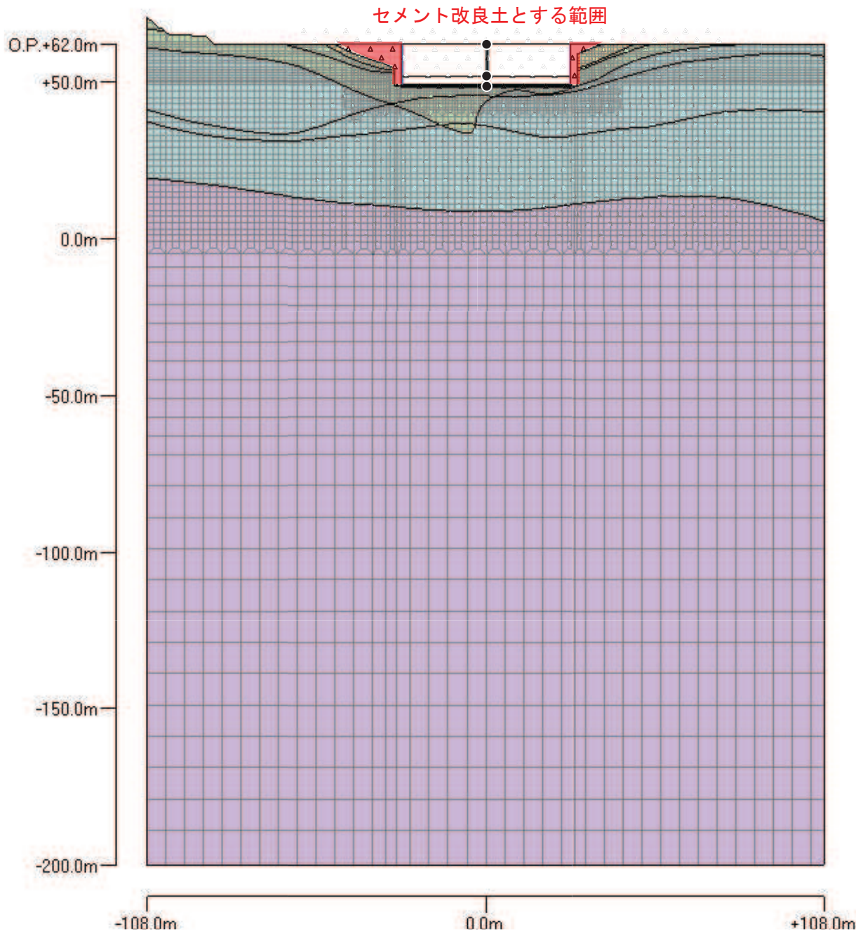
図 3-1(2) 第2 保管エリアの地震応答解析モデル (二次元)
