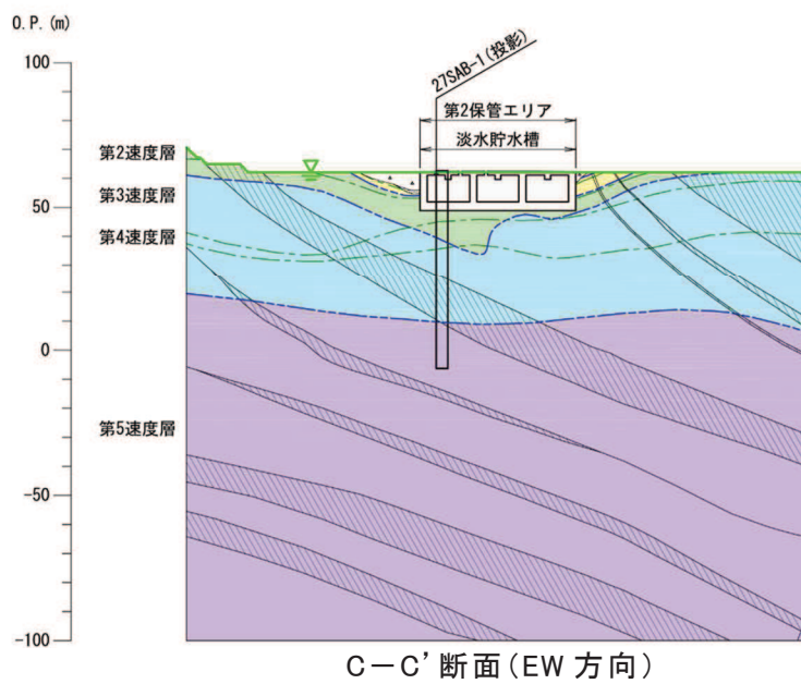
図 2.3.3-3 第 2 保管エリアの地質断面図
