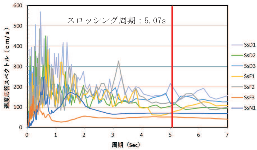
(a) ケース 1 (標準地盤 NS 方向)
