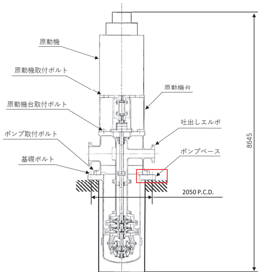
構造概要図
