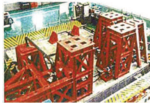
実規模配管系試験装置
