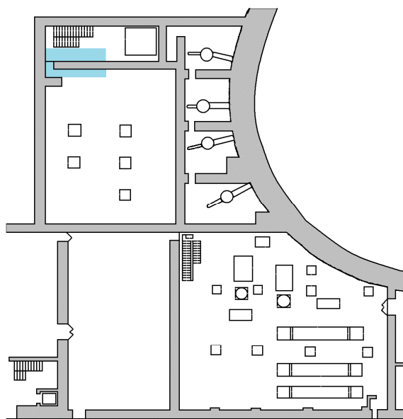
原子炉補助建屋 E L. 5. 3 m
