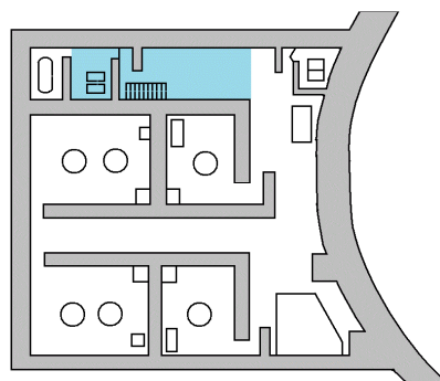
原子炉補助建屋 E L. - 1. 6 m
