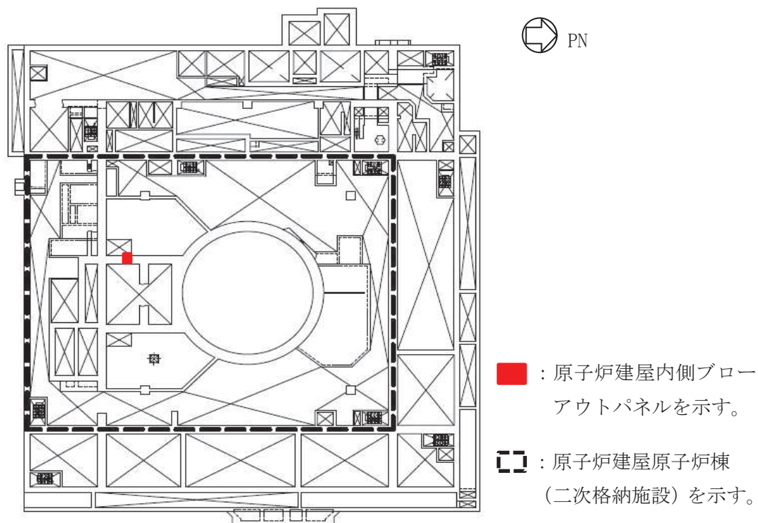
原子炉建屋原子炉棟中地下 1 階 概略平面図(0.P. 11.50m)
