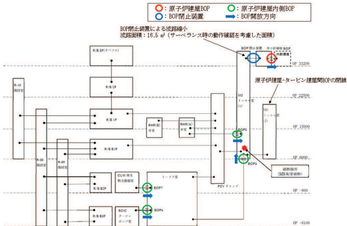
図 2-1 解析モデル
