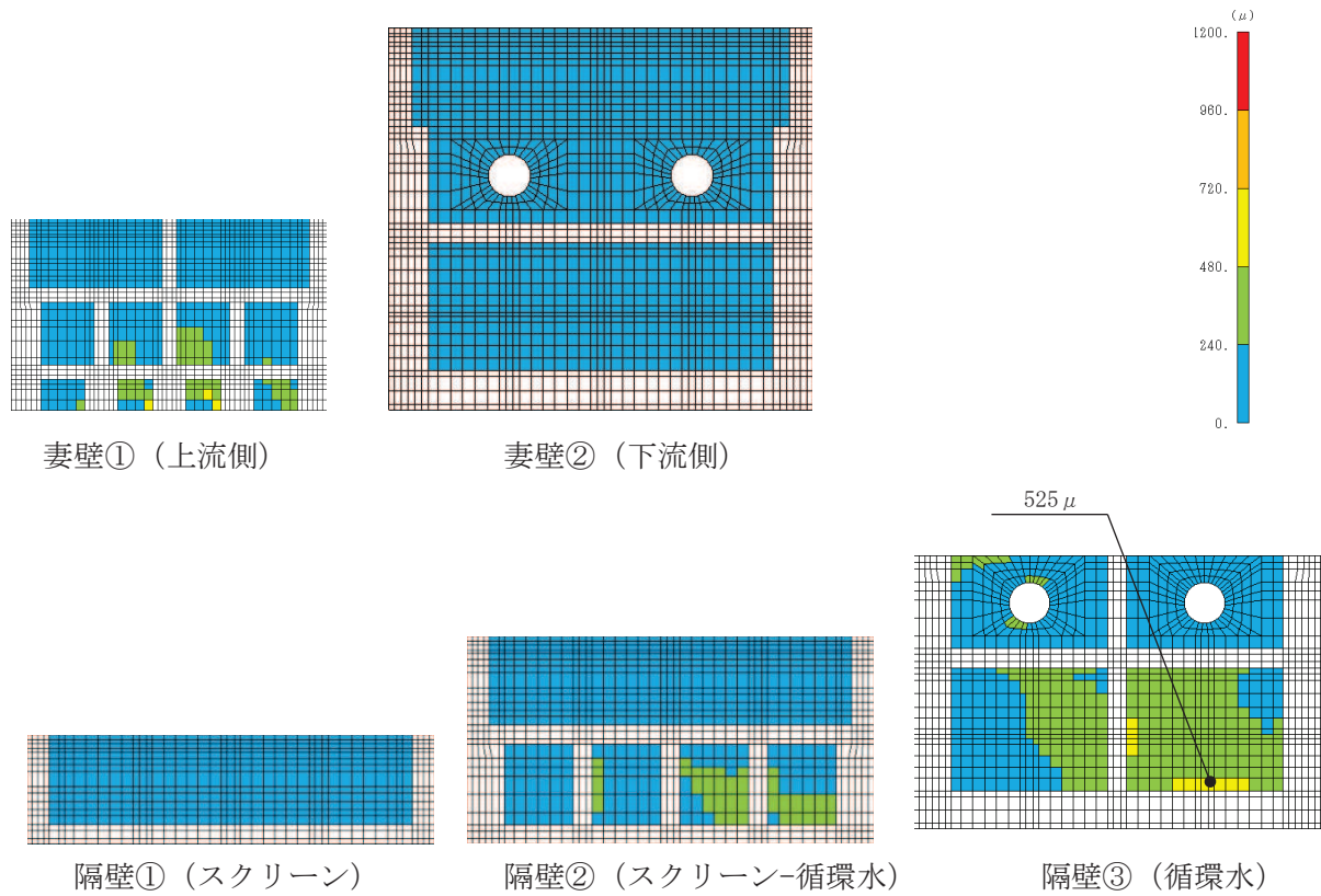
図 6-26(2) 曲げ・軸力系の破壊に対する照査値最大時のひずみ分布図 (全応力解析) (コンクリートの圧縮ひずみ)
