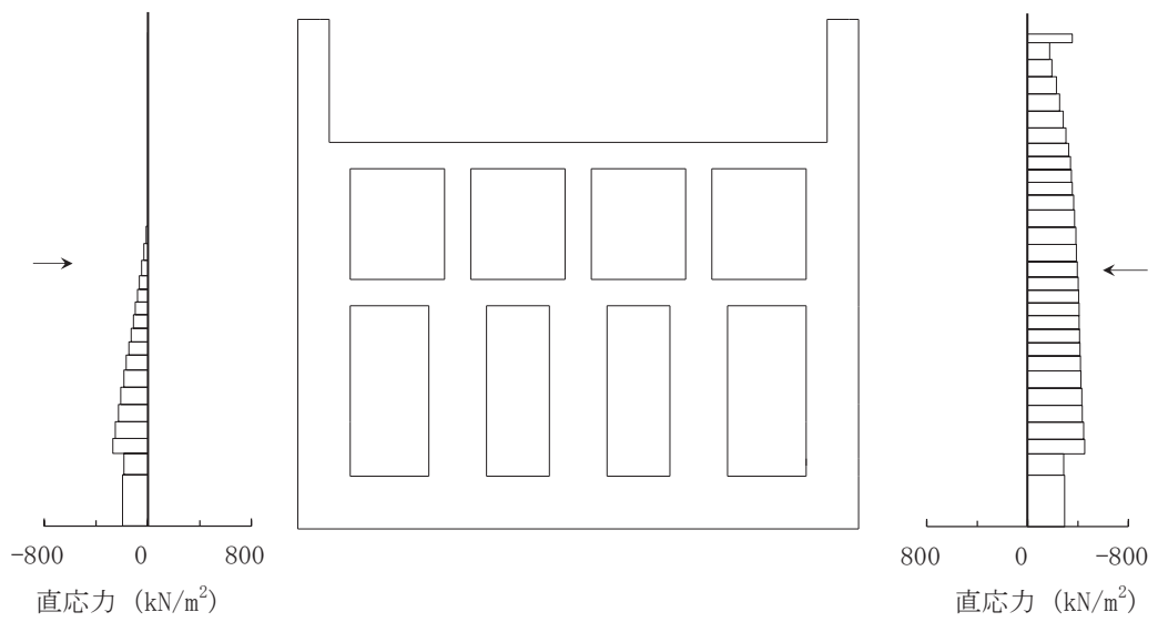
直応力
