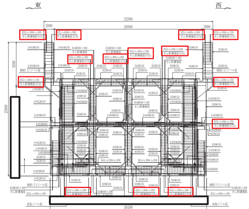
図 2-15 海水ポンプ室概略配筋図 (A-A 断面, 東西 (スクリーンエリア))
