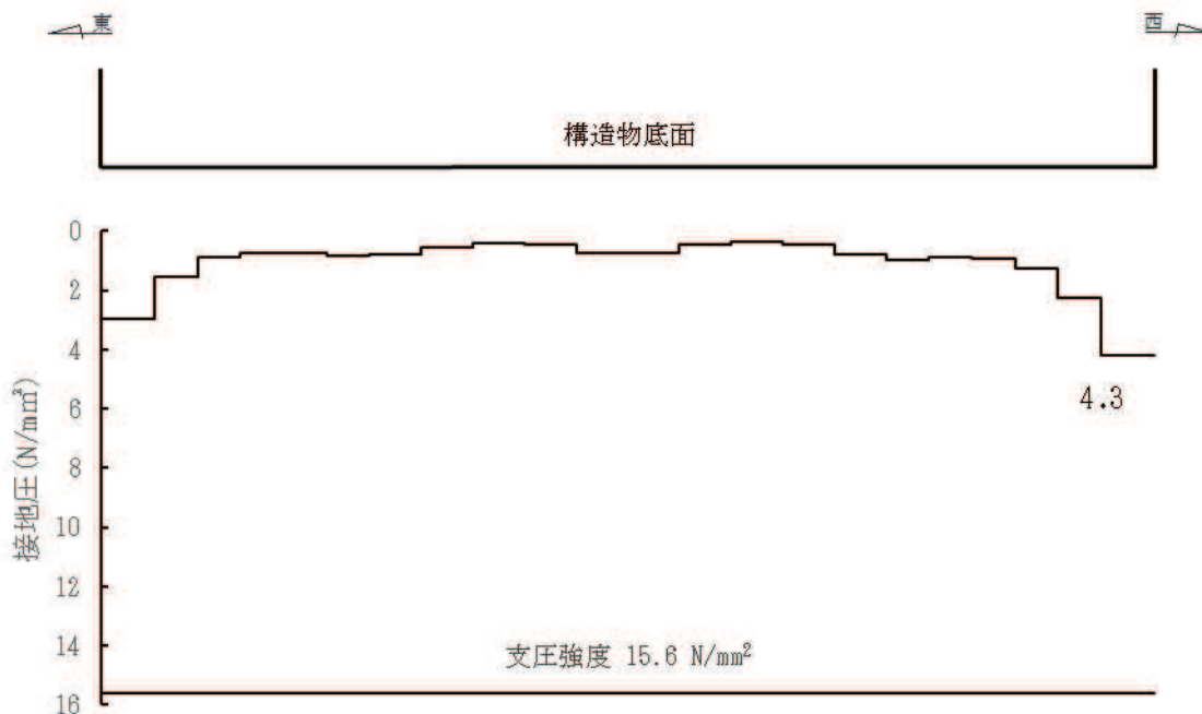
図5-11 MMR（既設）の最大接地圧分布図 (解析ケース①, S s -D2 (-+), スクリーンエリア)
