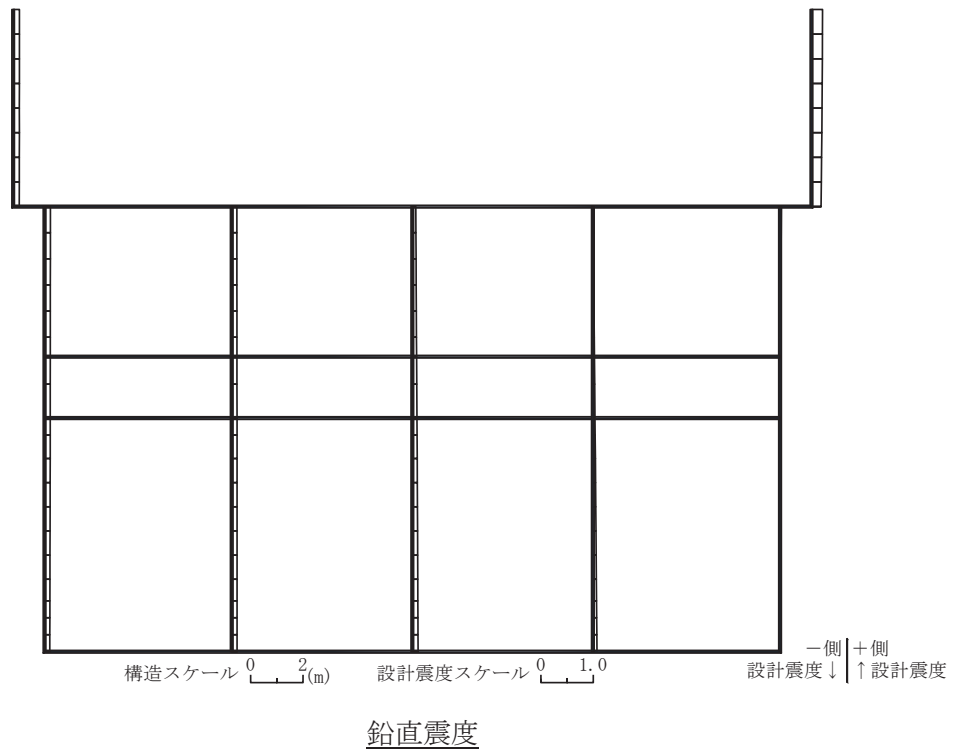
図 3-14 作用荷重分布図 (設計震度分布)
