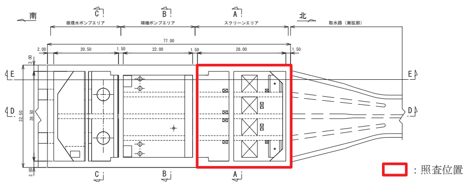
図5-12 照査位置図
