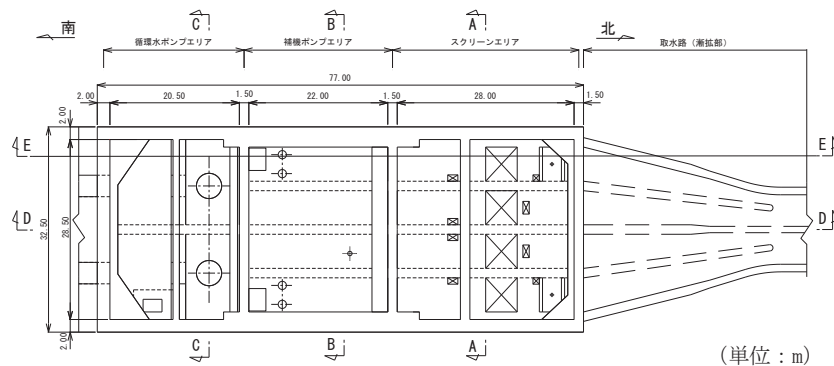
図3-1 海水ポンプ室の地震時荷重算出断面位置図
