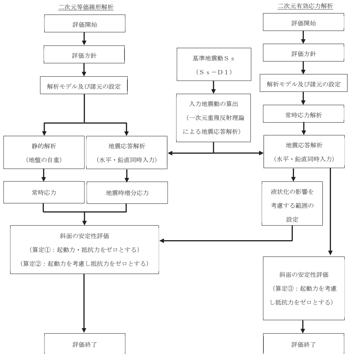
図 3.4-17 評価フロー
