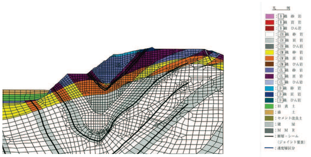
図 6. 2. 2-10 二次元有限要素法解析モデル図
