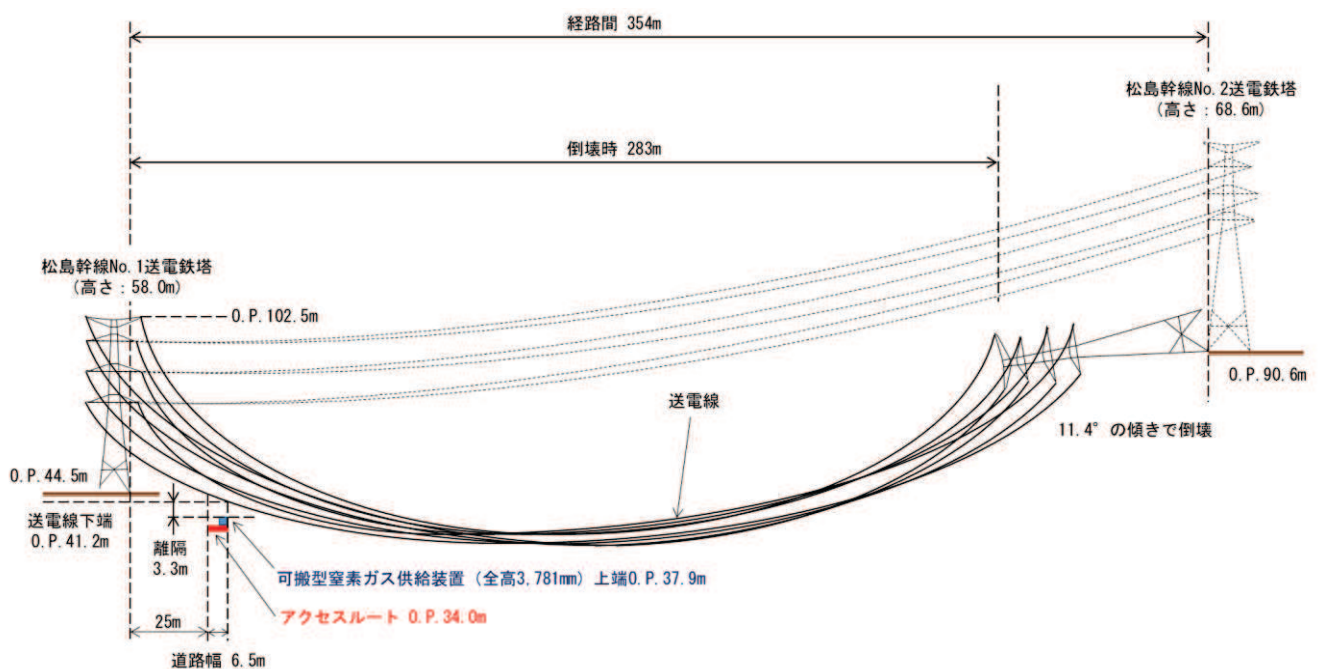
図 6. 2. 2-43 松島幹線 No. 2 送電鉄塔倒壊時の送電線状況
