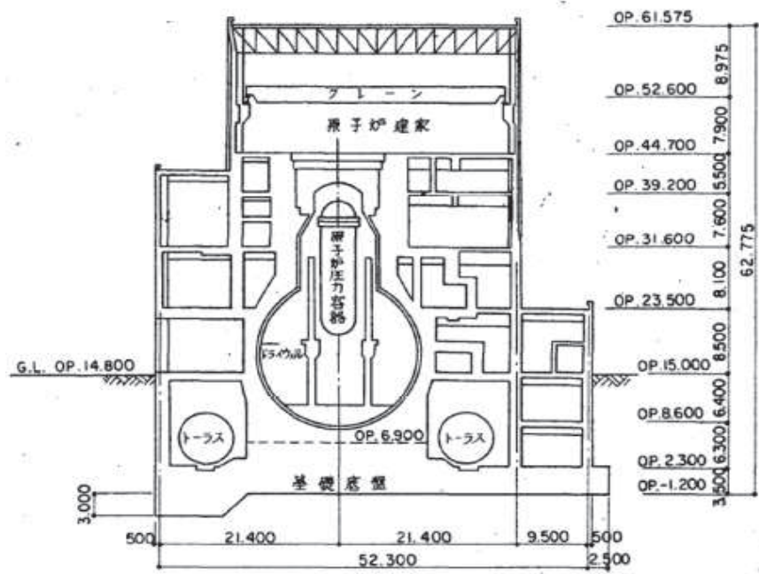
図 6. 3. 1-2 断面図
