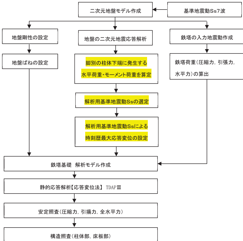
図 6.2.3-1 松島幹線 No.1 送電鉄塔 耐震性評価フロー
