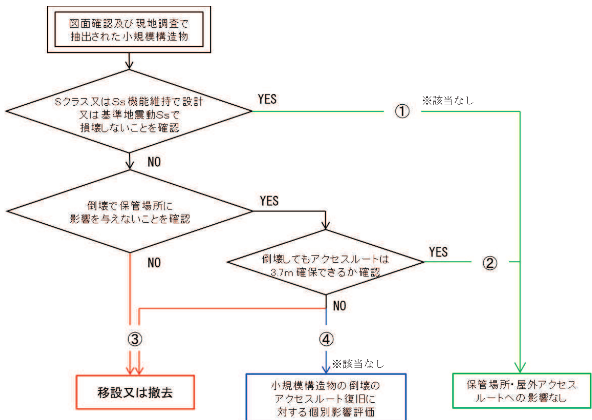
図 5-6 小規模構造物の個別影響評価要否判断フロー
