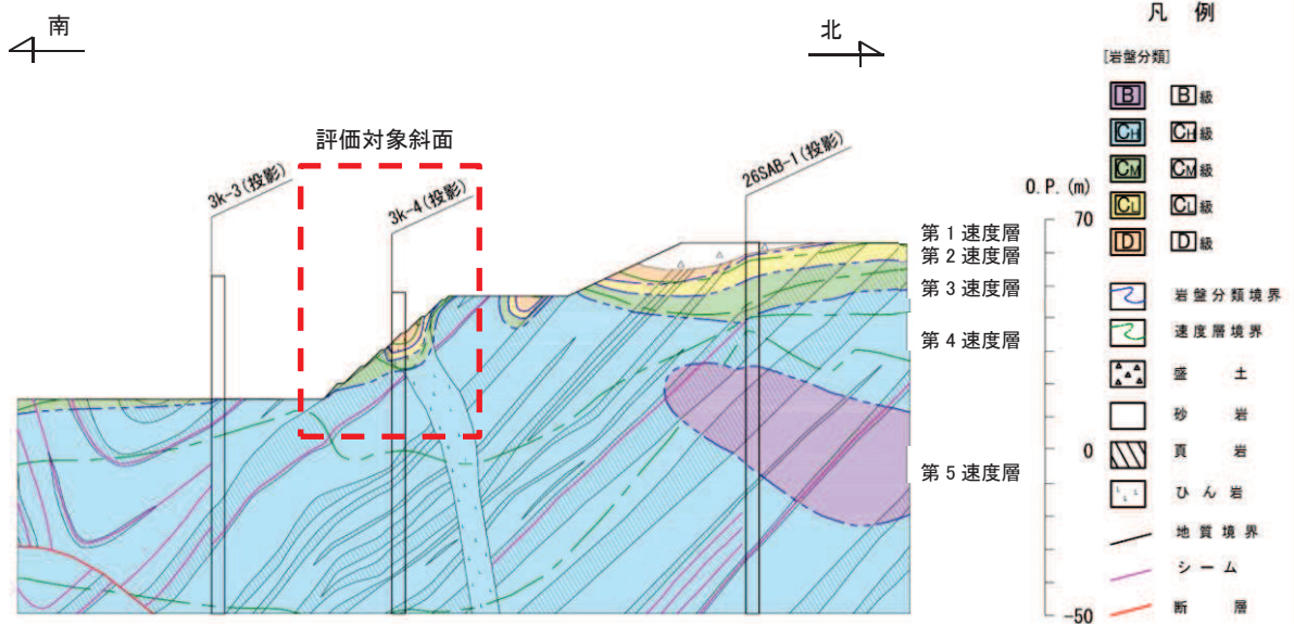
図 3.4-30 地質断面図
