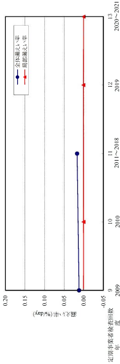
【 原子炉格納容器 漏えい率 】
