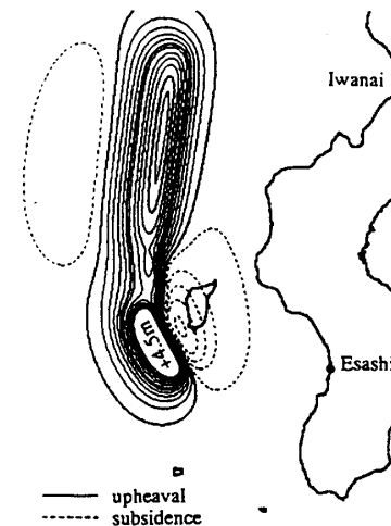
図1 地盤変位
