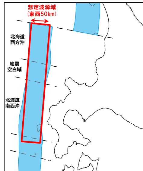
想定波源域(東西方向)の設定
