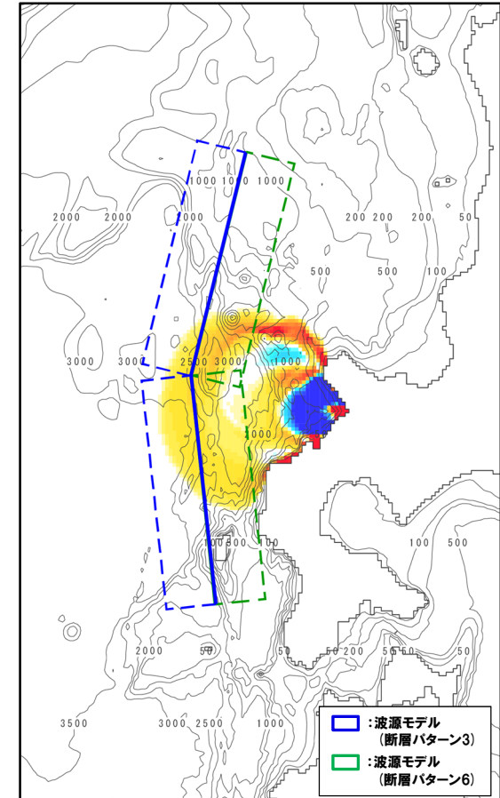
逆伝播解析結果, 波源モデル位置 (代表として断層パターン3, 6を示す)
