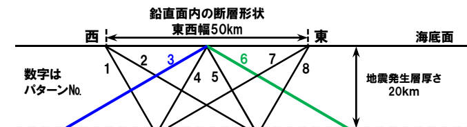
逆伝播解析結果, 波源モデル位置 (代表として断層パターン3, 6を示す)
