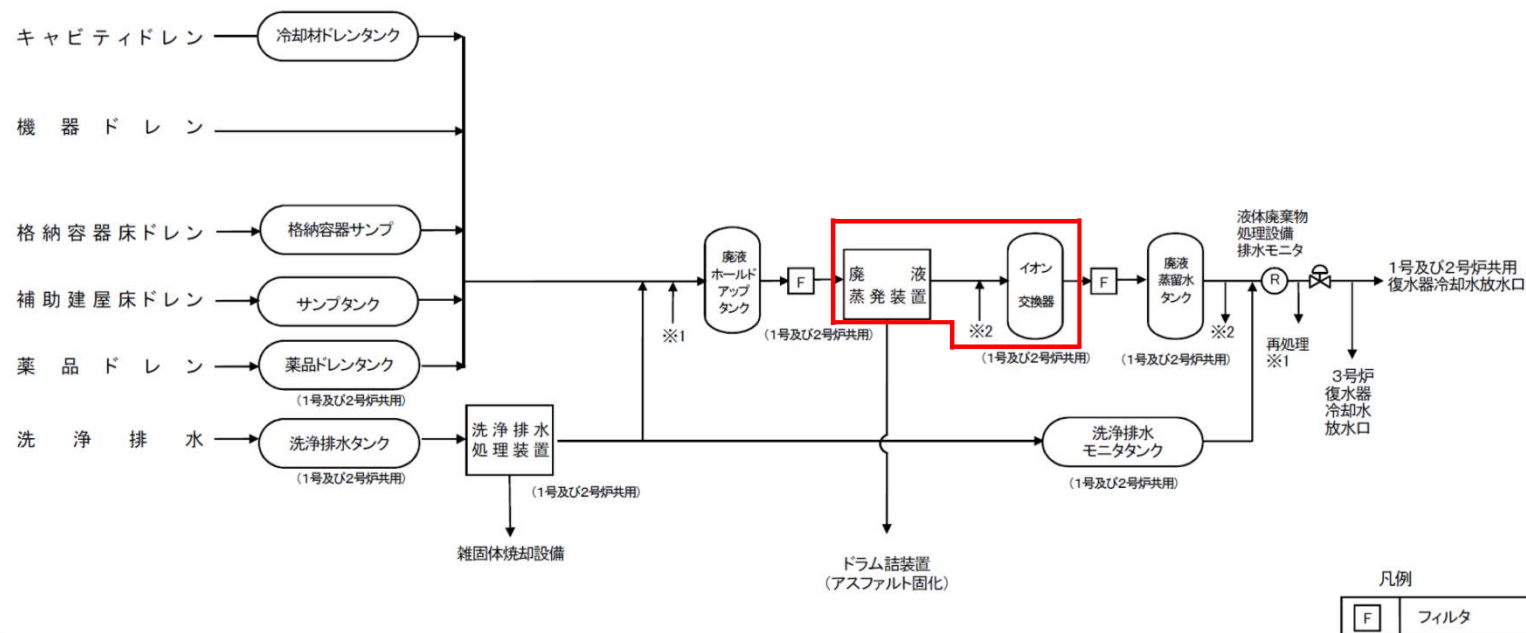
図1 放射性液体廃棄物の処理流路線図
