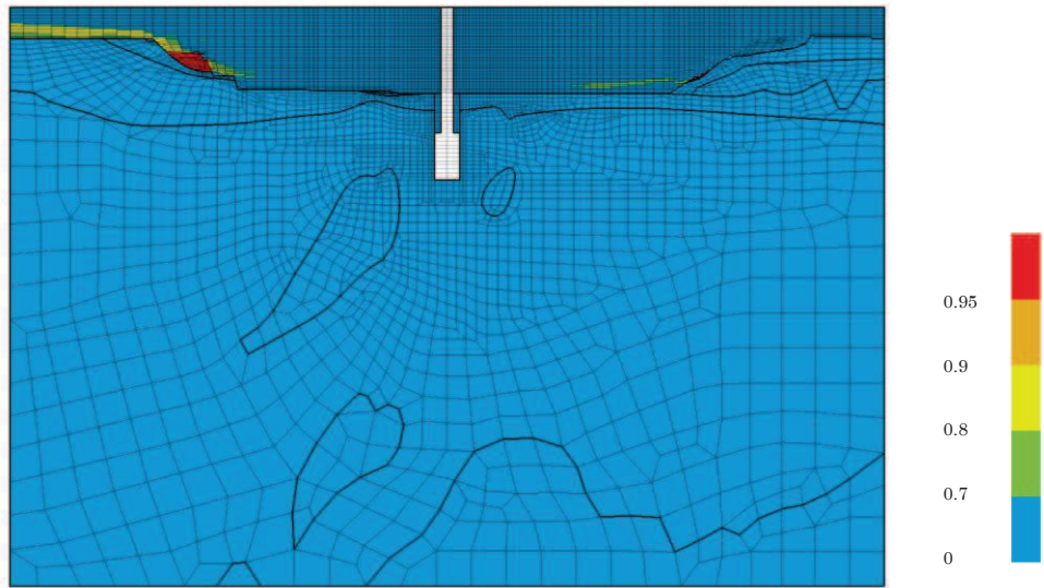
図 4-35(4) 最大過剰間隙水圧比分布 (No.2 揚水井戸, S_s - F1 (一+), 解析ケース②)
