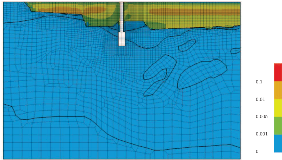
図 4-34(1) 最大せん断ひずみ分布 (No.1 揚水井戸, S s - N 1 (一+), 解析ケース①) (全応力解析)
