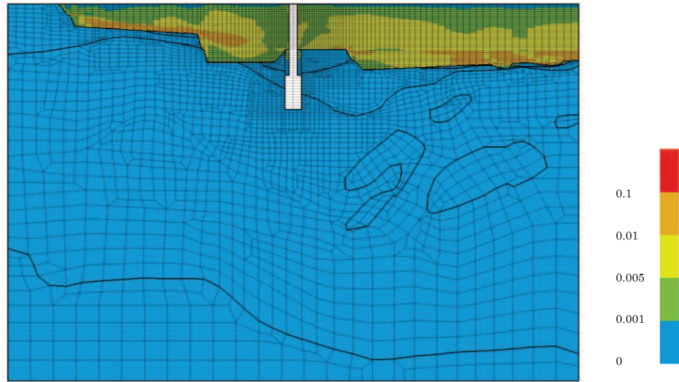
図 4-34(6) 最大せん断ひずみ分布 (No.1 揚水井戸, S_s - N1 (一十), 解析ケース②) (有効応力解析)
