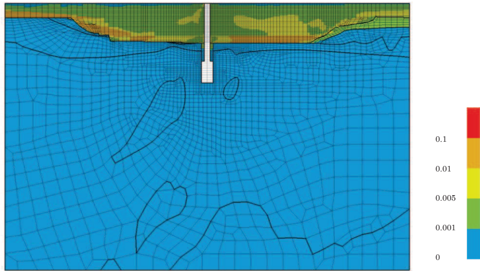
図 4-34(12) 最大せん断ひずみ分布 (No.2 揚水井戸, S_s - F1 (一十), 解析ケース③) (有効応力解析)
