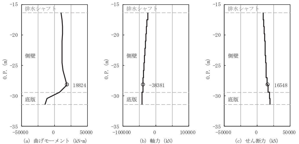
図 4-13(1) 集水ピット 軸方向照査におけるコンクリートの曲げ・軸力系の破壊に対する評価時刻での断面力 (No.1 揚水井戸, S s - N 1 (-+), 7.50s) 解析ケース①：基本ケース (全応力解析)
