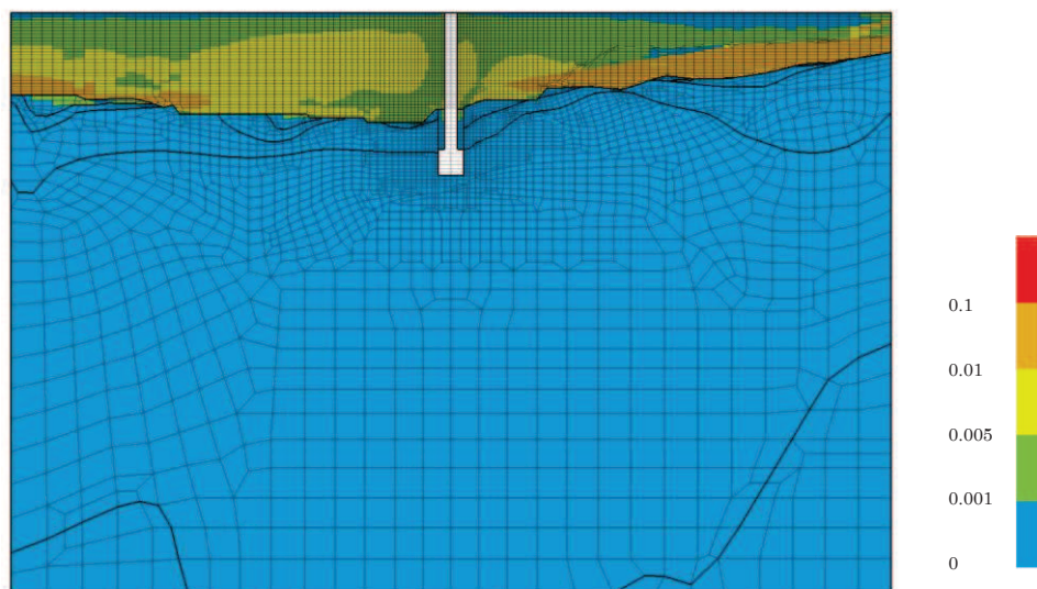
図 4-34(16) 最大せん断ひずみ分布 (No. 3 揚水井戸, S s -N1 (++) , 解析ケース②) (有効応力解析)
