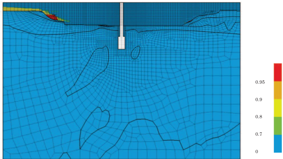
図 4-35(5) 最大過剰間隙水圧比分布 (No.2 揚水井戸, S_s - D2 (++) , 解析ケース②)
