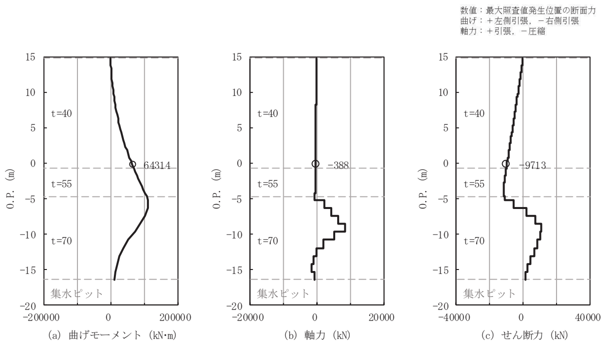
図 4-2(1) 排水シャフト 軸方向照査におけるせん断破壊に対する評価時刻での断面力 (No.1 揚水井戸 (板厚 t=40 mm), S s -N1 (++) , 7.73s)
