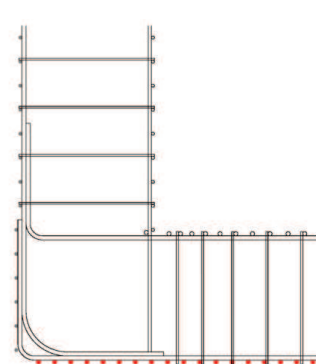
断面図
