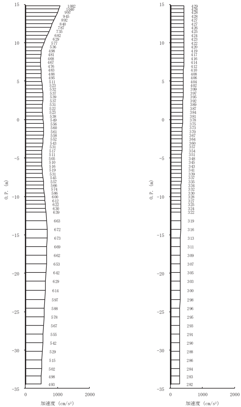
(a) S s - F 2 (++) 水平 (b) S s - F 2 (++) 鉛直 図 1-4(5) 最大加速度分布図 (5/7) (No. 4 揚水井戸)
