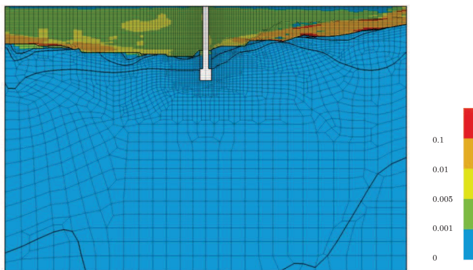
図 4-34(17) 最大せん断ひずみ分布 (No. 3 揚水井戸, S s -D1 (-+) , 解析ケース①) (有効応力解析)
