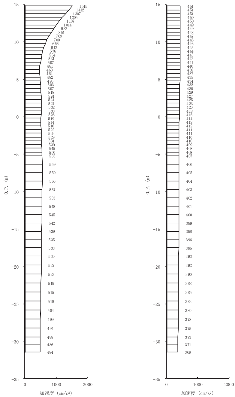
(a) S s - D 1 (++) 水平 (b) S s - D 1 (++) 鉛直 図 1-1(1) 最大加速度分布図 (1/7) (No. 1 揚水井戸)
