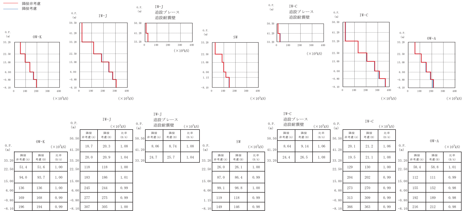
図 3.2-15 最大応答せん断力の比較 (O2R/B, NS 方向)
