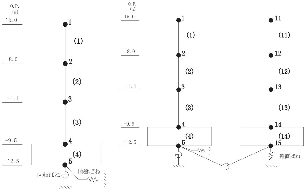
(a) 誘発上下動を考慮しないモデル
