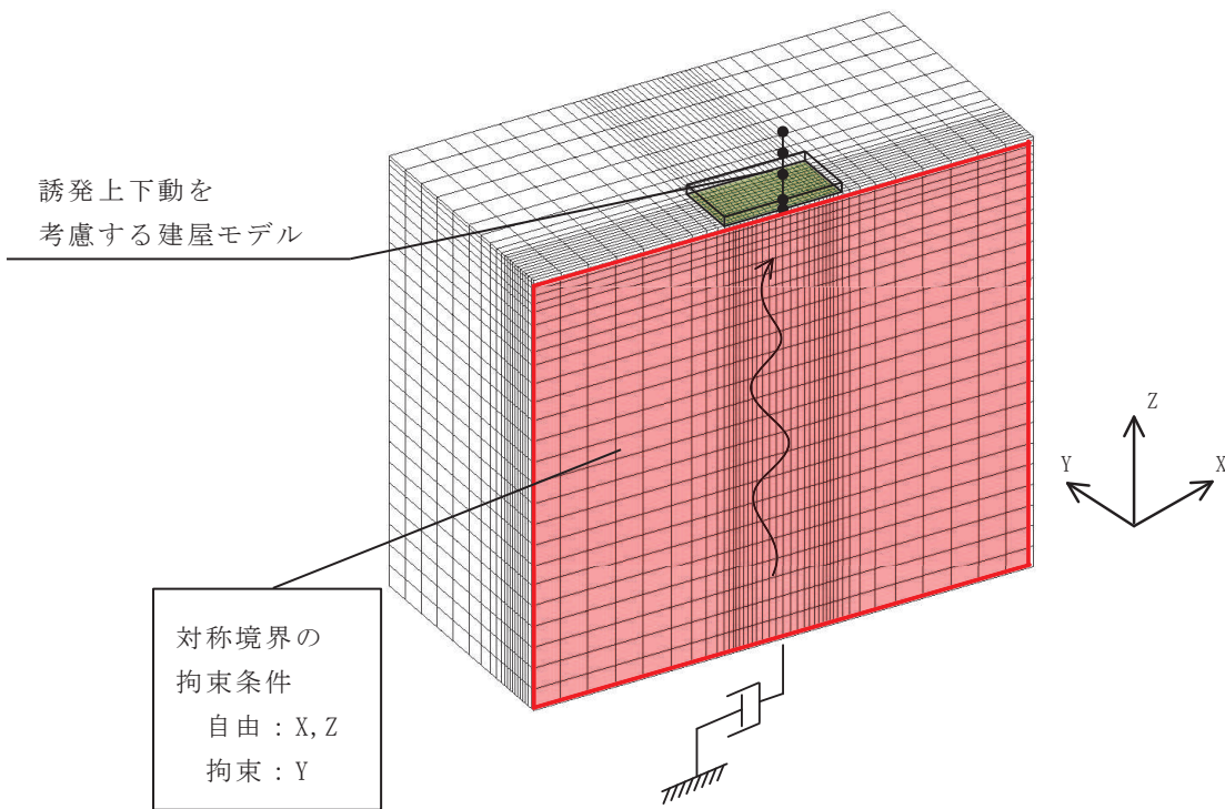
(c) 地盤 3 次元 FEM モデル
