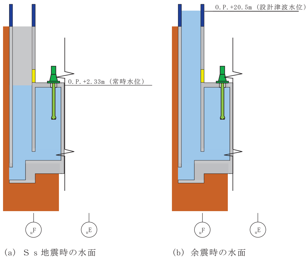
図3-2 水面高さ
