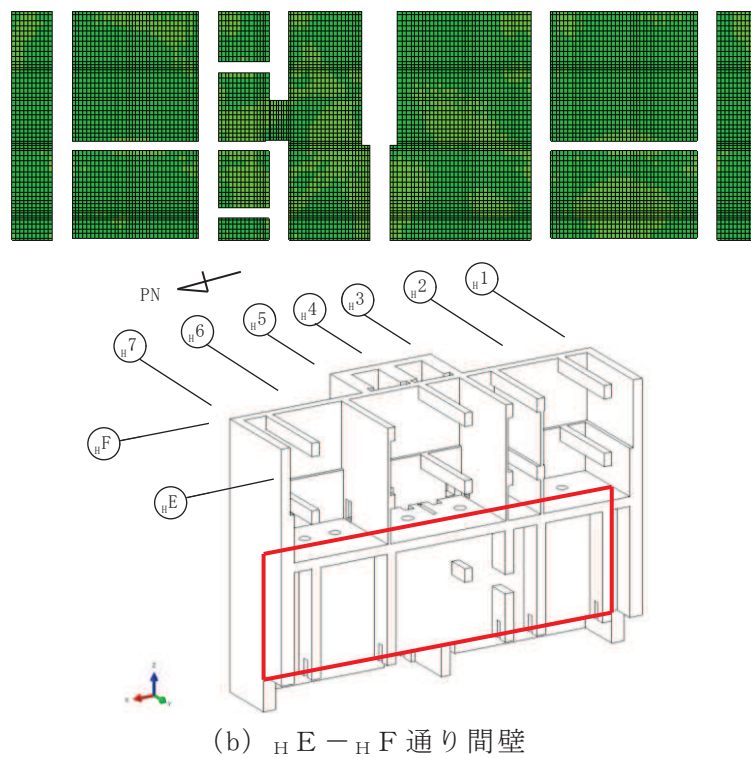
図 3-13(1) S_s 地震時鉄筋ひずみ (X, 横方向)
