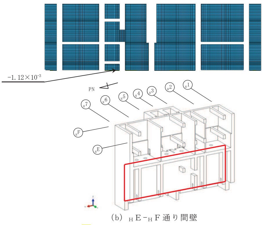
図 3-20(1) 余震時コンクリート最小主ひずみ
