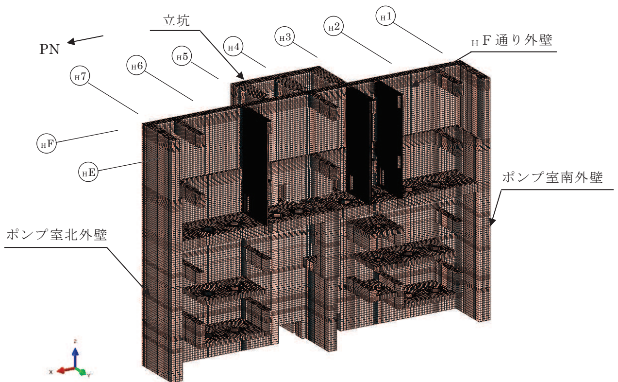
(a) 全体図
