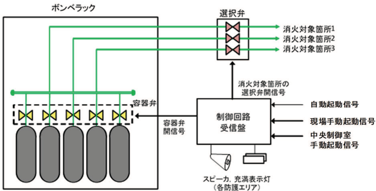
図2 ハロンガス消火設備（全域）概要（選択放出方式）
