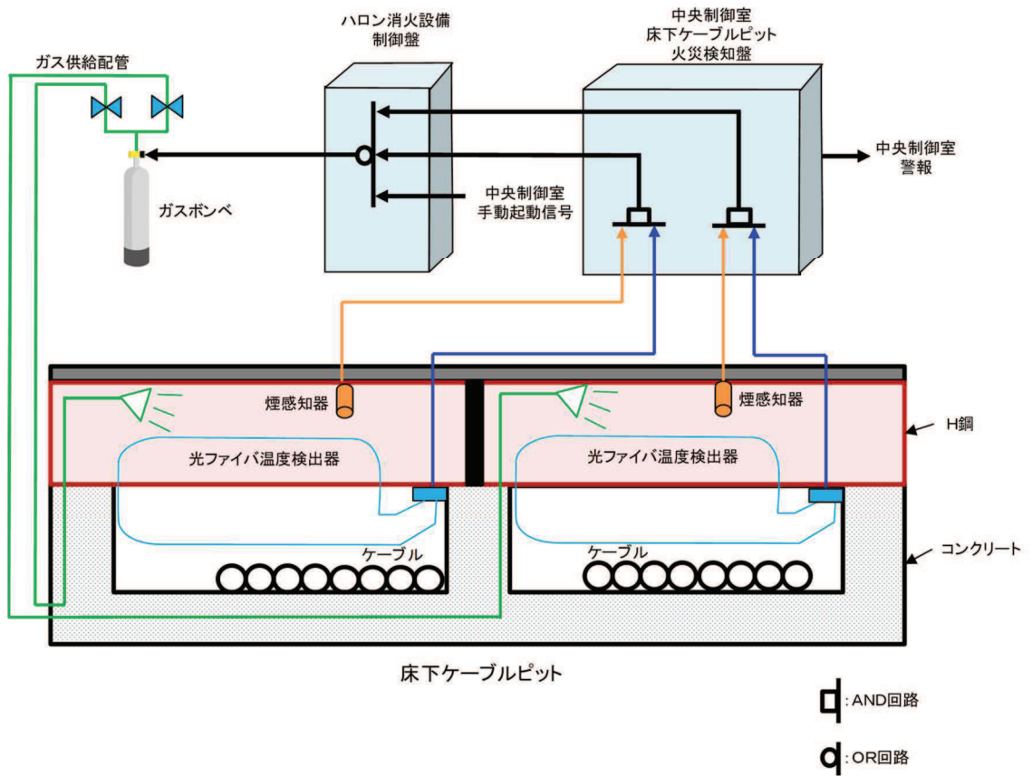
図5 ハロンガス消火設備（局所）（中央制御室床下ケーブルピット）概要
