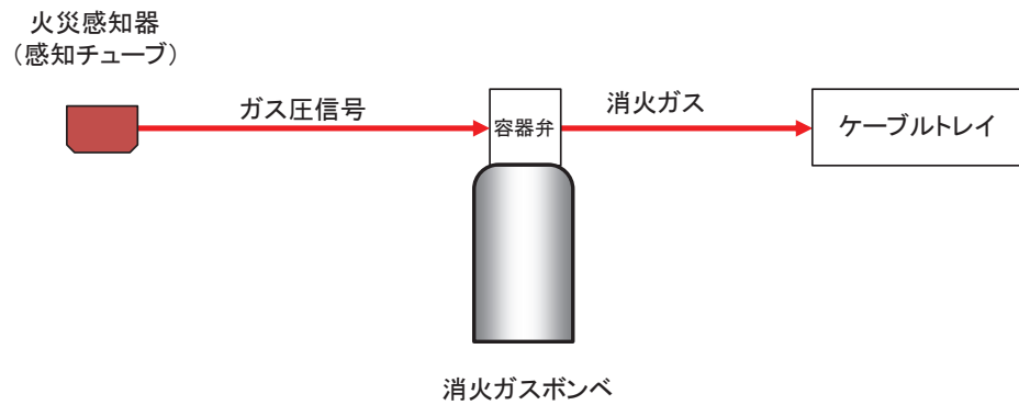
図 18 ケーブルトレイ消火設備の系統構成
