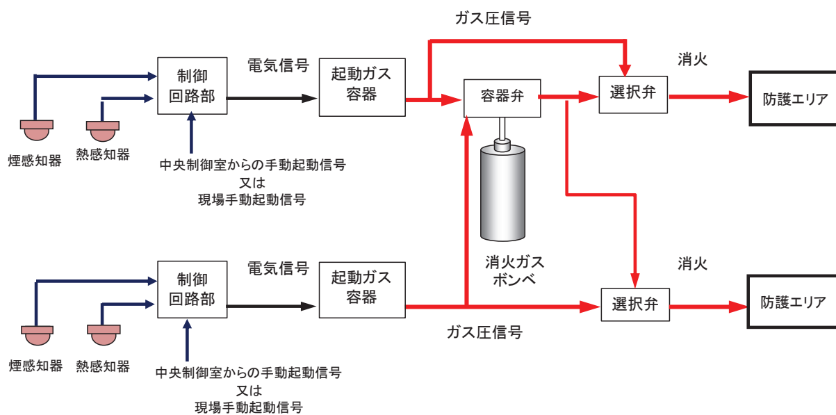
図 12 ハロンガス消火設備（全域）（選択式）の系統構成
