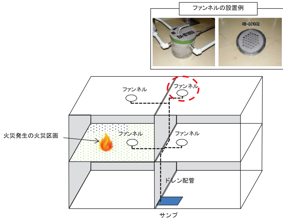
図5 建屋内排水系統概要
