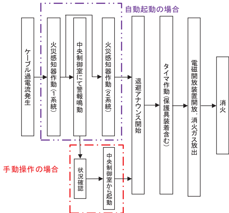
図 15 火災時の信号の流れ (中央制御室床下ケーブルピット)
