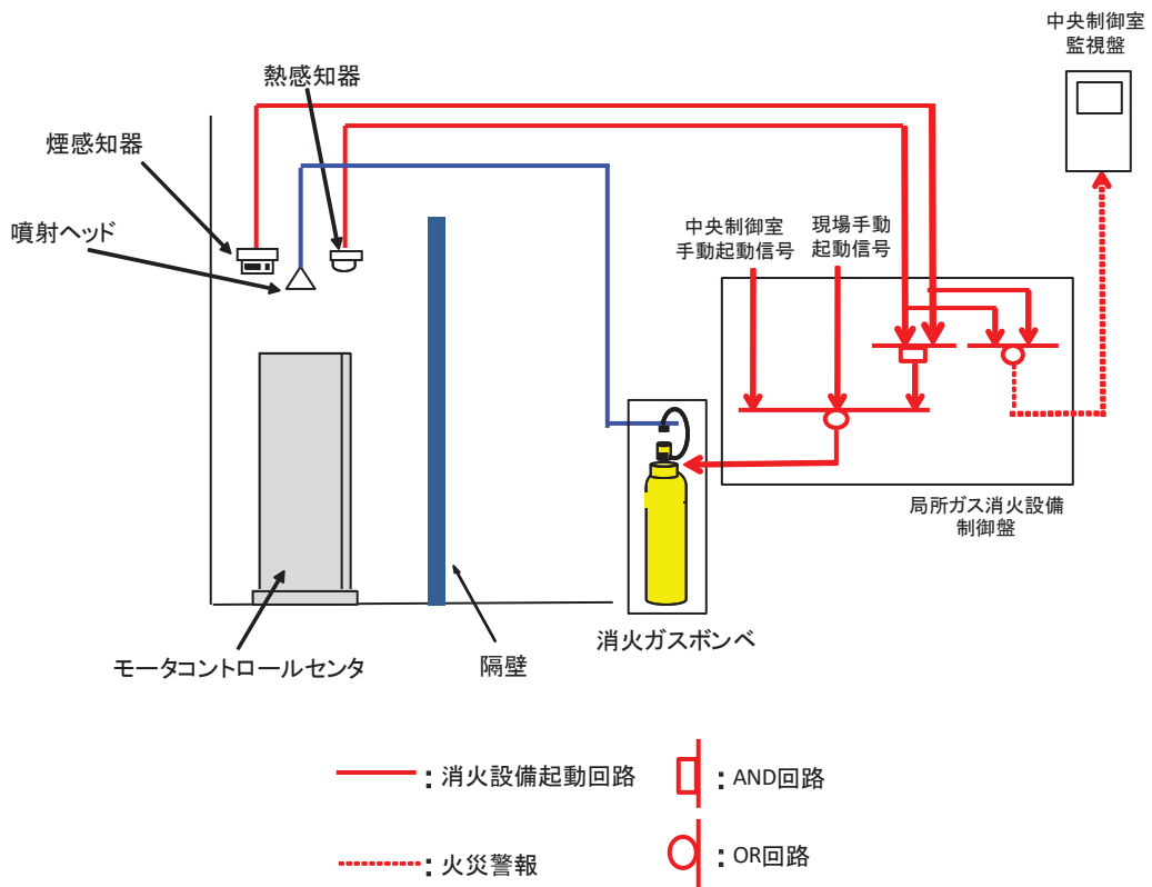
図4 ハロンガス消火設備（局所）（モータコントロールセンタ）概要
