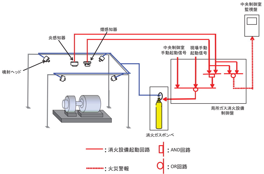
図3 ハロンガス消火設備（局所）（油内包機器）概要
