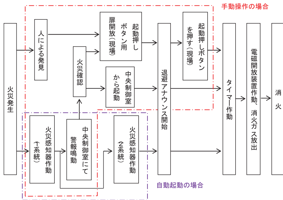
図13 火災時の信号の流れ（油内包機器）
