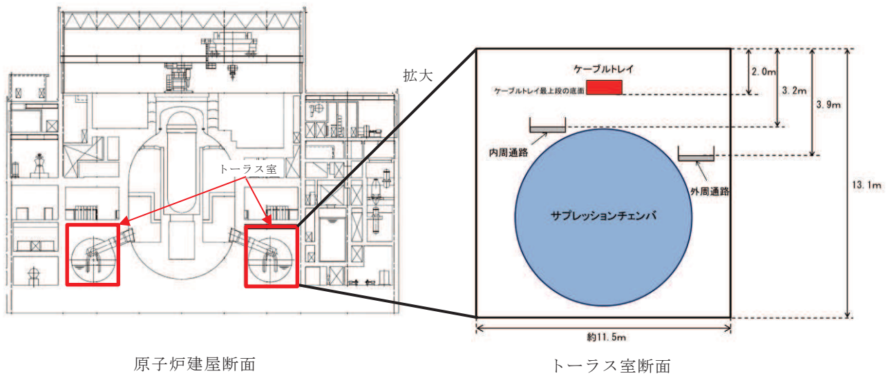
図2 原子炉建屋及びトラス室断面図
