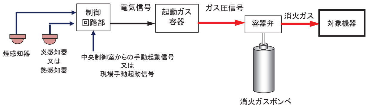
図 16 ハロンガス消火設備（局所）（油内包機器，モータコントロールセンタ）の系統構成
