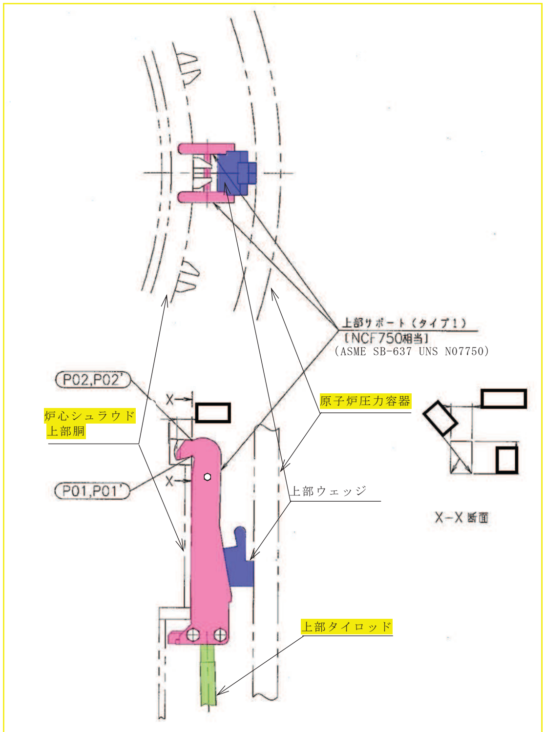
A部詳細
