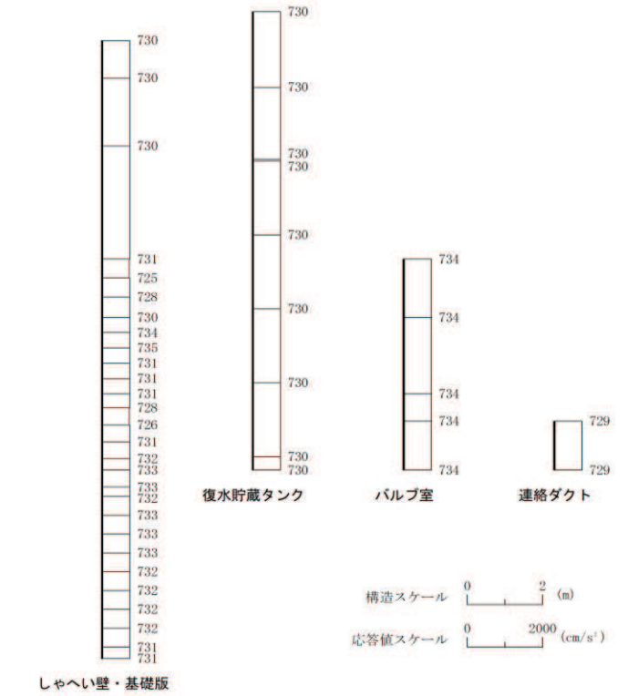
図 1-8(2) 最大加速度分布図 (解析ケース⑤, 東西方向)
