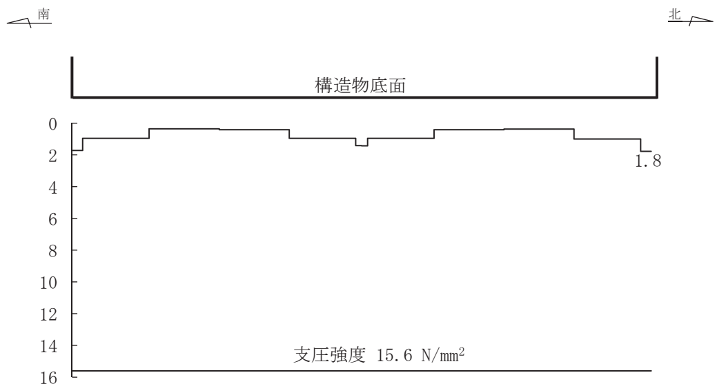
図 6-55(2) MMR (既設) の最大接地圧分布図 (断面④) (解析ケース⑥', S s -D2 (++))
