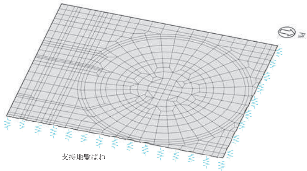
図4-8 地盤ばねの設定イメージ図（基礎版）
