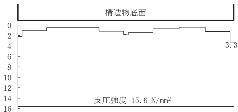
図 6-56(1) MMR (既設) 最大接地圧分布図 (断面⑤) (解析ケース③, S s -N1 (++) )
