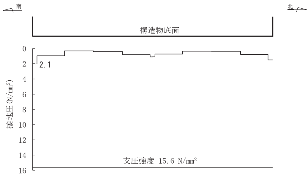
図 6-57(2) MMR (既設) の最大接地圧分布図 (断面⑥) (解析ケース⑧', S s -N1 (-+))
