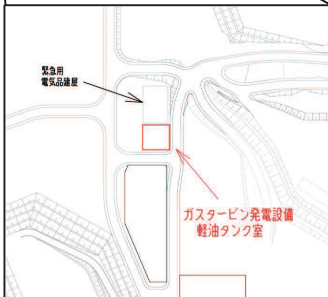
図 2-1 ガスタービン発電設備軽油タンク室の位置図
