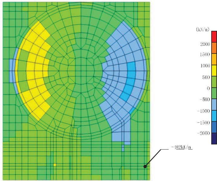
図 6-16(5) 曲げ・軸力系の破壊に対する照査値最大時の断面力分布図 (面内せん断力 ( \text{kN/m} ) : N_{xy} ) (解析ケース②, S_s - D 2 (++) , t=6.86\text{s} , 南北)
