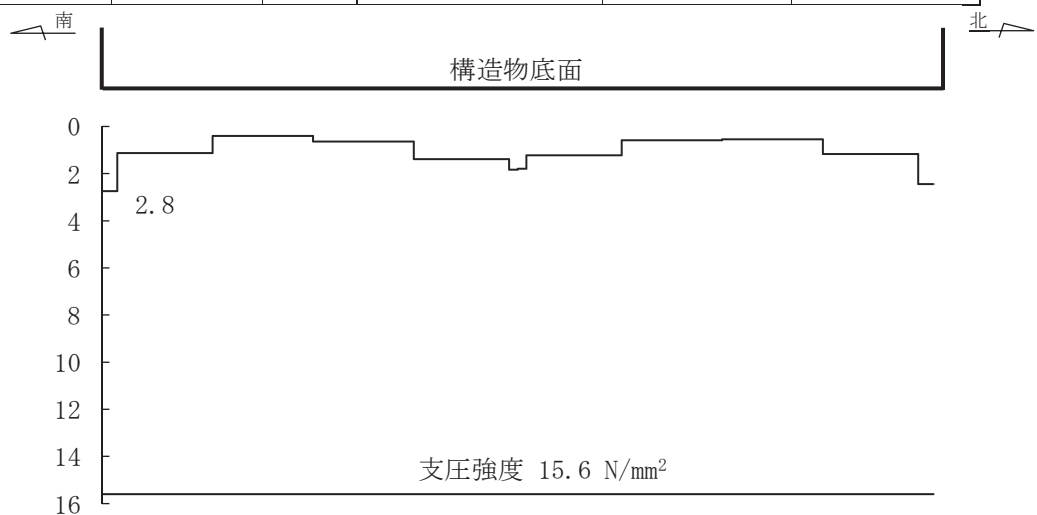
図 6-56(2) MMR (既設) 最大接地圧分布図 (断面⑤) (解析ケース⑧', S s -N1 (-+))
