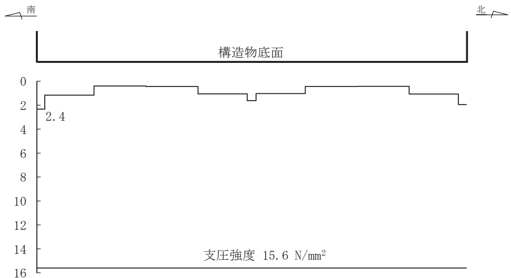
図 6-57(1) MMR (既設) の最大接地圧分布図 (断面⑥) (解析ケース①, S s -D1 (++) )
