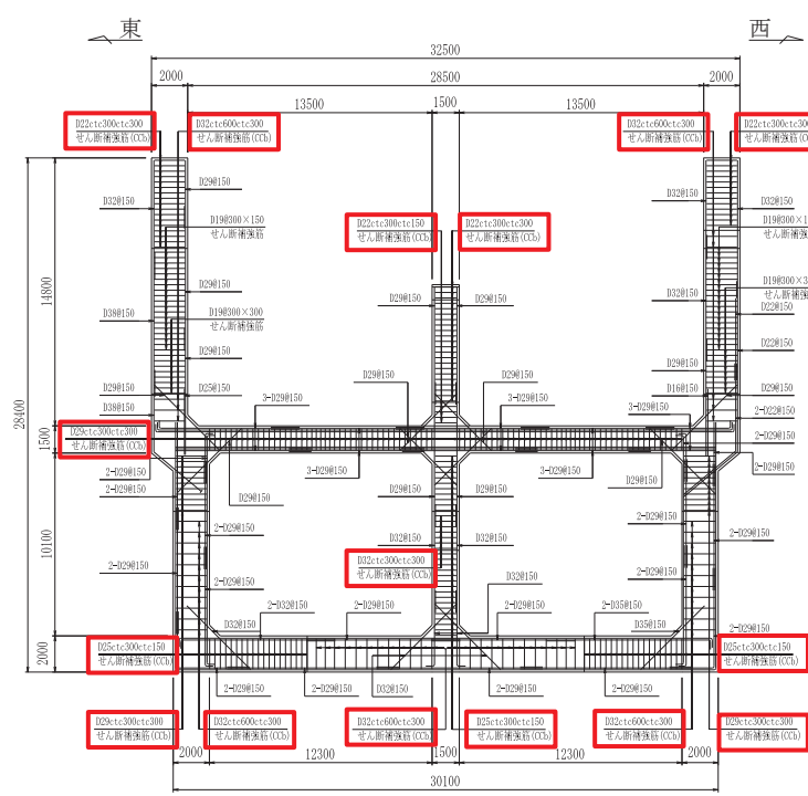
図 2-10 海水ポンプ室概略配筋図 (C-C 断面, 東西 (循環水ポンプエリア))
