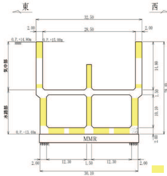
図 2-16 補強計画図 (C-C 断面, 東西 (循環水ポンプエリア))
