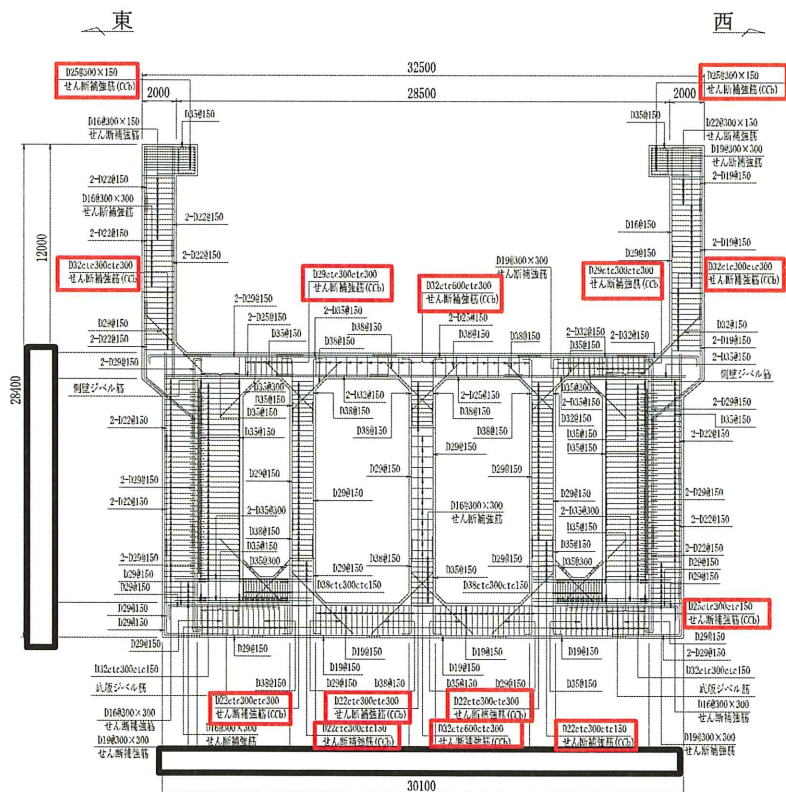
図 2-8 海水ポンプ室概略配筋図 (A-A 断面, 東西 (スクリーンエリア))
