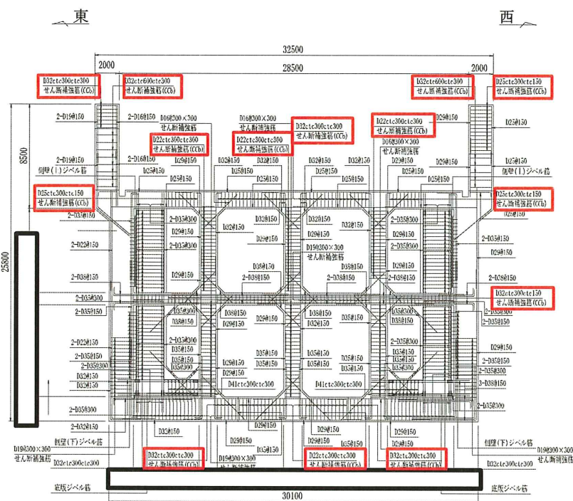
図 2-8 海水ポンプ室概略配筋図 (A-A 断面, 東西 (スクリーンエリア))
