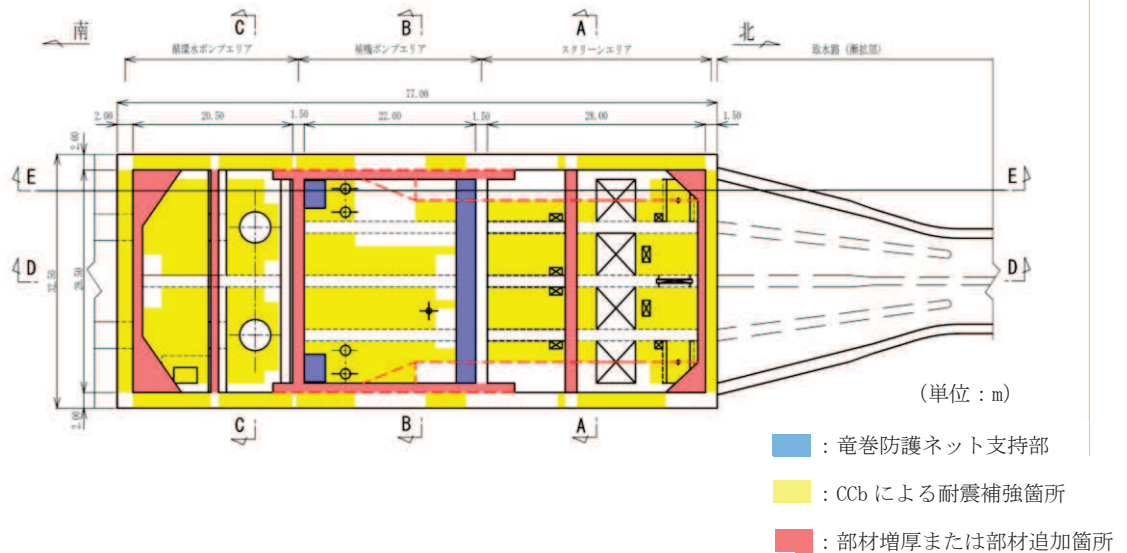
図 2-13 補強計画図 (平面図)
