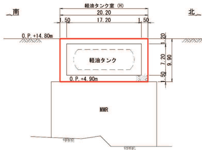
図 2-3(1) 軽油タンク室 (H) 断面図 (A-A 断面, 南北)
