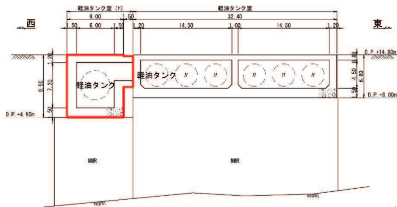
図 2-3(2) 軽油タンク室 (H) 断面図 (B-B 断面, 東西)
