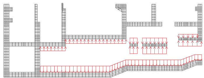
スクリーンエリア 補機ポンプエリア 循環水ポンプエリア (鉛直方向)
