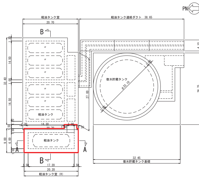
図 2-2 軽油タンク室 (H) 平面図
