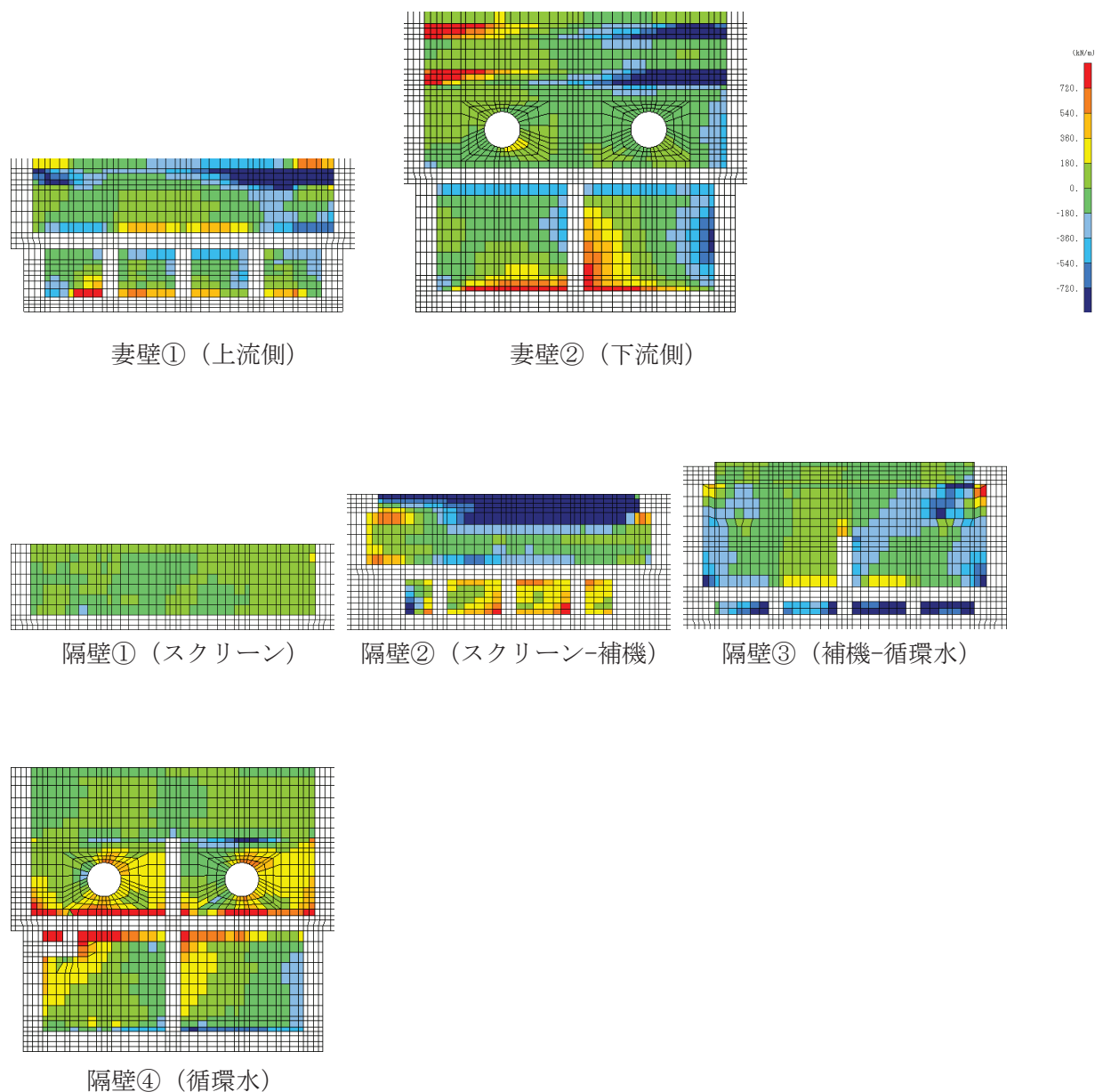
図 6-28(2) せん断破壊に対する照査値最大時の断面力分布図
