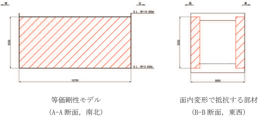
図 3-10 等価剛性モデル (A-A 断面, 南北)
