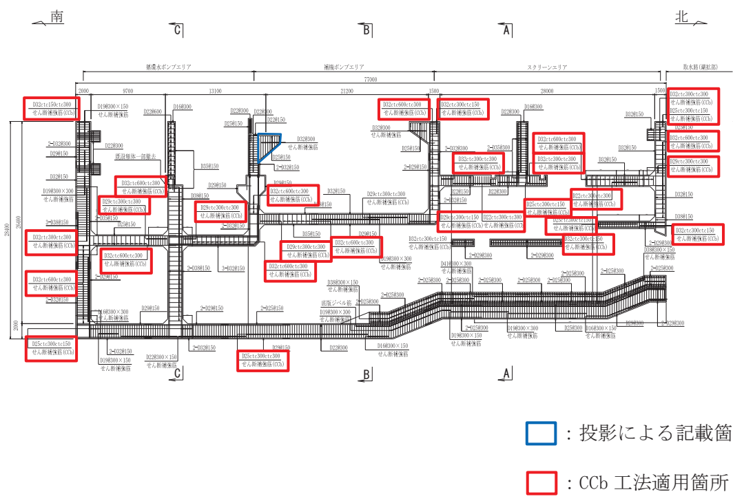
図 2-11 海水ポンプ室概略配筋図 (D-D 断面, 南北)
