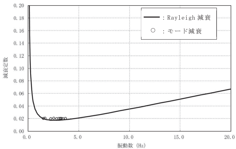
図 3-3 設定した Rayleigh 減衰
