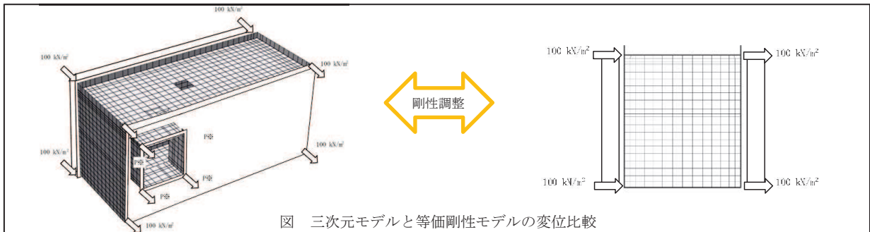
図 三次元モデルと等価剛性モデルの変位比較
