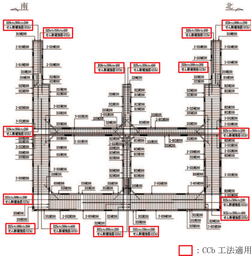
図 2-7 第 3 号機海水ポンプ室概略配筋図 (B-B 断面, 南北 (循環水ポンプエリア))
