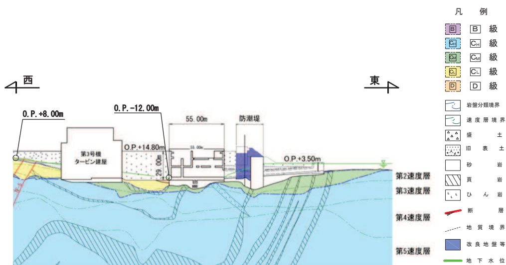
図 2-27 設計用地下水位 (C-C 断面, 東西)
