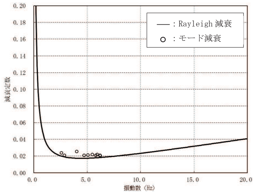
図 3-22 設定した Rayleigh 減衰 (A-A 断面, 南北 (スクリーンエリア))
