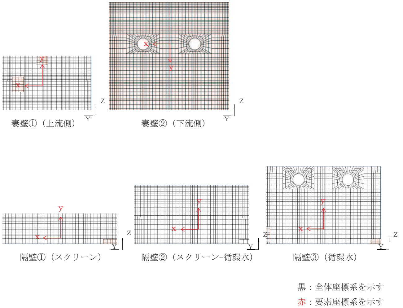
図 4-2(2) 各部材の要素座標系
