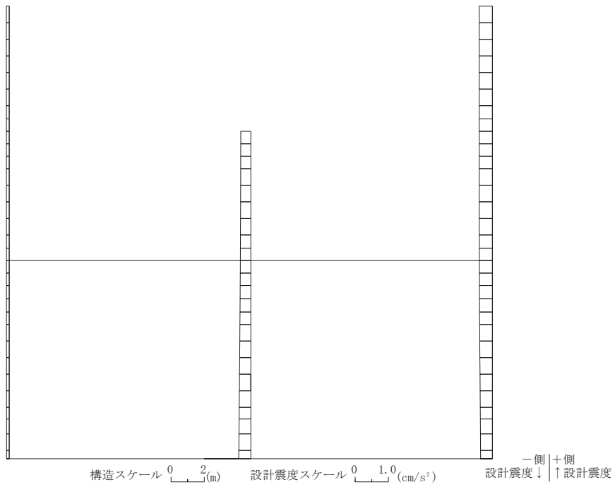
図 6-4(1) 作用荷重分布図 (設計震度分布) (全応力解析)
