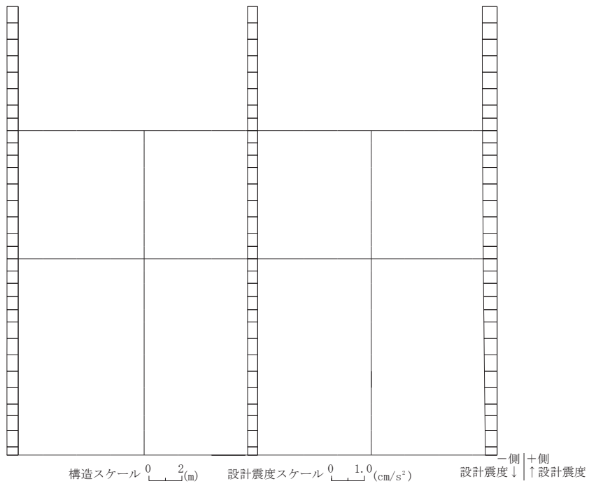
図 6-2(1) 作用荷重分布図 (設計震度分布) (全応力解析)
