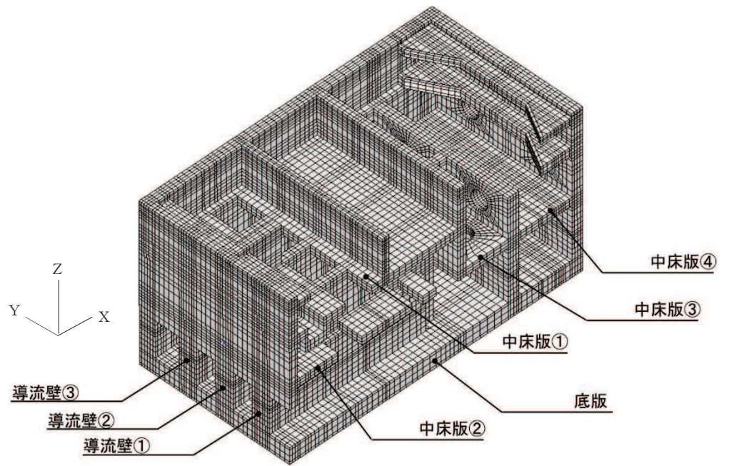
図 2-22 評価部位の位置
