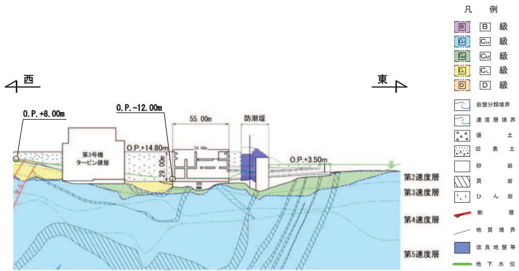
図 2-21 第 3 号機海水ポンプ室 地震時荷重算出用地質断面図 (C-C 断面, 東西)
