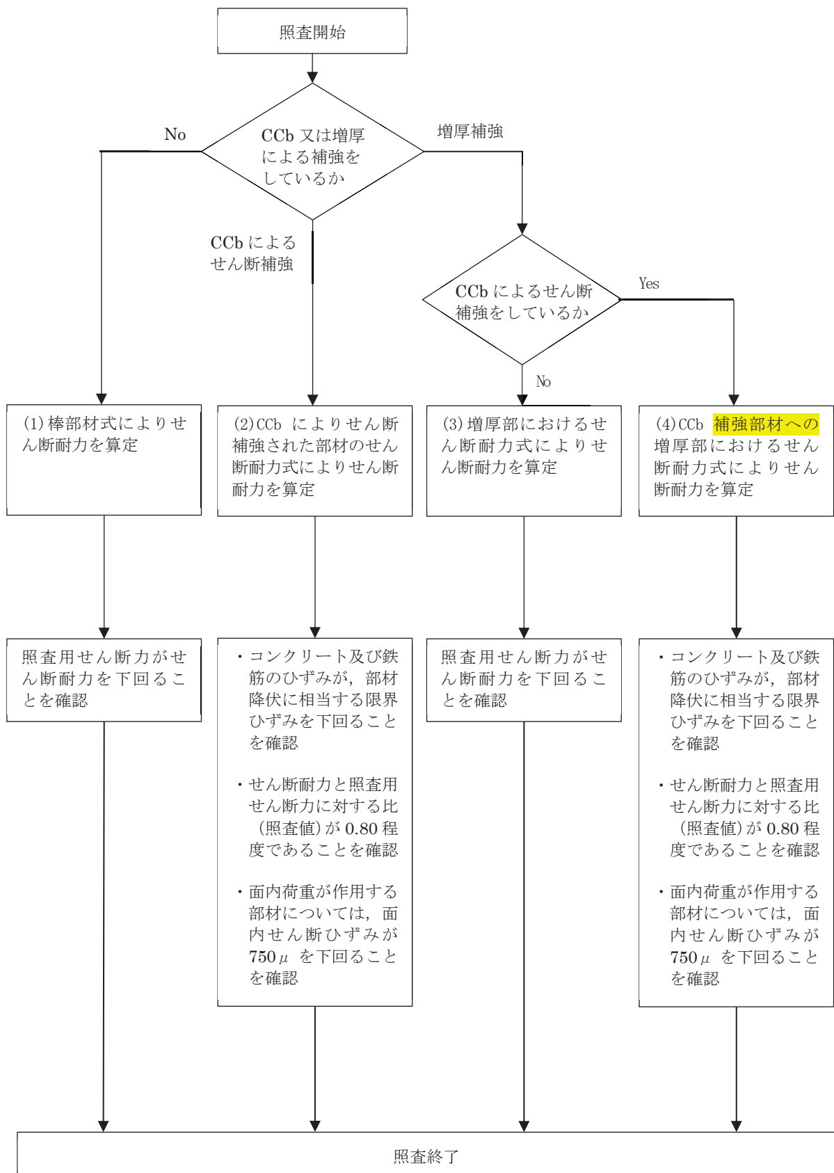
図 5-35 せん断破壊に対する照査フロー
