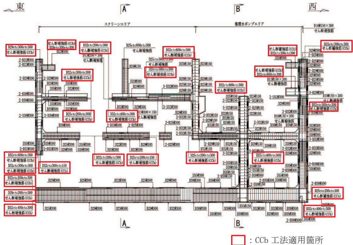
図 2-8 第 3 号機海水ポンプ室概略配筋図 (C-C 断面, 東西)
