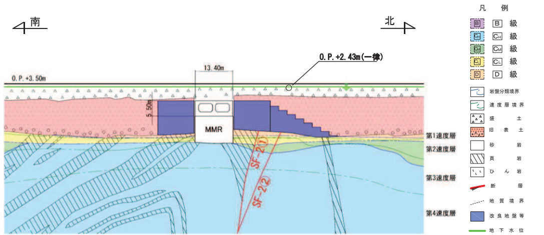
图 3-3 取水路（標準部） 地震時荷重算出用地質断面図（断面②）
