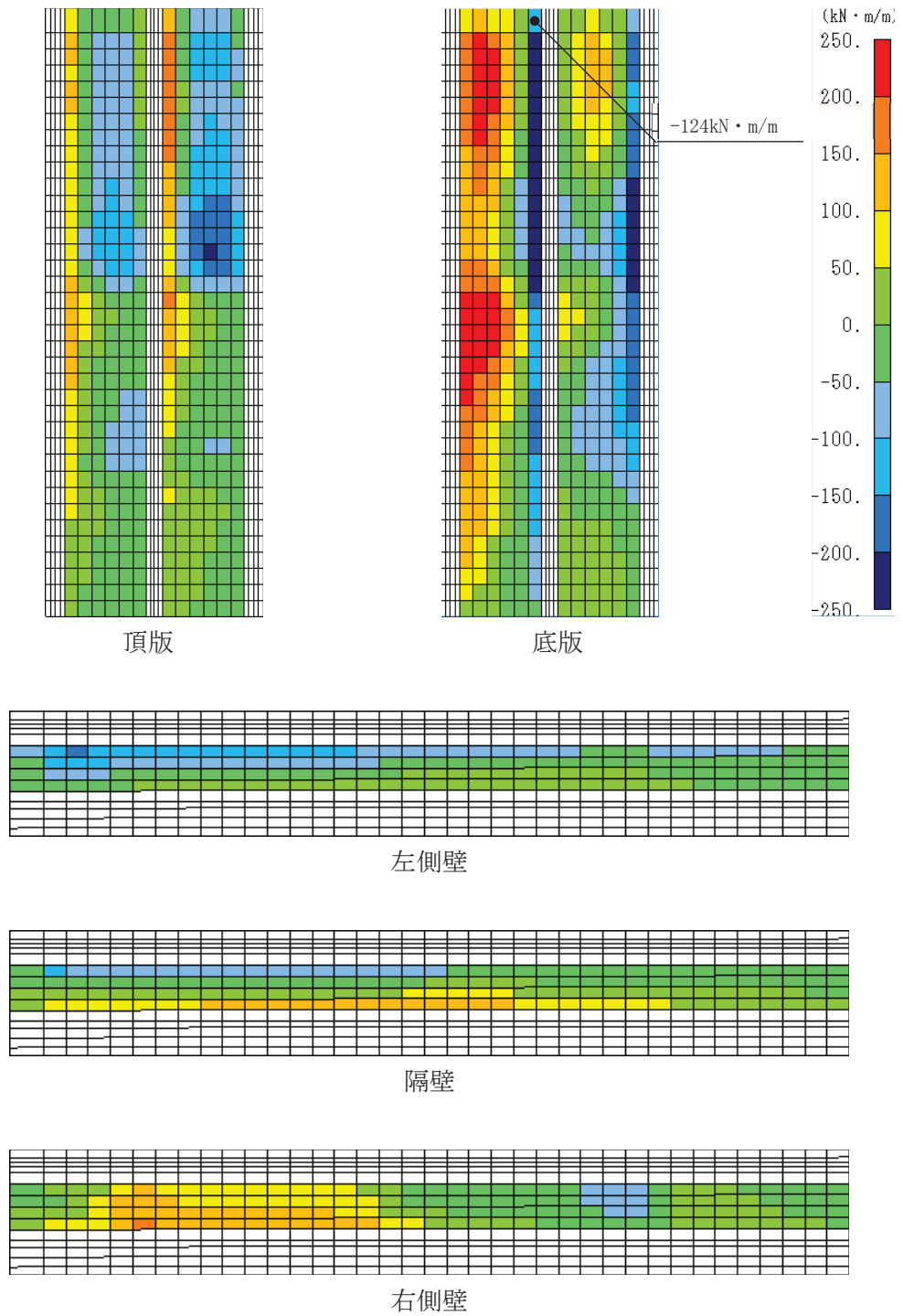
図 4-27 せん断破壊に対する照査における照査値最大時の断面力分布図 (曲げモーメント (kN · m/m) : My) (直線部, 底板, 解析ケース④', S s -F3 (++)
