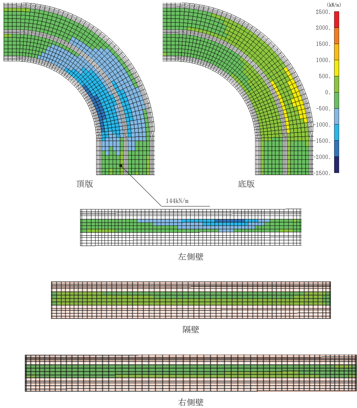
図 4-35 せん断破壊に対する照査における照査値最大時の断面力分布図 (軸力 (kN/m) : N_y ) (曲線部, 頂版, 解析ケース③, S_s - N 1 (++) )
