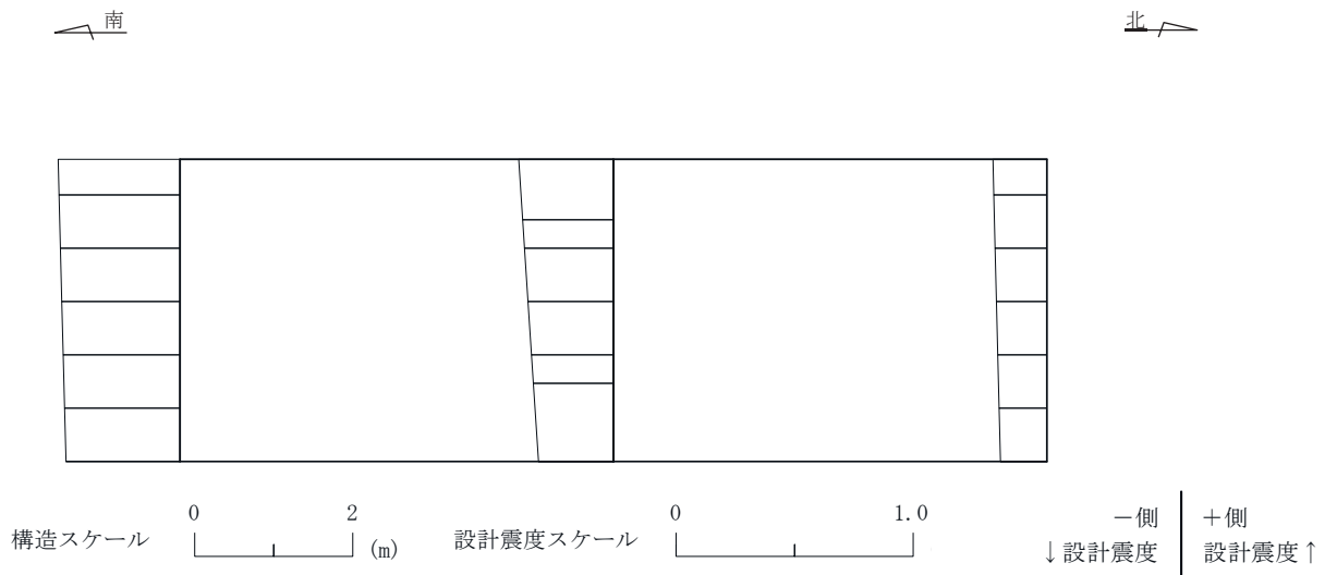
図 3-115 作用荷重分布図 (設計震度分布) (断面③：直線部，解析ケース③，S s -N1 (++) )
