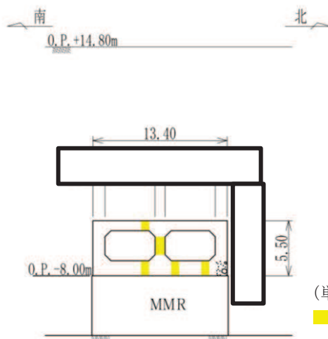
図 2-4(3) CCbによる耐震補強箇所 (②断面, 曲線部; 取水口側)
