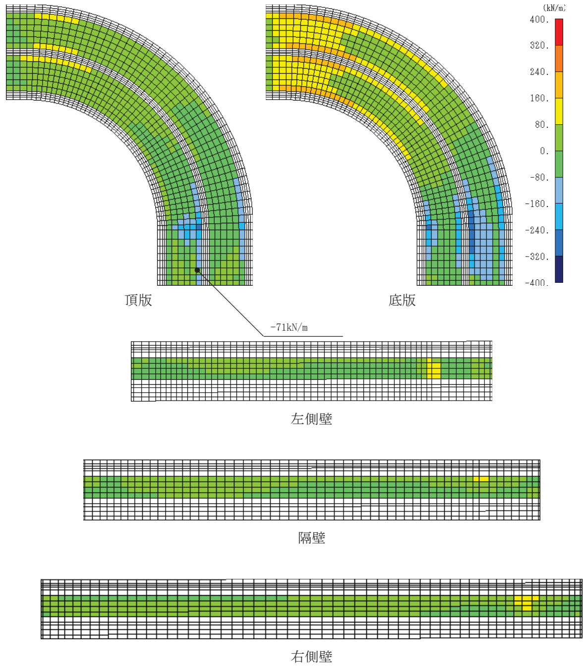
図 4-37 せん断破壊に対する照査における照査値最大時の断面力分布図
