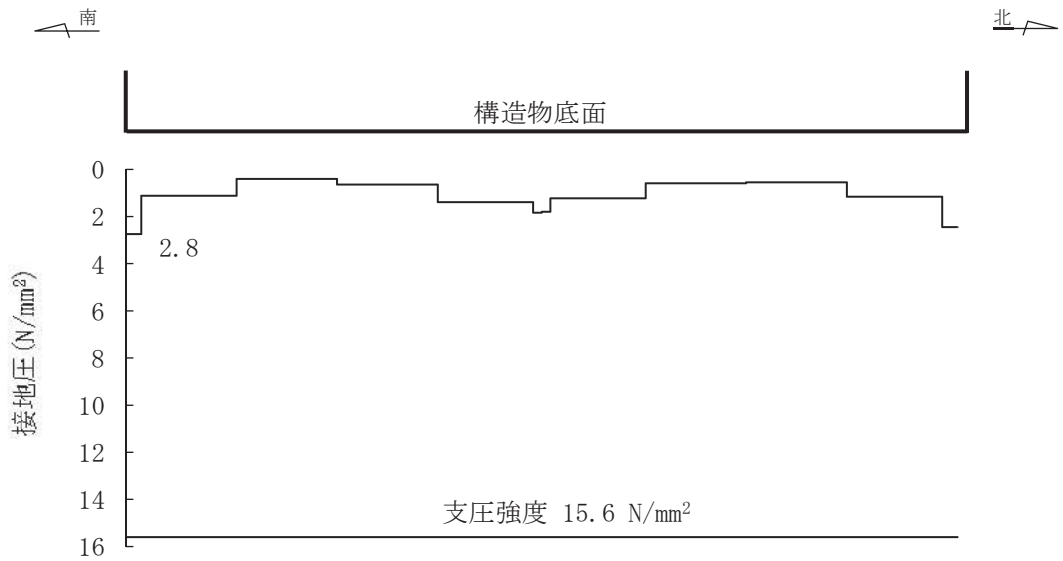
図 6-7 MMR (既設) の最大接地圧分布図
