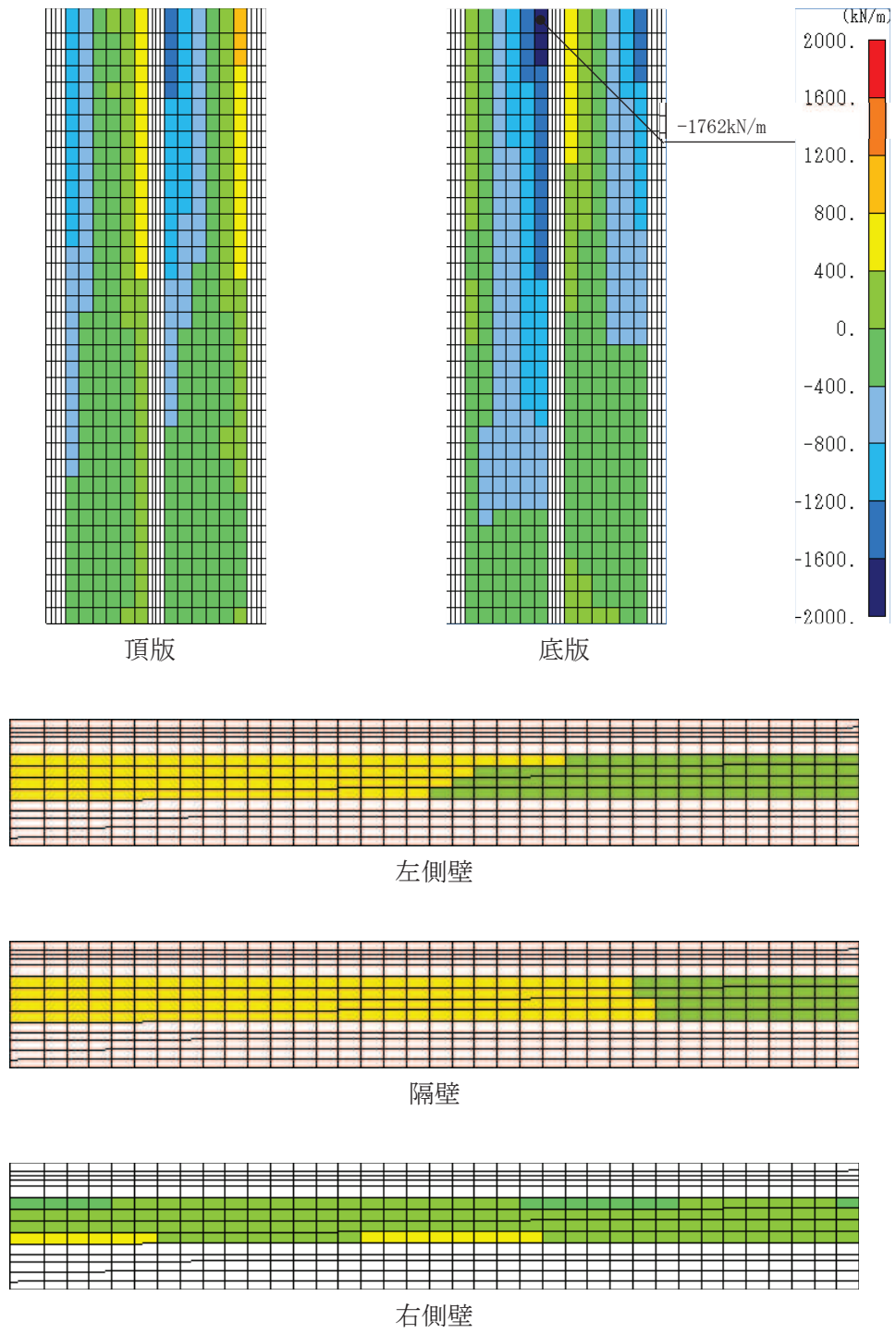
図 4-30 せん断破壊に対する照査における照査値最大時の断面力分布図 (せん断力 (kN/m) : Qx) (直線部, 底板, 解析ケース④', S s -F3 (++) )
