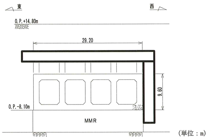
図 2-3 取水路（漸拡部）断面図（A-A 断面）
