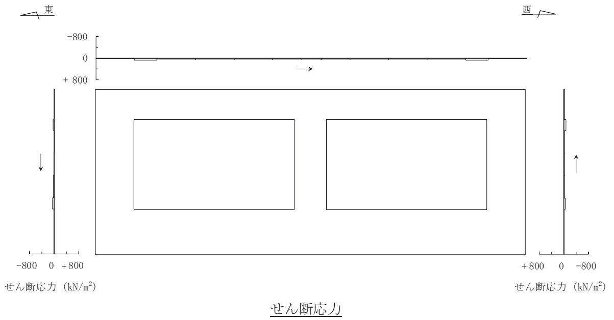
図 3-134 作用荷重分布図 (直応力及びせん断応力) (断面⑦ : 曲線部, 解析ケース③, S s -N1 (++) )
