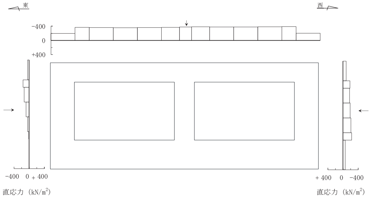
直応力
