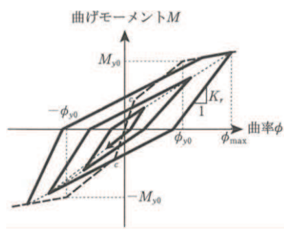
図 3-4 鉄筋コンクリート部材の履歴特性（修正武田モデル）
