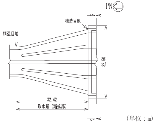
図3-1 取水路（漸拡部）の評価対象断面位置図
