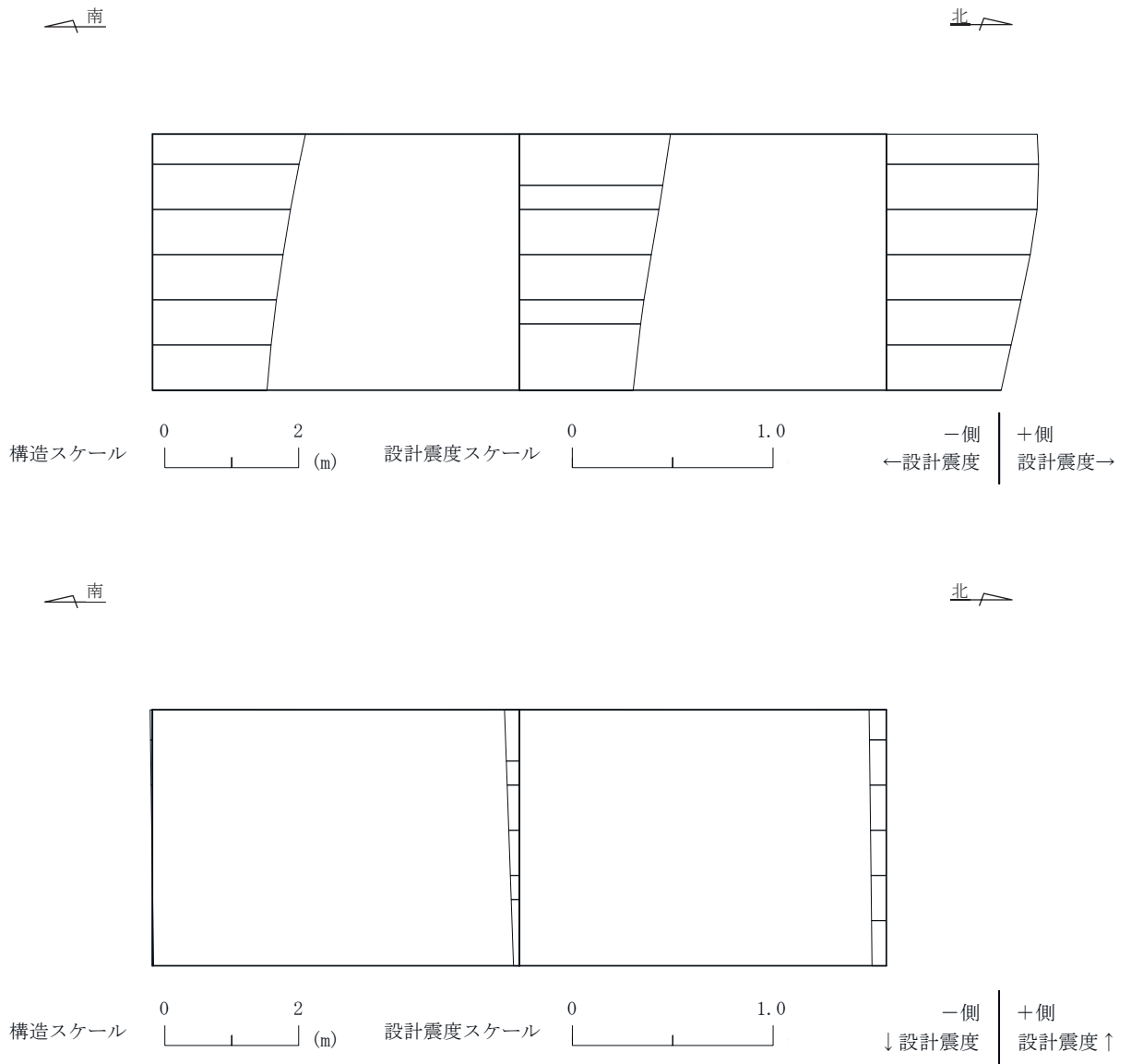
図 3-123 作用荷重分布図 (設計震度分布) (断面⑤: 直線部, 解析ケース③, S s -N1 (++) )
