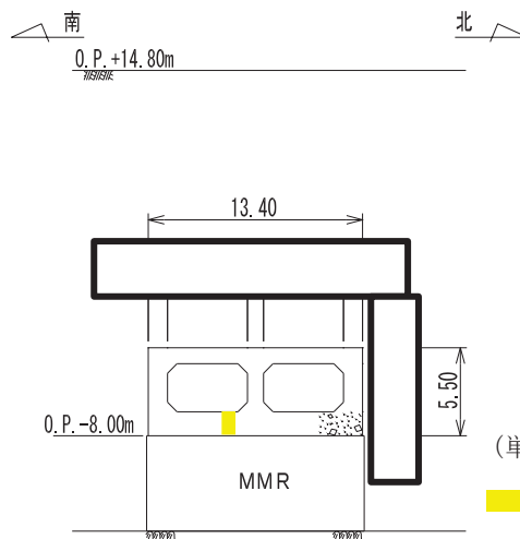
図 2-4(4) CCbによる耐震補強箇所 (③断面, 曲線部; 海水ポンプ室側)
