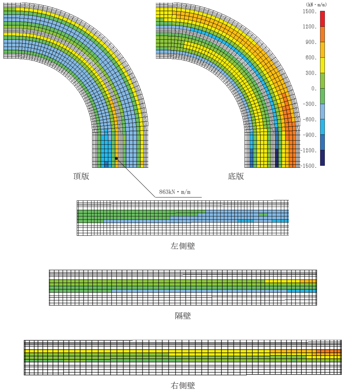
図 4-32 せん断破壊に対する照査における照査値最大時の断面力分布図
