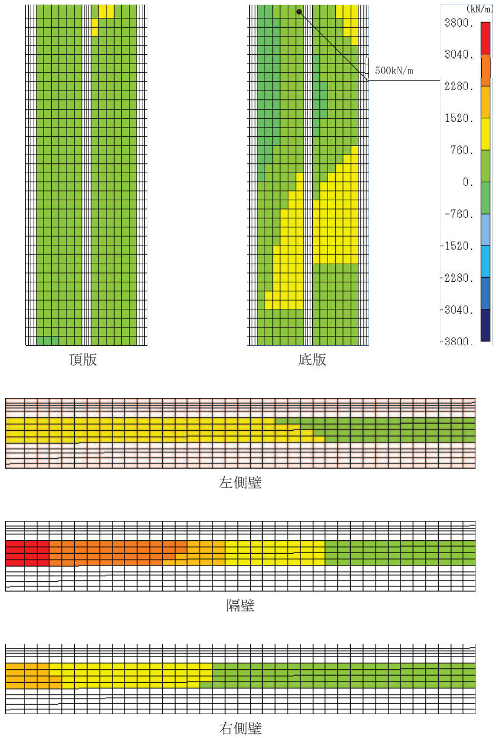
図 4-28 せん断破壊に対する照査における照査値最大時の断面力分布図 (軸力 (kN/m) : Nx) (直線部, 底板, 解析ケース④', S s - F 3 (++)
