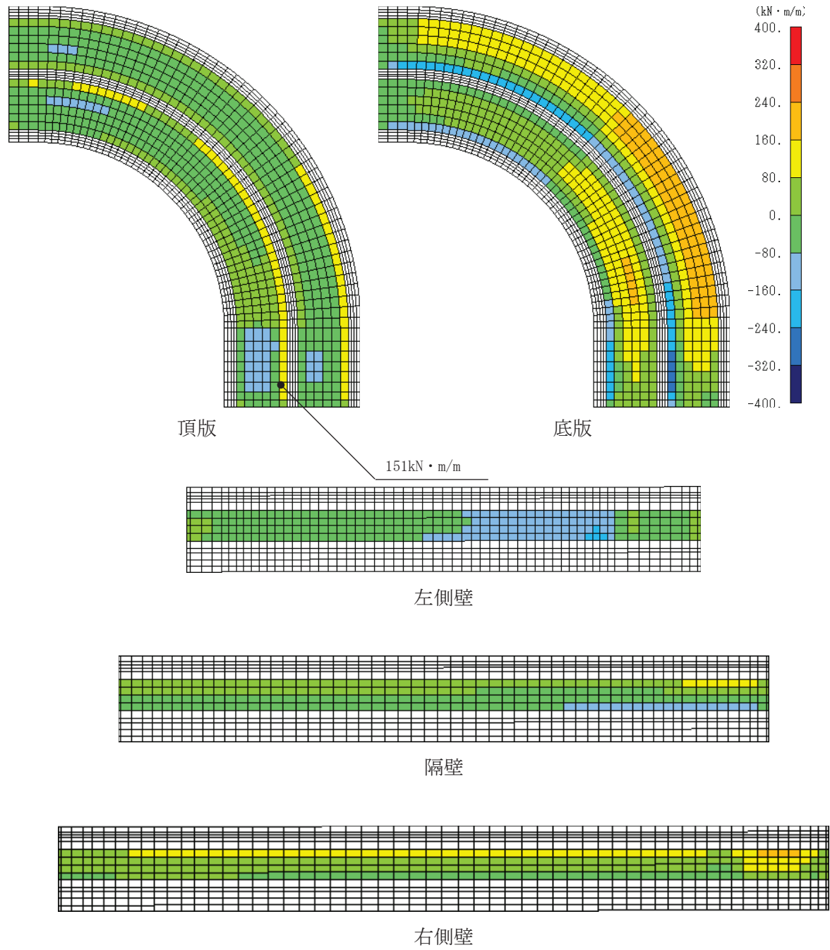
図 4-33 せん断破壊に対する照査における照査値最大時の断面力分布図
