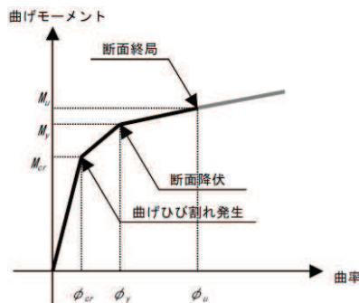
図3-3 鉄筋コンクリート部材のM- \phi 関係
