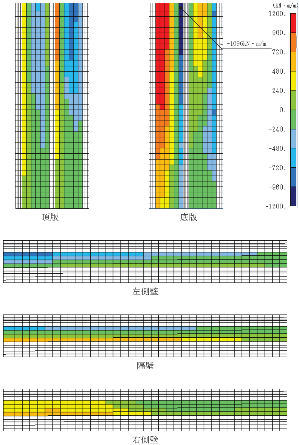
図 4-26 せん断破壊に対する照査における照査値最大時の断面力分布図 (曲げモーメント ( \text{kN} \cdot \text{m}/\text{m} ) : M_x ) (直線部, 底板, 解析ケース④', S_s - F 3 (++)
