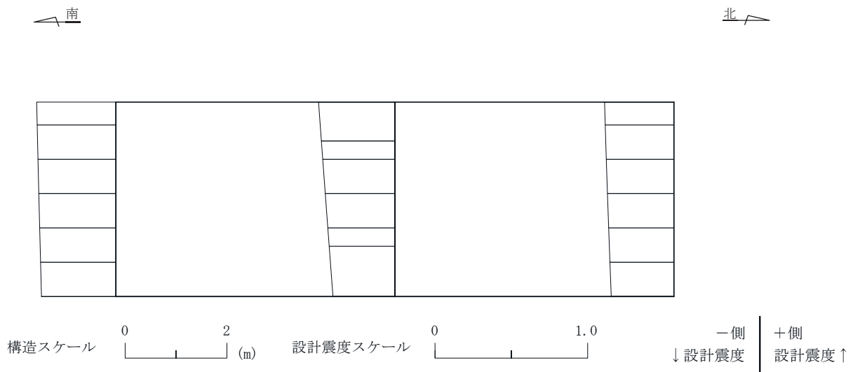
図3-111 作用荷重分布図（設計震度分布） （断面②：直線部，解析ケース③，S s -N1（++））
