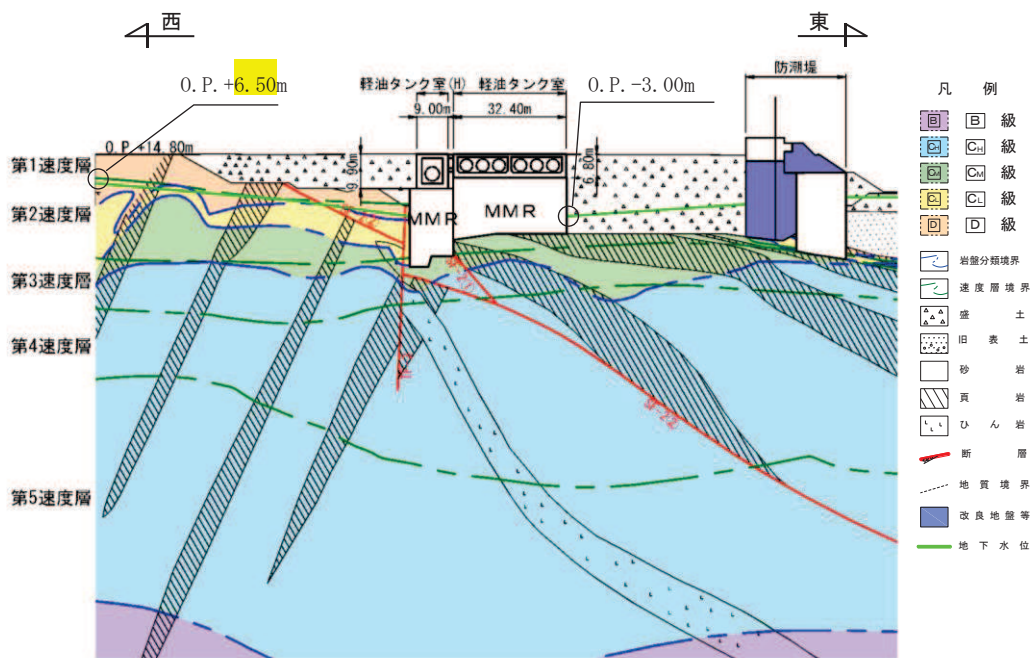
図 3-36 設計用地下水位 (東西)
