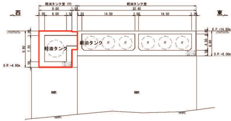
図 2-4 軽油タンク室 (H) 断面図 (B-B 断面, 東西)
