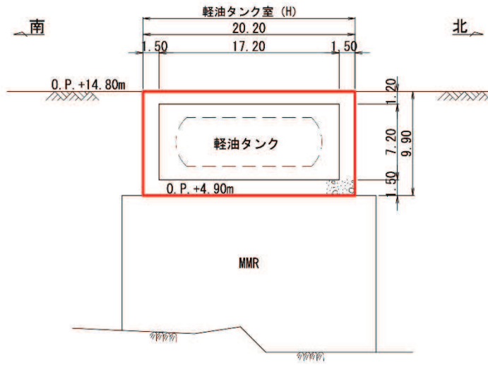
図 2-3 軽油タンク室 (H) 断面図 (A-A 断面, 南北)
