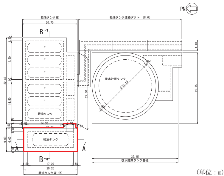
図 3-1 軽油タンク室 (H) の地震時荷重算出断面位置図
