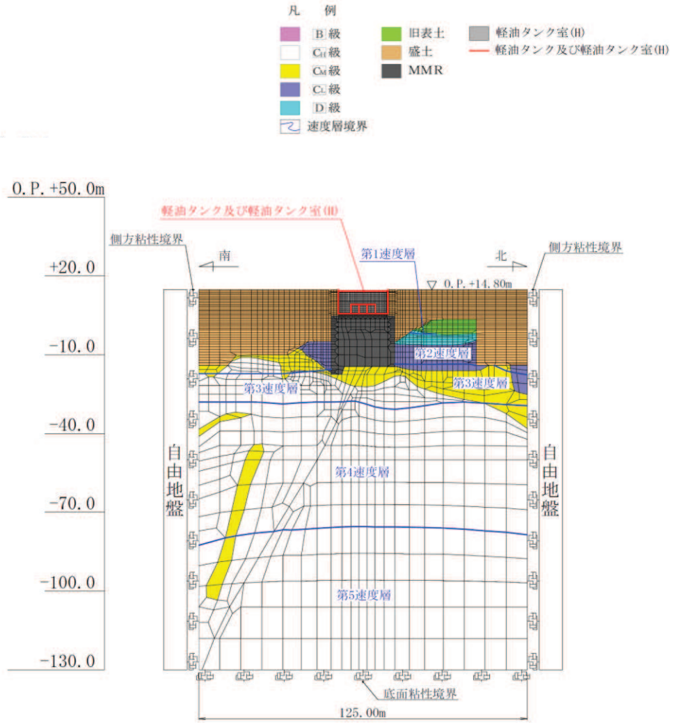
図 3-33 軽油タンク室 (H) の地震応答解析モデル図 (南北方向)
