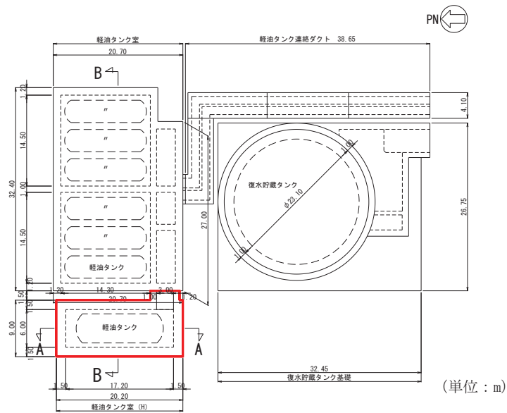
図 2-2 軽油タンク室 (H) 平面図
