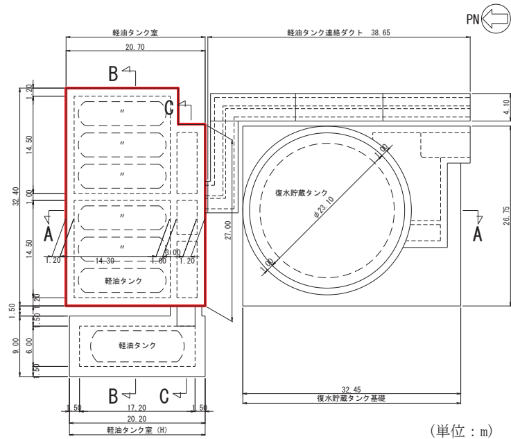
図 3-1 軽油タンク室の地震時荷重算出断面位置図
