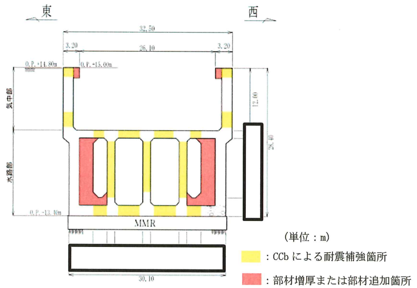
図 2-11 補強計画図 (B-B 断面, 東西 (補機ポンプエリア))
