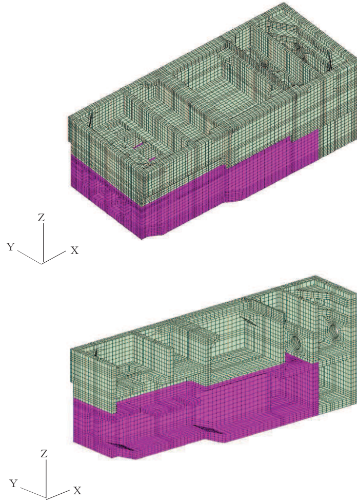
図 5-5 通水機能が要求される部材の範囲
