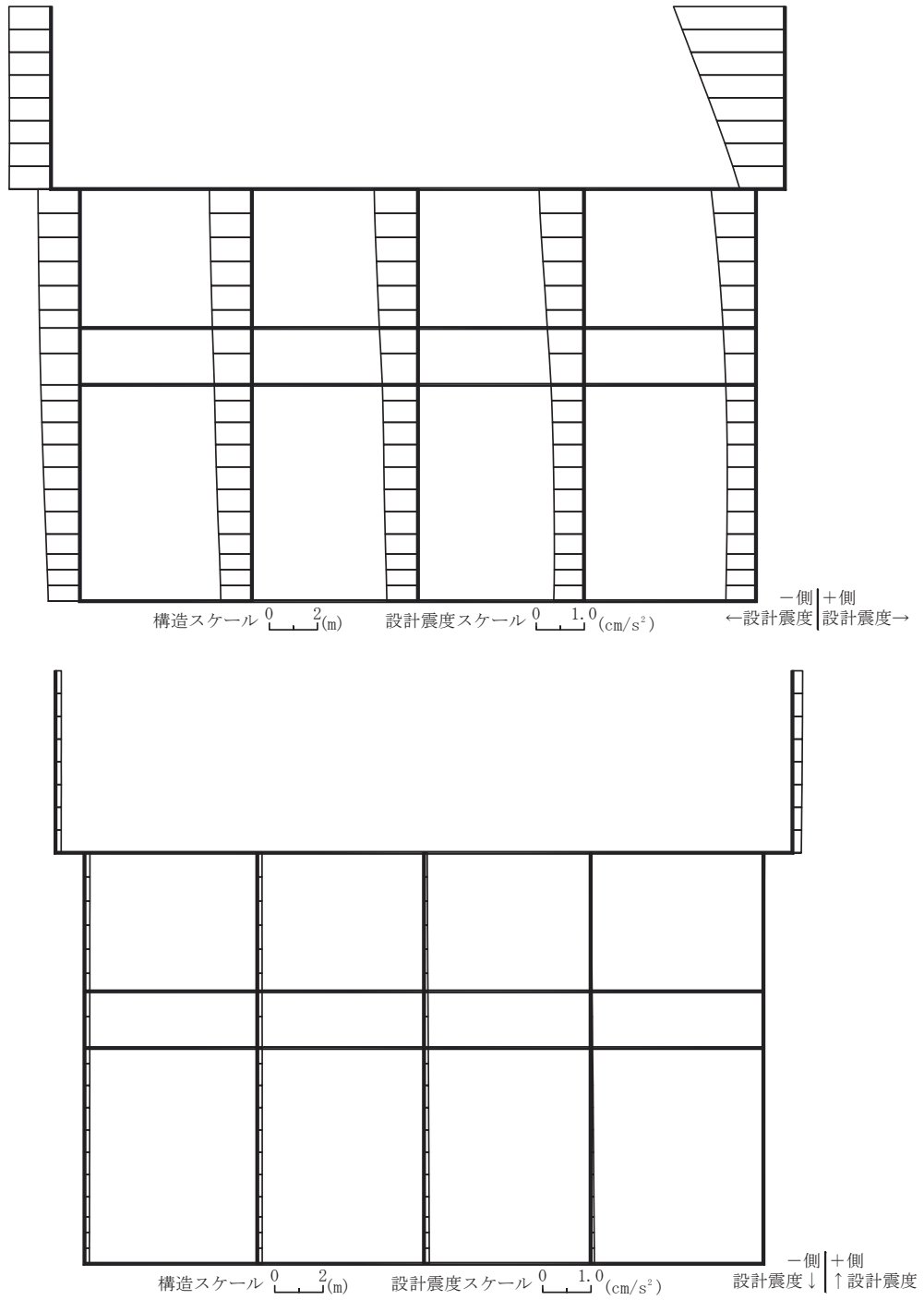
図 3-14 作用荷重分布図 (設計震度分布) (解析ケース③, S s - N 1 (++) , A-A 断面, 東西 (スクリーンエリア))
