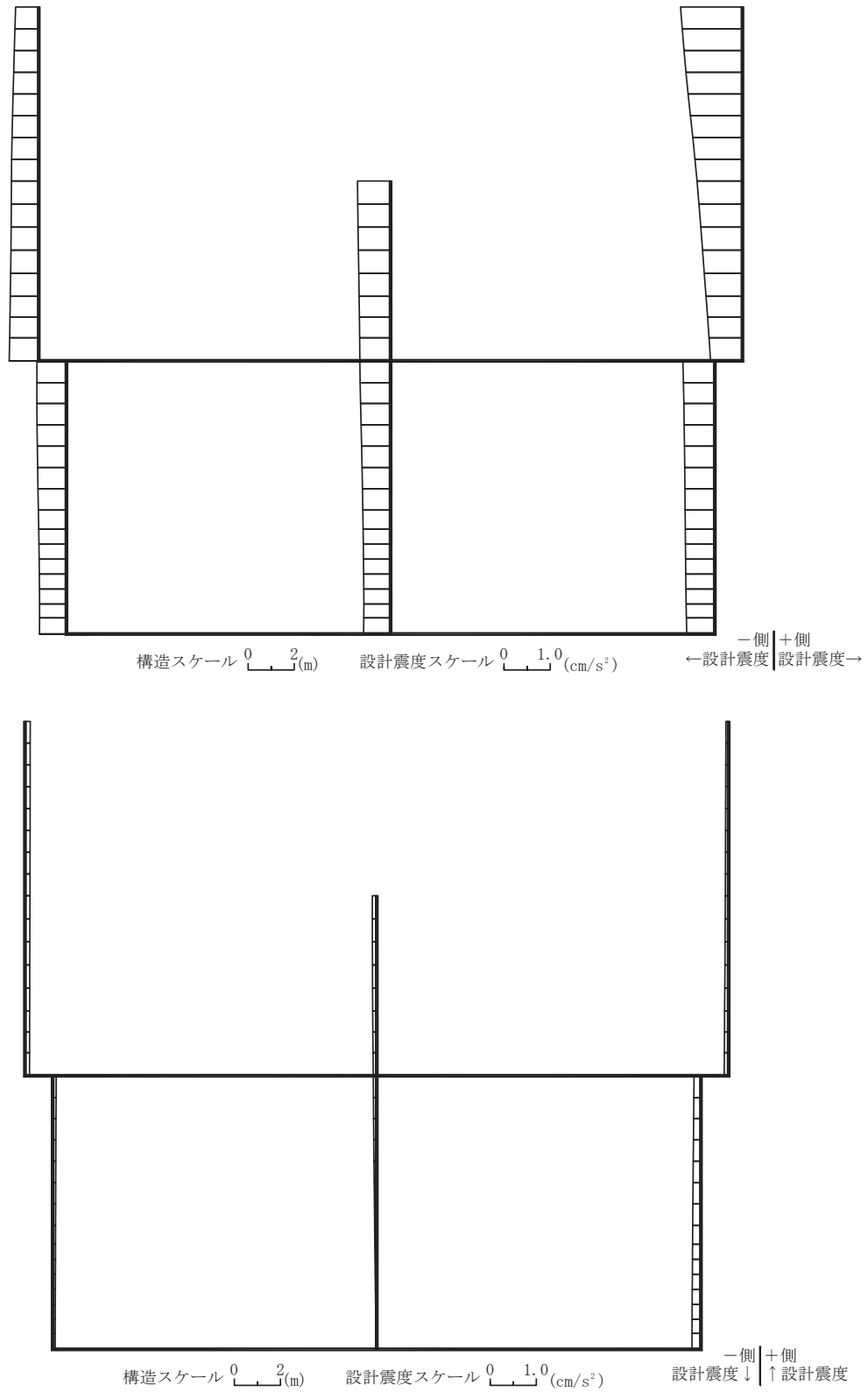
図 3-18 作用荷重分布図（設計震度分布） （解析ケース③，S s - N 1（++），C-C 断面，東西（循環水ポンプエリア））
