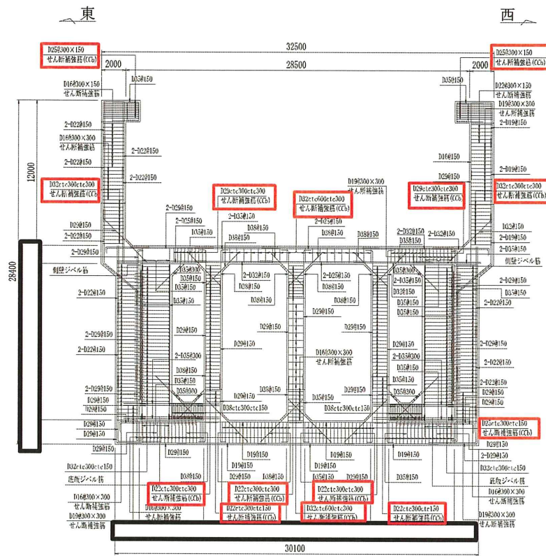
図 2-16 海水ポンプ室概略配筋図 (B-B 断面, 東西 (補機ポンプエリア))
