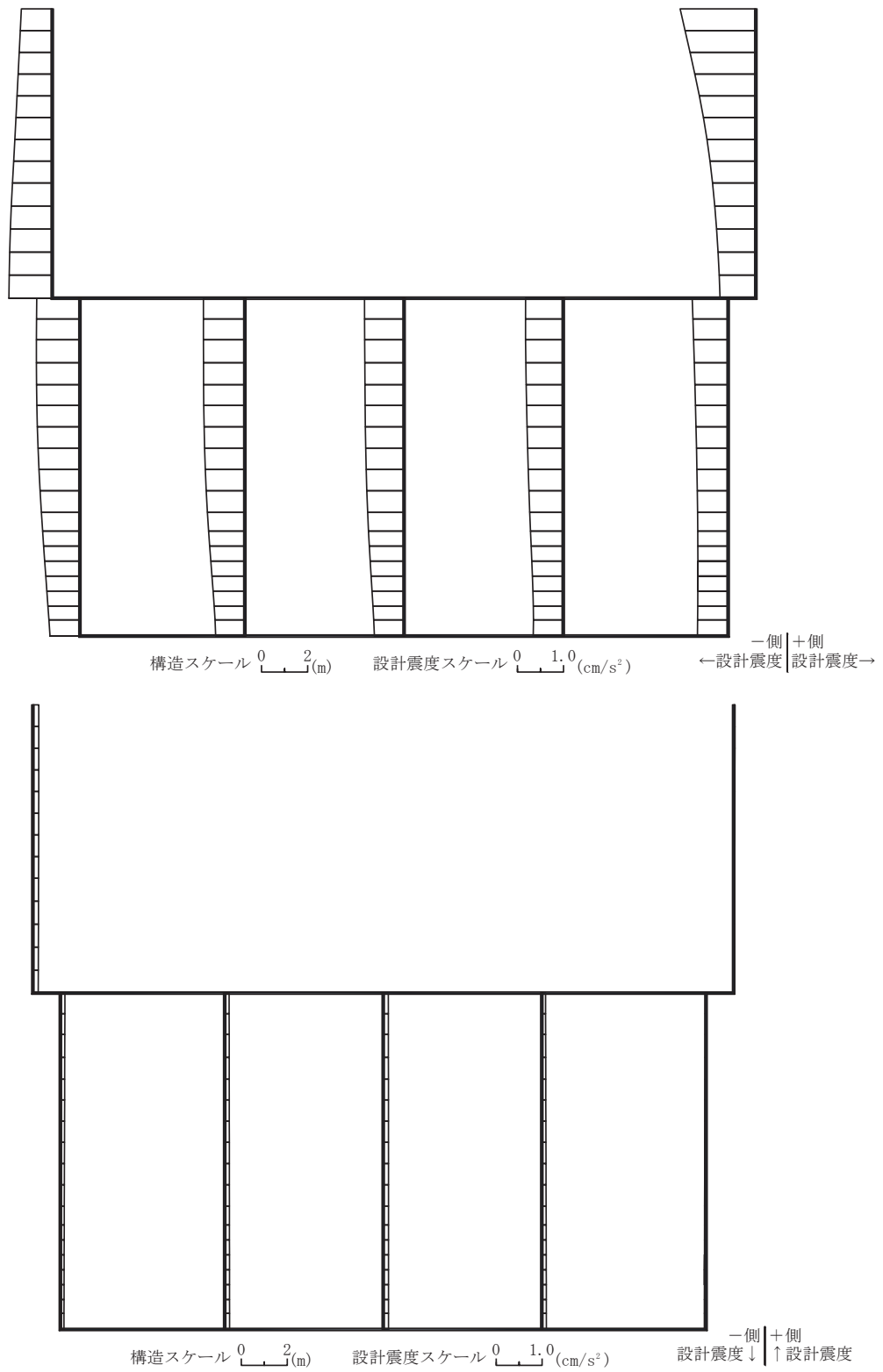
図 3-16 作用荷重分布図 (設計震度分布) (解析ケース③, S s - N 1 (++) , B-B 断面, 東西 (補機ポンプエリア))
