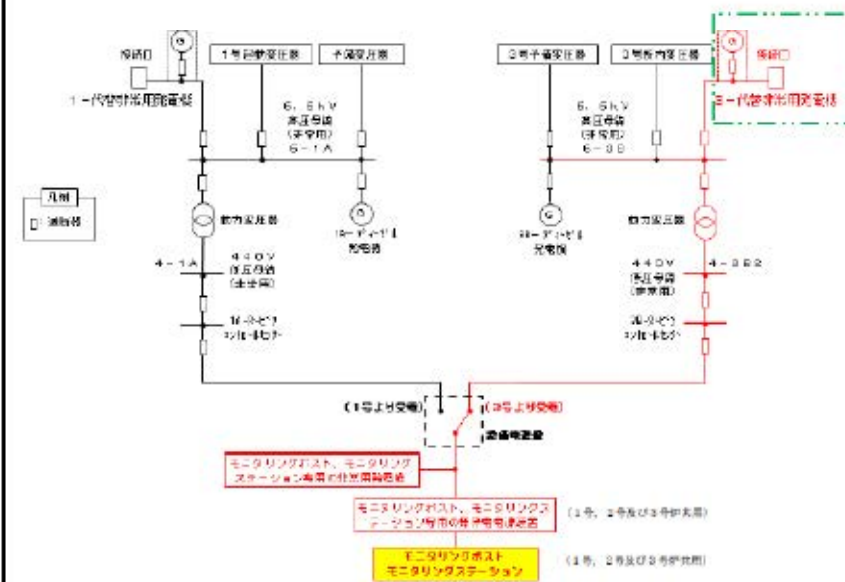
図7 モニタリングポストおよびモニタリングステーションの電源
