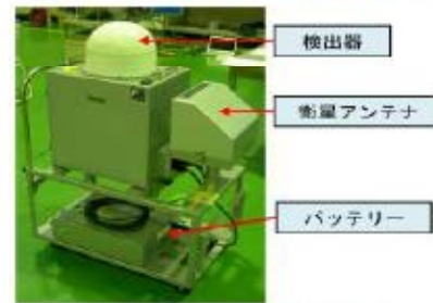
図6 可搬型モニタリングポストの外観
