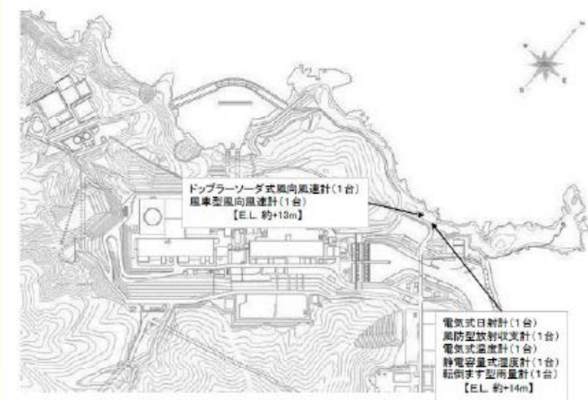
図3-1 気象観測設備の配置図
