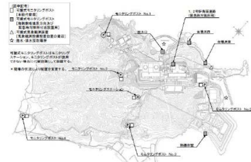
図2-3-1 モニタリング設備の配置場所及び試料採取場所
