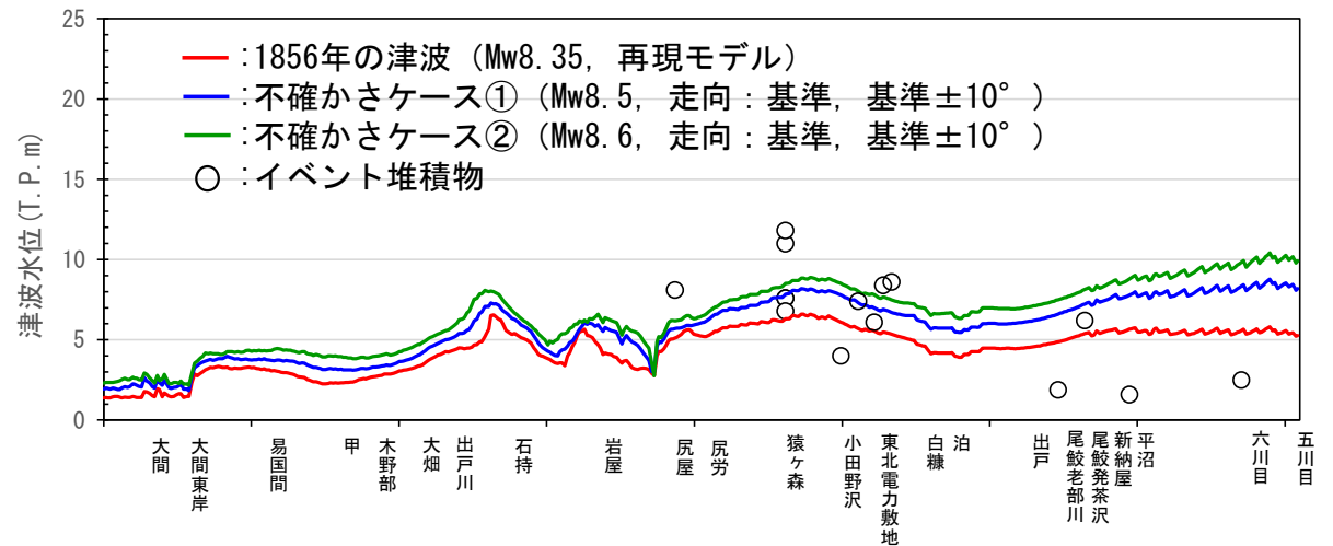
海岸線位置における想定津波群(空間格子間隔278m)とイベント堆積物の比較
