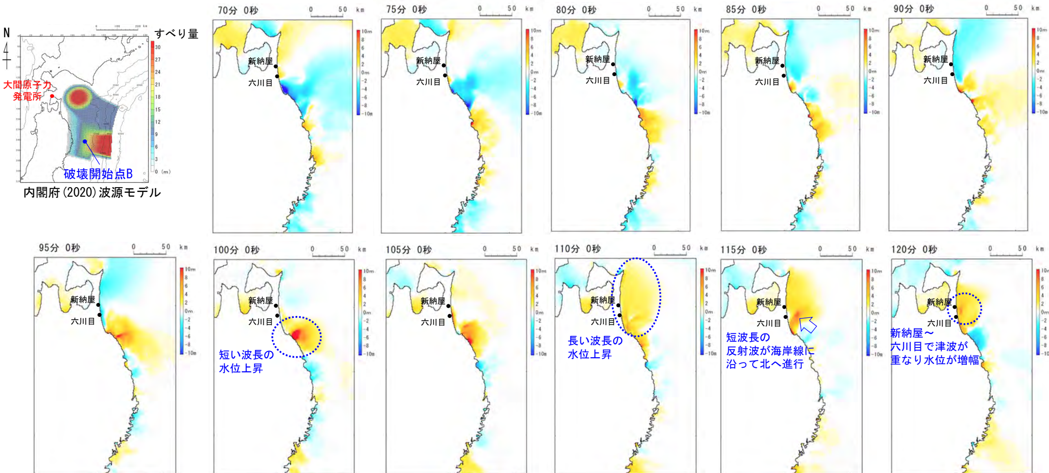
下北半島周辺の津波伝播スナップショット (内閣府(2020a) (102) モデル)
