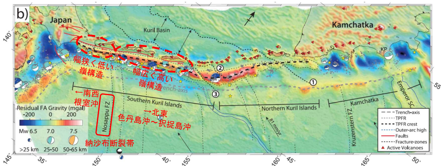
千島～カムチャッカ沈み込み帯 Bassett and Watts (2015) (147) に一部加筆 (コンターは重力異常の短波長成分, 黒破線はTPFRの嶺, 灰色破線は海溝軸を表す。)
