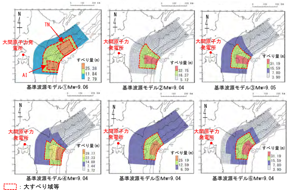
想定津波群作成ケース
