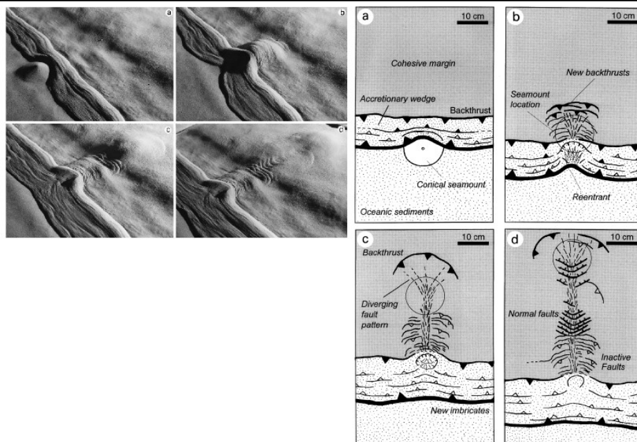
砂箱を用いた実験に基づく沈み込む海山による陸側斜面の変形構造 (左: 実験, 右: 模式図) Dominguez et al. (1998) (164)
