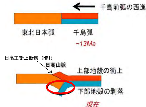
千島弧の前弧スリパーの西進、東北日本弧との衝突による日高山脈形成過程の模式図 日野ほか (2008) (145)に一部加筆
