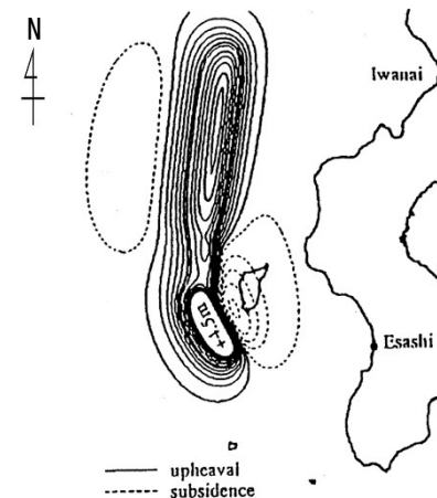
1993年北海道南西沖地震津波 断層モデル 高橋ほか (1995) (46) に一部加筆
