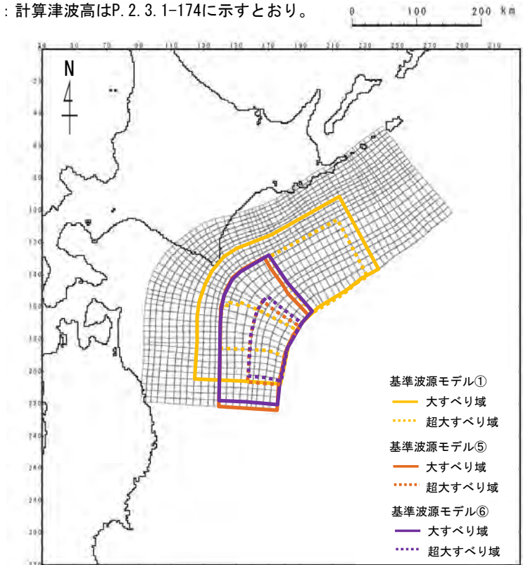
アスぺリティの位置を変化させる概略パラメータスタディで上昇側最大ケースとなった各基準波源モデルの大すべり域等の位置図
