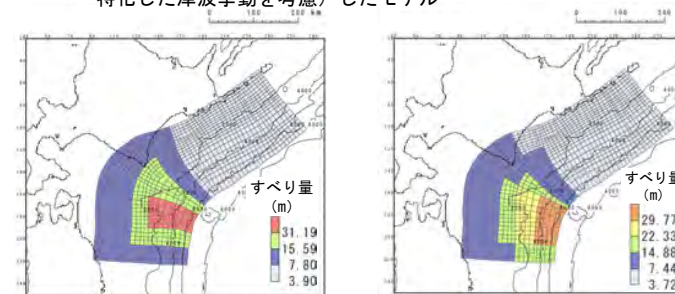
基準波源モデル③ 基準波源モデル④
