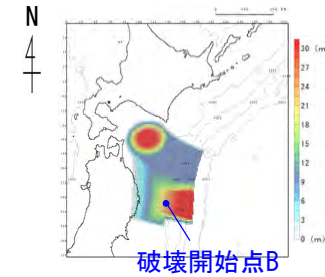
内閣府(2020a) (102) モデル
