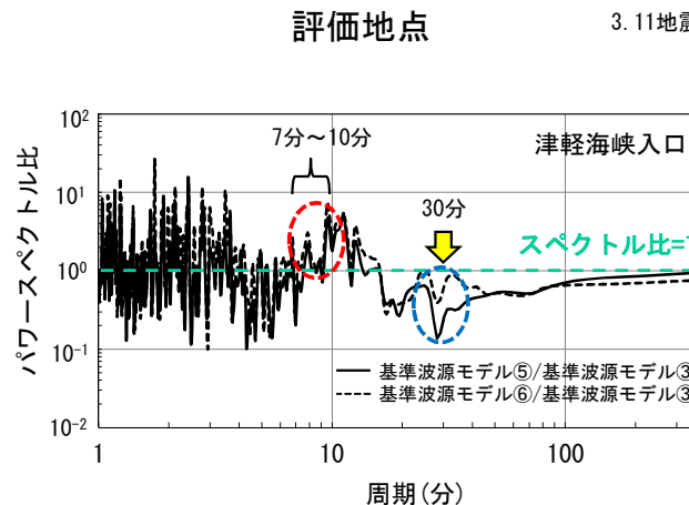
基準波源モデル③と基準波源モデル⑤⑥との比較
