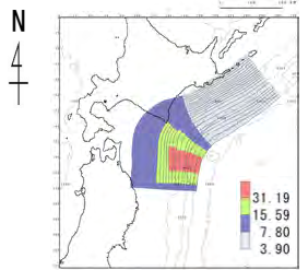
基準波源モデル③
