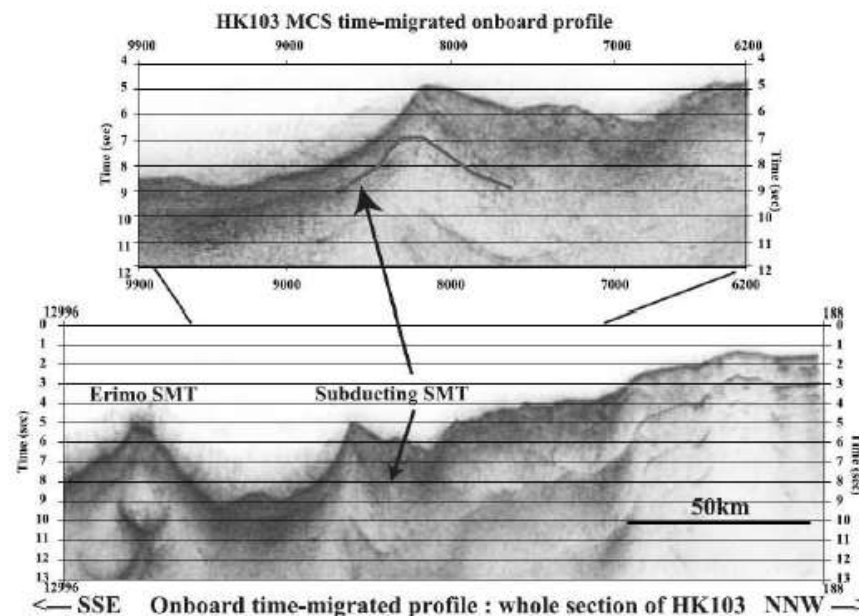
襟裳海山及び沈み込む海山直上のプロファイル (MCS処理記録 (測線: HK103)) 木戸ほか (2002) (163)
