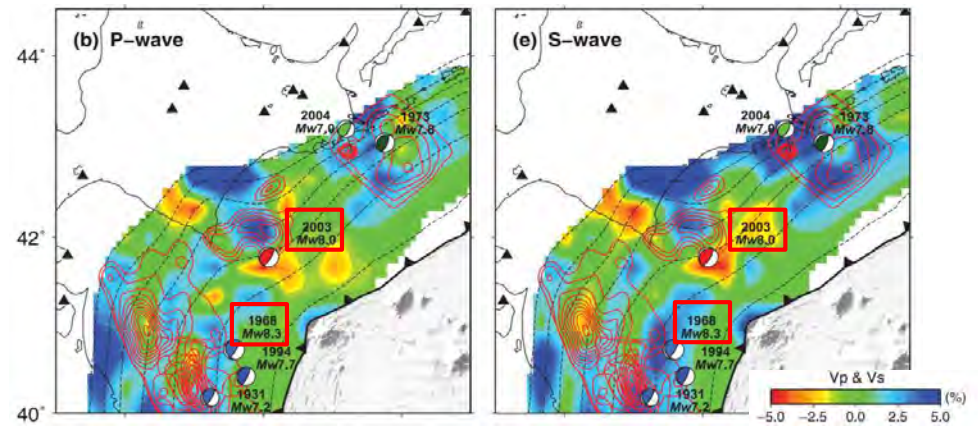
日本海溝・千島海溝島弧改造部付近の地震波トモグラフィと既往地震発生域の関係 Liu et al. (2013) (144)に一部加筆
