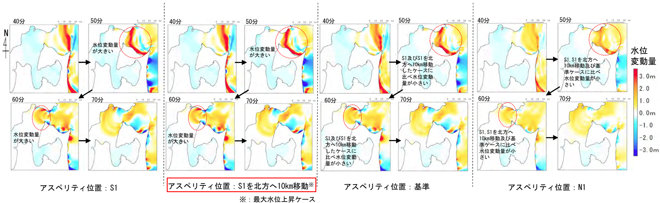
スナップショット \Delta t = 278\text{m} 領域 (地震発生40分後～70分後)
