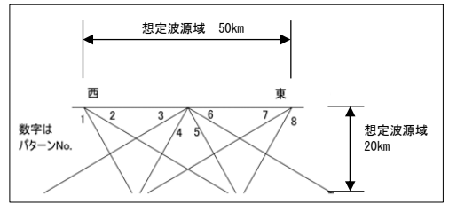
東西位置、傾斜角パターン 土木学会 (2016) (39) に一部加筆
