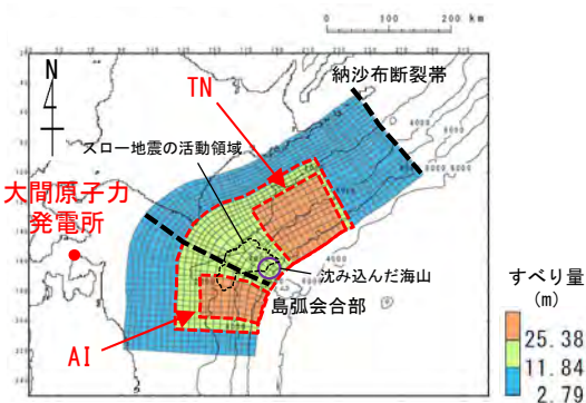
基準波源モデル① 基準配置
