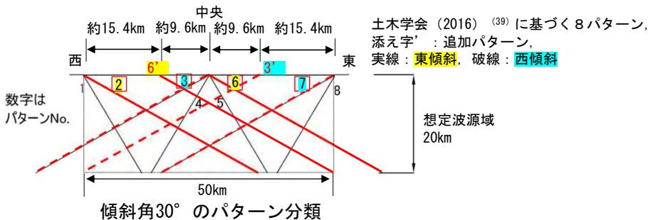
結果一覧 (傾斜角30°)
