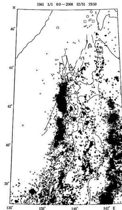
日本海東縁の浅い地震（深さ30km以浅）の震源（1961-2000年）と活断層の分布
