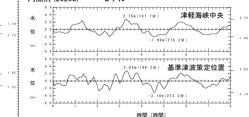
内閣府(2020a) (102) モデル
