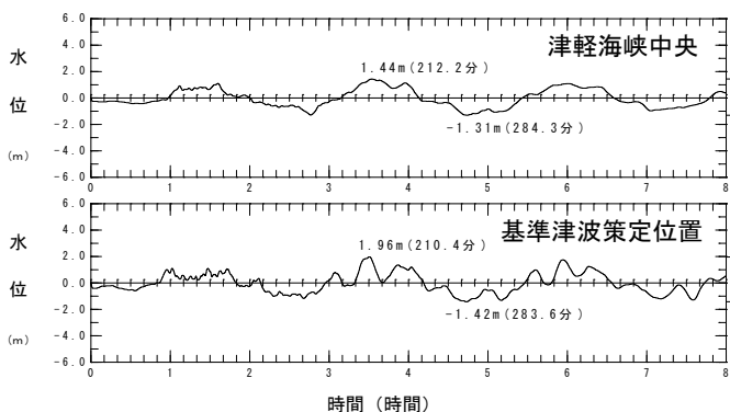
基準波源モデル③
