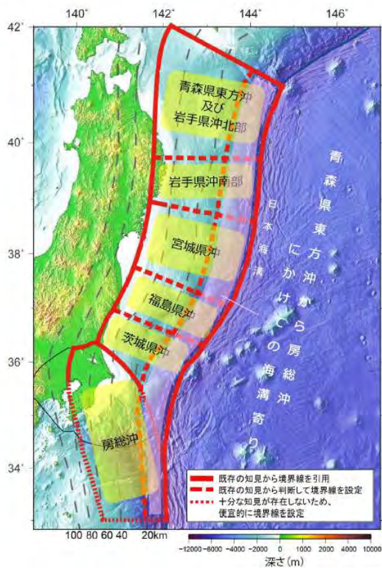
三陸沖から房総沖にかけての評価対象領域の分け 地震調査研究推進本部 (2019) (78)
