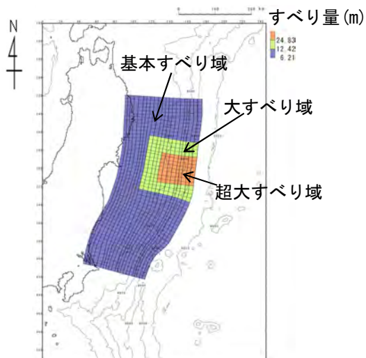
3.11地震における宮城県沖の破壊特性を考慮した特性化モデル
