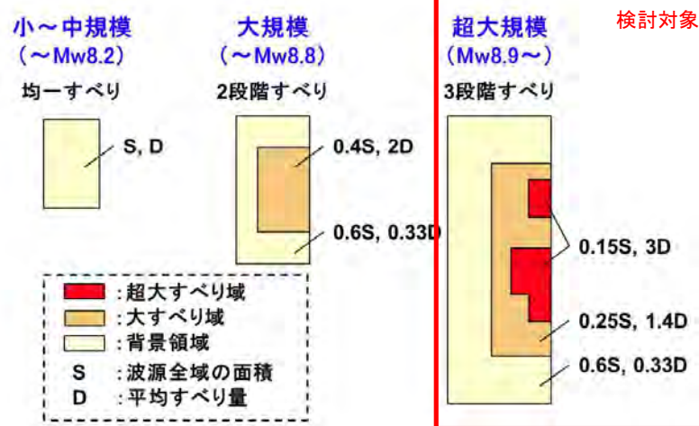
微視的波源特性に係る波源領域内の空間的すべり分布の設定方法 杉野ほか（2014） (130) に一部加筆
