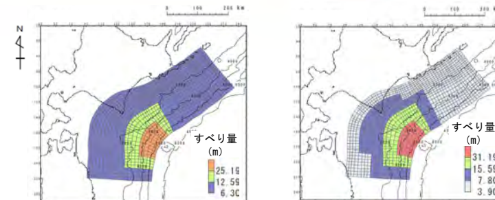
基準波源モデル⑤ 基準波源モデル⑥
