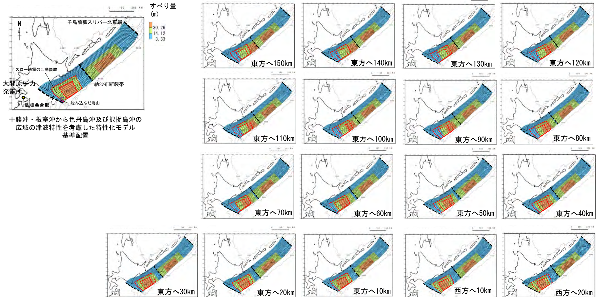
： 標準配置のアスペリティ位置
