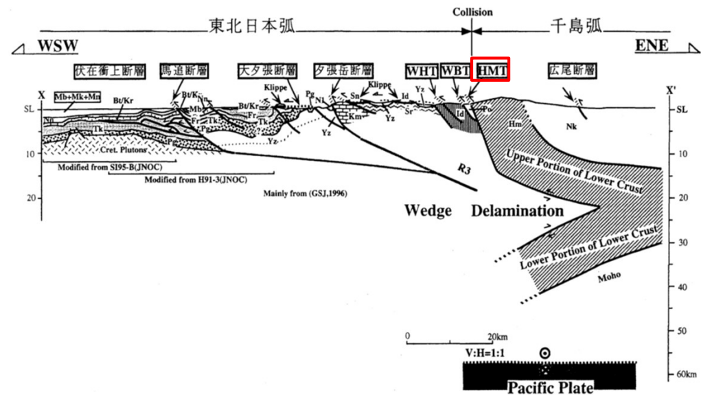
図2 日高衝突帯ならびに前縁褶曲・衝上断層帯の地下構造断面図。断面線の位置は図1のX-X'。断面図下に主要な出典を示した。略称は図1と同じ。Ito et al. (1998) および伊藤ら(1999)を改変。
