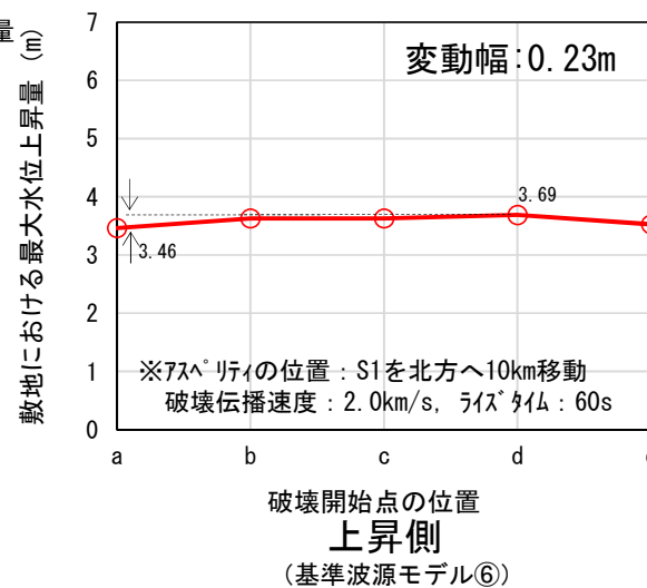
破壊開始点の位置の影響
