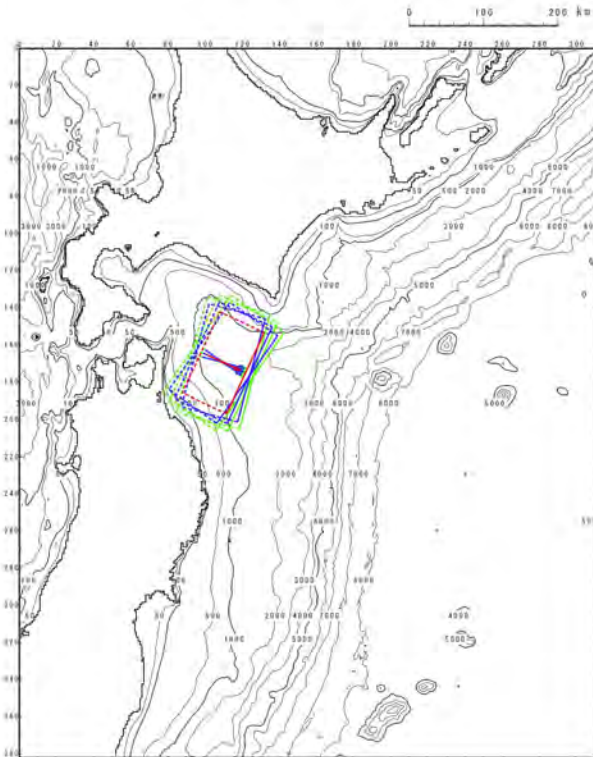
検討波源モデル
