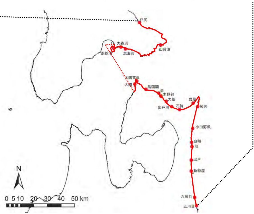
基準波源モデル①~④の計算津波高と太平洋側既往津波高との比較
