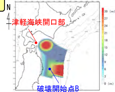
内閣府(2020a) (102) モデル 周期(分)
