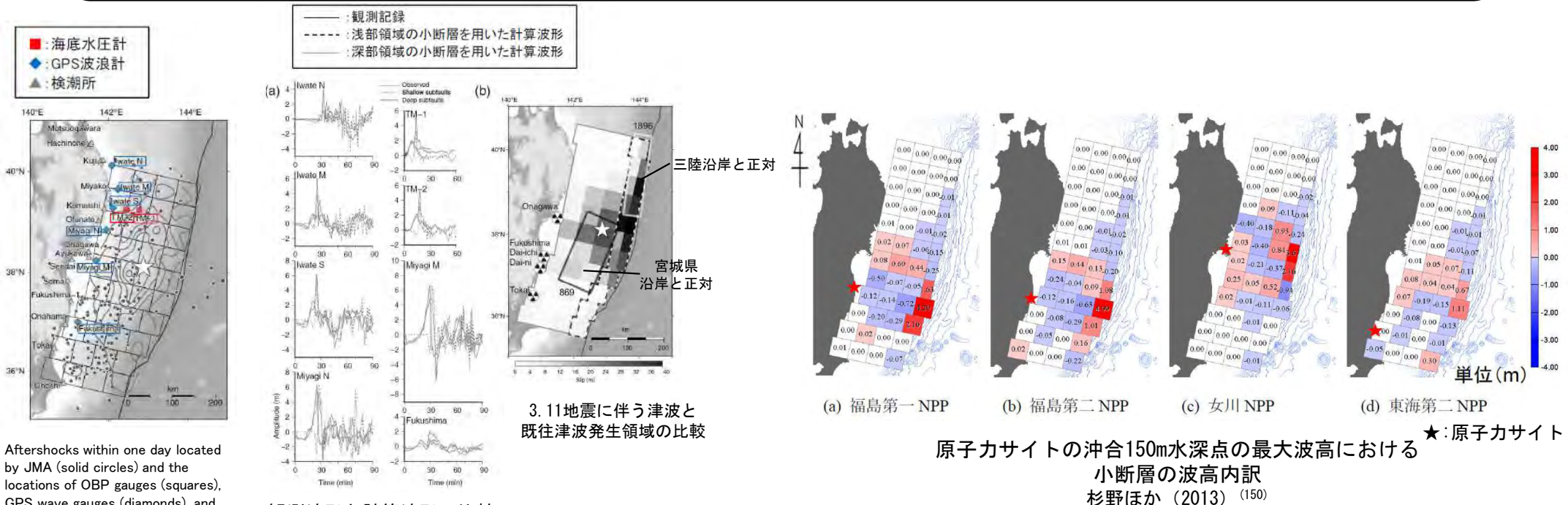
観測波形と計算波形の比較
