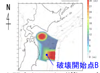
内閣府(2020a) (102) モデル
