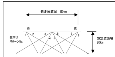
東西方向位置・傾斜角及び傾斜方向パターン 土木学会 (2016) (39) に一部加筆
