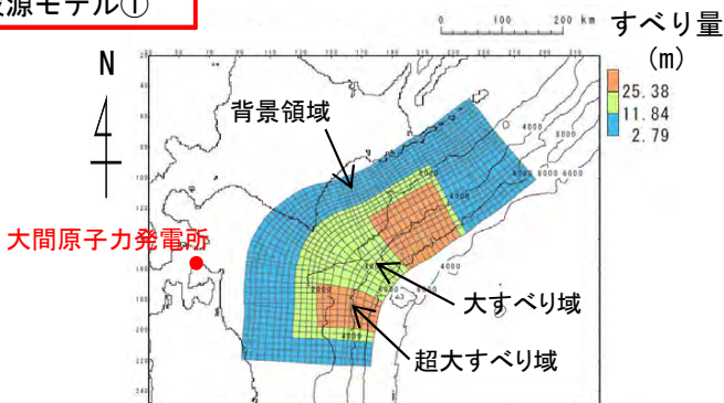
基準波源モデル①
