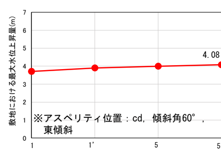
東西方向位置・傾斜角及び傾斜方向パターン
