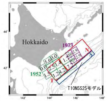
17世紀に発生した超巨大地震に伴う津波の再現モデル (Ioki and Tanioka (2016) (153) によるT10N5S25モデル) 地震調査研究推進本部 (2017a) (129) に一部加筆
