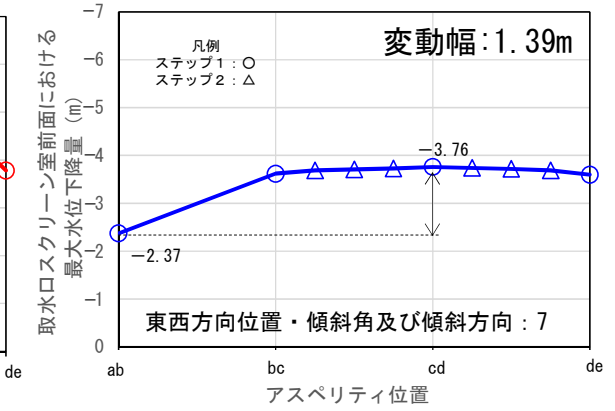
アスペリティ位置の影響
