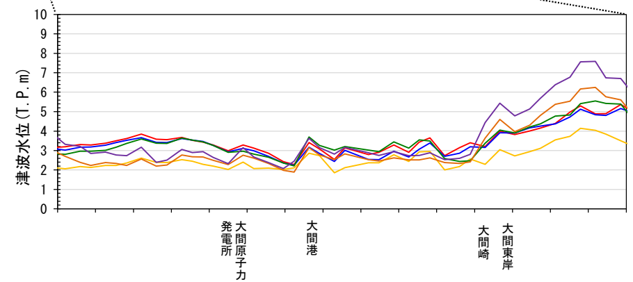
津軽海峡開口部付近沿岸における基準波源モデル①～⑥の想定津波群とイベント堆積物の比較
