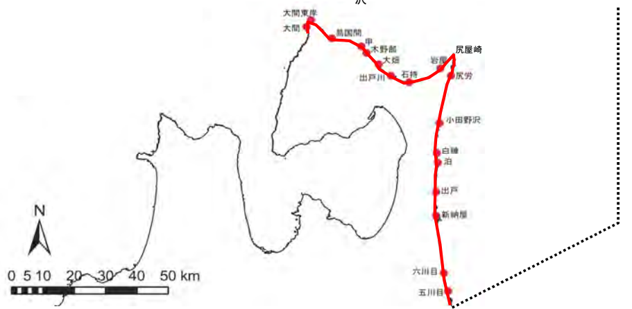
津軽海峡開口部付近沿岸における基準波源モデル①～⑥と内閣府(2020a) (102) モデルの想定津波群との比較
