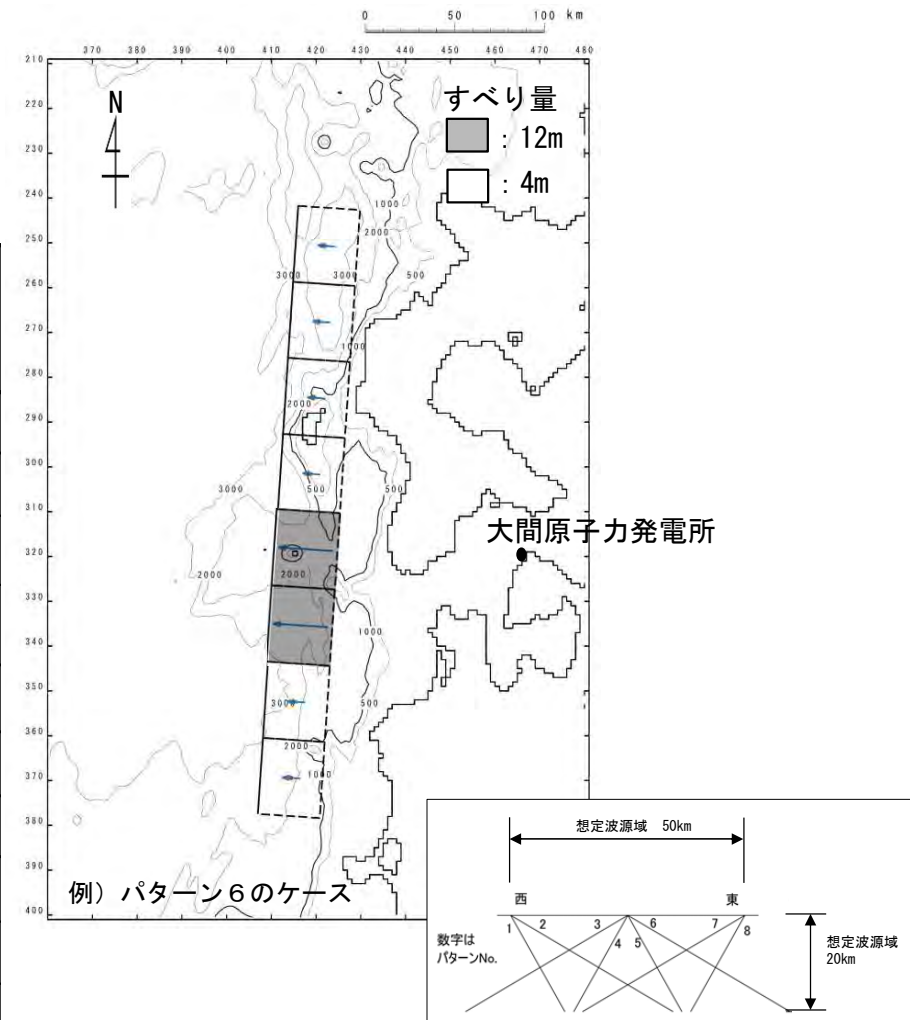
東西位置, 傾斜角パターン 土木学会(2016) (39) に一部加筆 基準波源モデル
