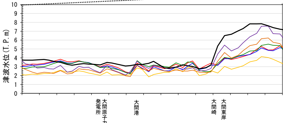
津軽海峡開口部付近沿岸の海岸線位置における基準波源モデル①～⑥と内閣府(2020a) (102) モデルの想定津波群との比較(大間周辺)
