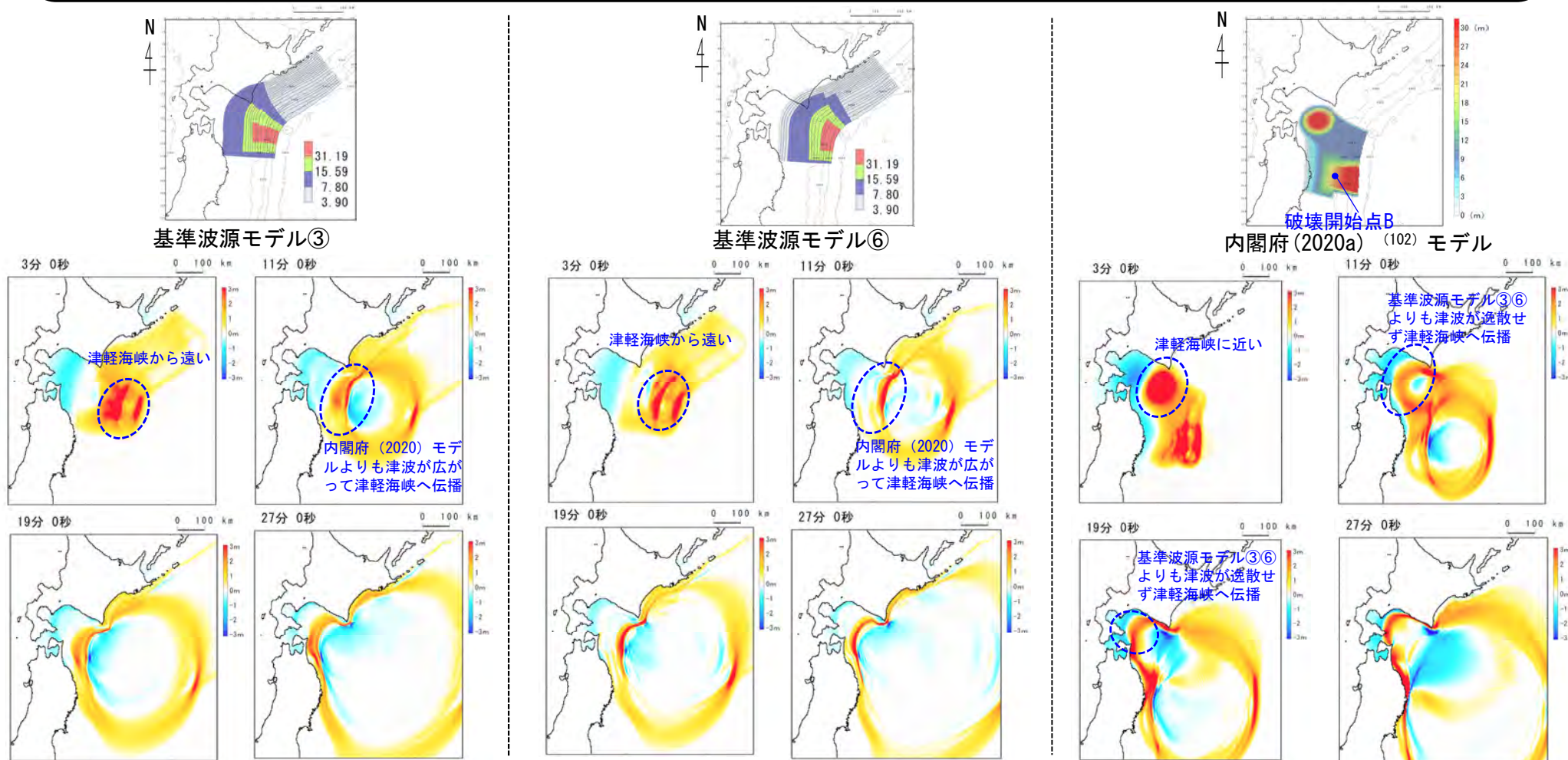
波源域からの津波伝播スナップショット (基準波源モデル③と⑥を例示)
