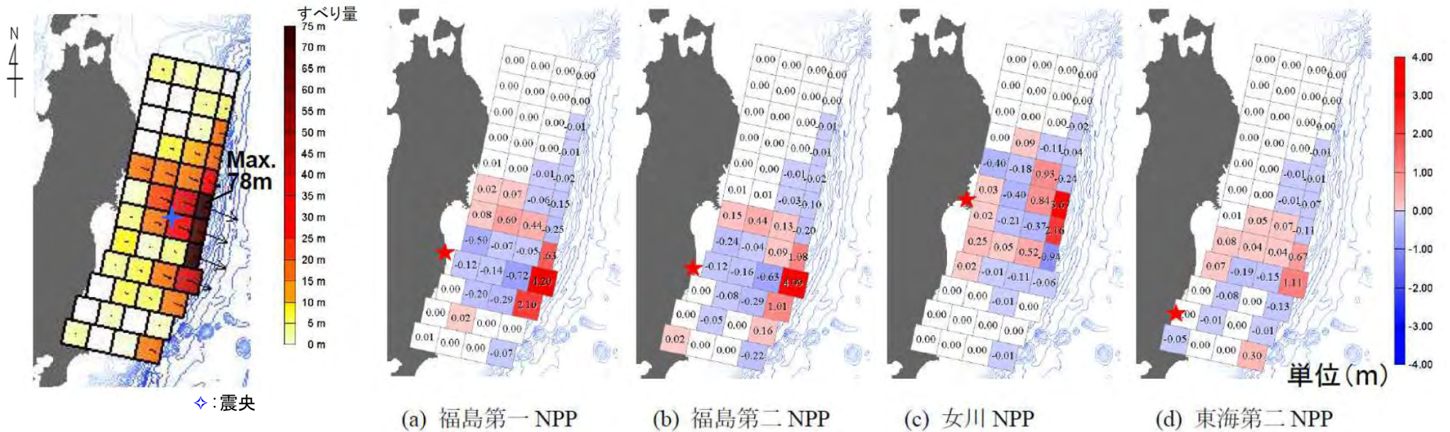
原子力サイトの沖合150m水深点の最大波高における小断層の波高内訳 杉野ほか (2013) (150)
