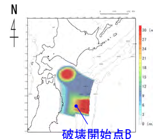
内閣府(2020a) (102) モデル
