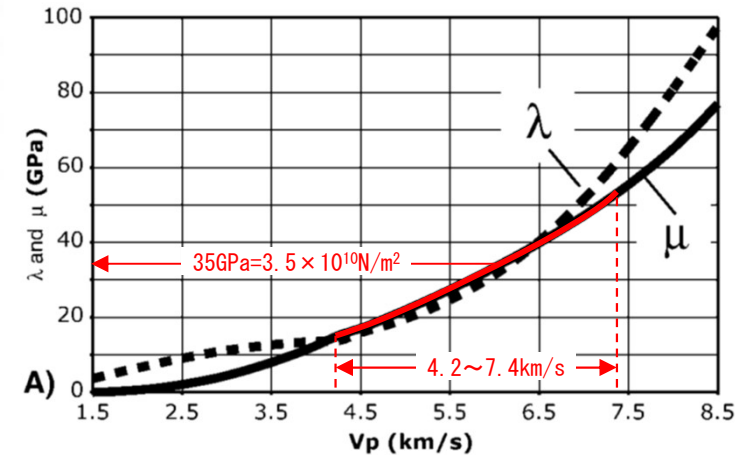
Brocher (2005) (75) に一部加筆
