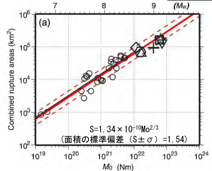
破壊領域 (S) と Mo の関係 Murotani et al. (2013) (110) に一部加筆
