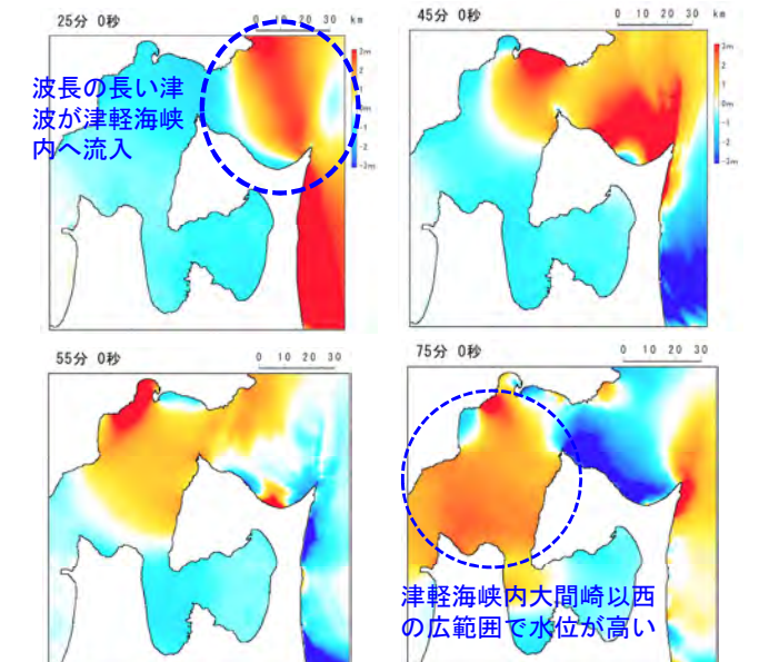
津軽海峡内の津波伝播スナップショット (内閣府(2020a) (102) モデル)
