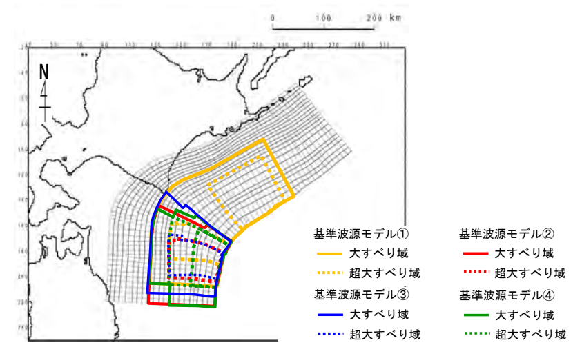
概略パラメータスタディで上昇側最大ケースとなった各基準波源モデルの大すべり域等の位置図
