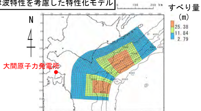
岩手県沖北部から十勝沖・根室沖の広域の津波特性を考慮した特性化モデル
