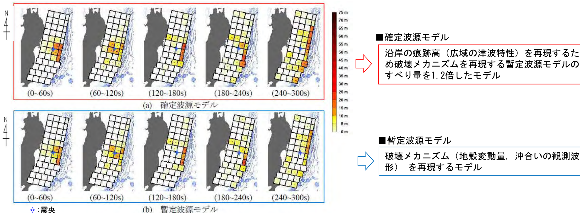
3.11地震を再現する津波波源モデルのすべり分布の経時変化 杉野ほか (2013) (150) に一部加筆
