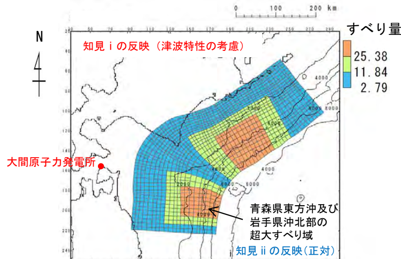
岩手県沖北部から十勝沖・根室沖の 広域の津波特性を考慮した特性化モデル (P. 2. 3. 1-67)
