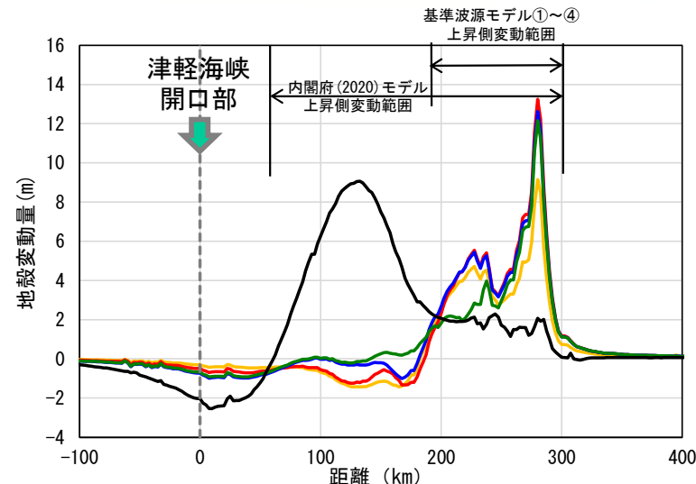
地盤変動量断面図 (基準波源モデル①～④, 内閣府(2020a) (102) モデル)
