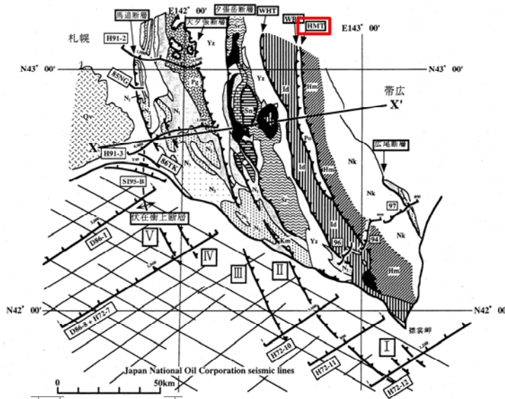
図1 日高衝突帯ならびに前縁褶曲・衝上断層帯の地質概略と主な反射法地震探査測線。X-X'は図2の断面位置を示す。伊藤ら(1999)を改変。 【地質】主として、地質調査所(1982, 1996)による。Nk: 中の川層群, Hm: 日高変成岩類(主帯), Po: ボロシリ・オフィオライト(西帯), Id: イドンナップ帯, Yz: 蝦夷層群, Sr: 空知層群, Km: 神威古潭変成岩類, Sn: 沙流川層一セウ層, Pg: 古第三系, N1~N3: 地質調査所(1982)と同じ。Qv: 第四紀火山岩類, HMT: 日高主衝上断層, WBT: 西縁衝上断層, WHT: 日高西部断層群 【測線】④4・96・97: 日高深部構造反射法探査, 85NG・86TK: 浅野ら(1990), Y97: 佐藤ら(1998), その他の測線は石油公団(1973, 1987, 1993, 1996)。
