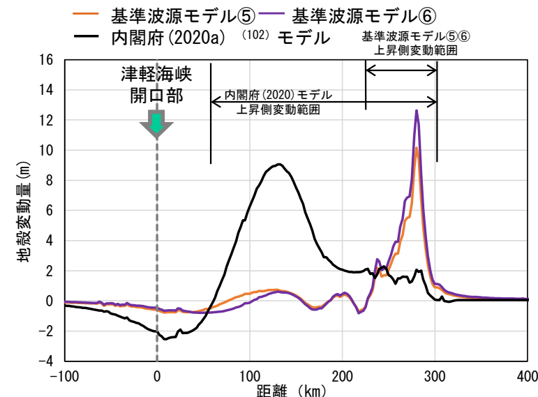
地盤変動量断面図 (基準波源モデル⑤⑥, 内閣府(2020a) (102) モデル)
