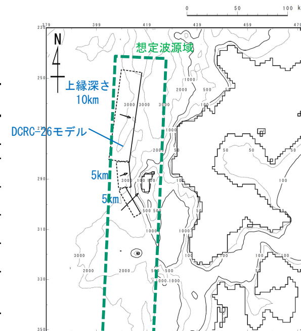
1993年北海道南西沖地震波源モデル (DCRC-26モデル) と想定波源域
