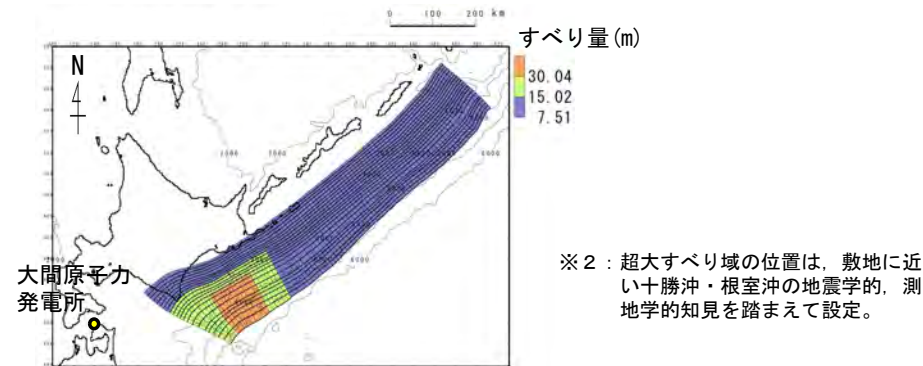
十勝沖・根室沖から色丹島沖及び択捉島沖の破壊特性を考慮した特性化モデル※2
