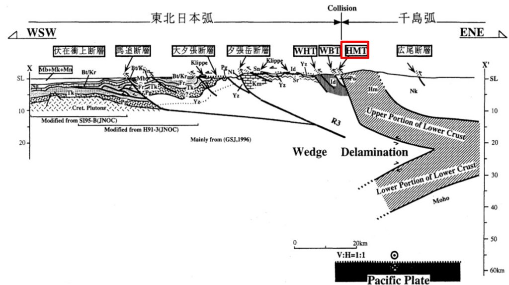
図2 日高衝突帯ならびに前縁褶曲・衝上断層帯の地下構造断面図。 断面線の位置は図1のX-X'。断面図下に主要な出典を示した。略称は図1に同じ。Ito et al. (1998) および伊藤ら(1999)を改変。 伊藤(2000) (142) に一部加筆
