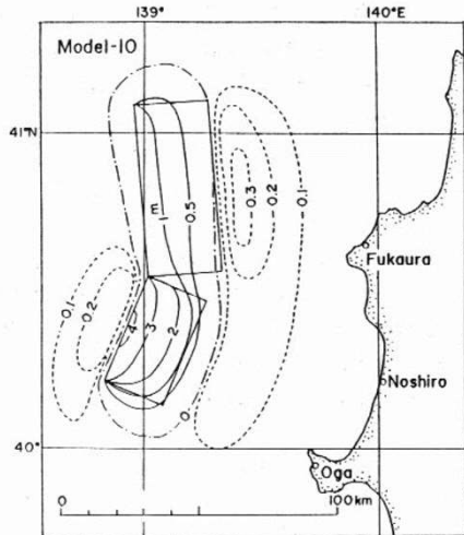
1983年日本海中部地震津波 断層モデル 相田 (1984) (76) に一部加筆
