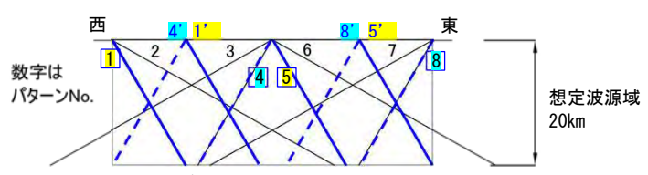
傾斜角60°のパターン分類 土木学会 (2016) (39) に基づく8パターン、 添え字' : 追加パターン、実線 : 東傾斜、破線 : 西傾斜
