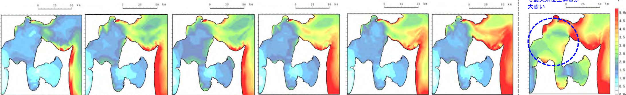
内閣府(2020a) (102) モデル
