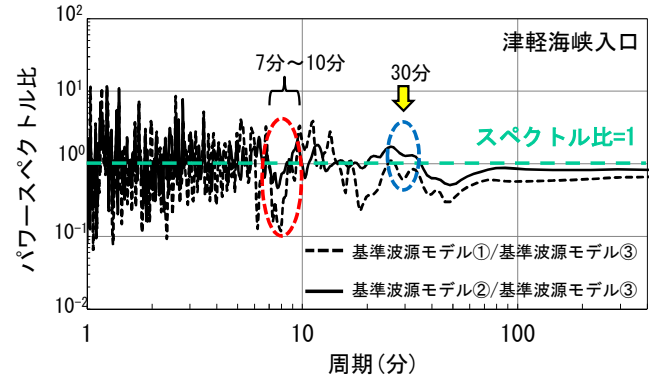
基準波源モデル③と基準波源モデル①②との比較 津軽海峡入口におけるスペクトル解析結果の比較
