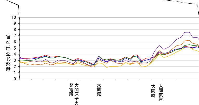
津軽海峡開口部付近沿岸における基準波源モデル①～⑥の想定津波群とイベント堆積物の比較
