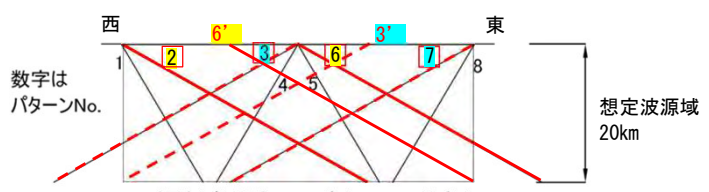
傾斜角30°のパターン分類 土木学会 (2016) (39) に基づく8パターン、 添え字' : 追加パターン、実線 : 東傾斜、破線 : 西傾斜
