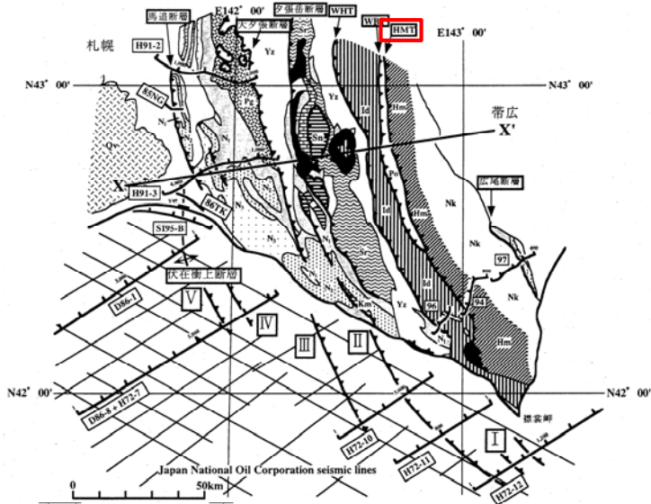
図1 日高衝突帯ならびに前縁褶曲・衝上断層帯の地質概略と主な反射法地震探査測線図。X-X'は図2の断面位置を示す。伊藤ら(1999)を改変。 【地質】主として、地質調査所(1982, 1996)による。Nk: 中の川層群, Hm: 日高変成岩類(主帯), Po: ポロシリ・オフィオライト(西帯), Id: イドソナップ帯, Yz: 蝦夷層群, Sr: 空知層群, Km: 神威古潭変成岩類, Sn: 沙流川層ニセウ層, Pg: 古第三系, N1~N3: 地質調査所(1982)に同じ。Qv: 第四紀火山岩類。 HMT: 日高主衝上断層, WBT: 西縁衝上断層, WHT: 日高西部断層群 【測線】84° 96' 37": 日高深部構造反射法探査, 85NG・86TK: 浅野ら(1990), Y97: 伊藤ら(1998), その他の測線は石油会社(1973, 1987, 1993, 1996)。
