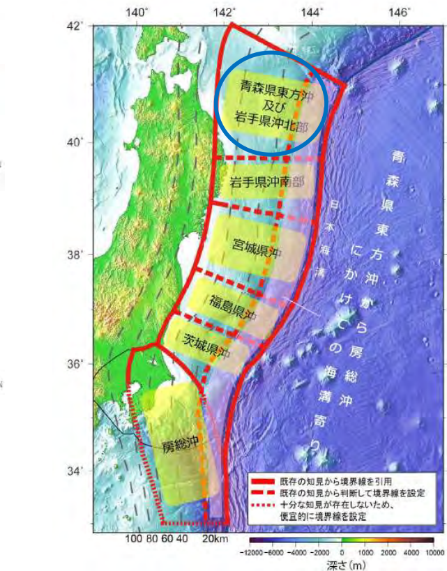
三陸沖から房総沖にかけての評価対象領域の区分け 地震調査研究推進本部 (2019) (78) に一部加筆
