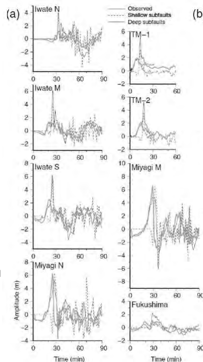
観測波形と計算波形の比較 3.11地震に伴う津波特性の分析 Satake et al. (2013) (105) に一部加筆
