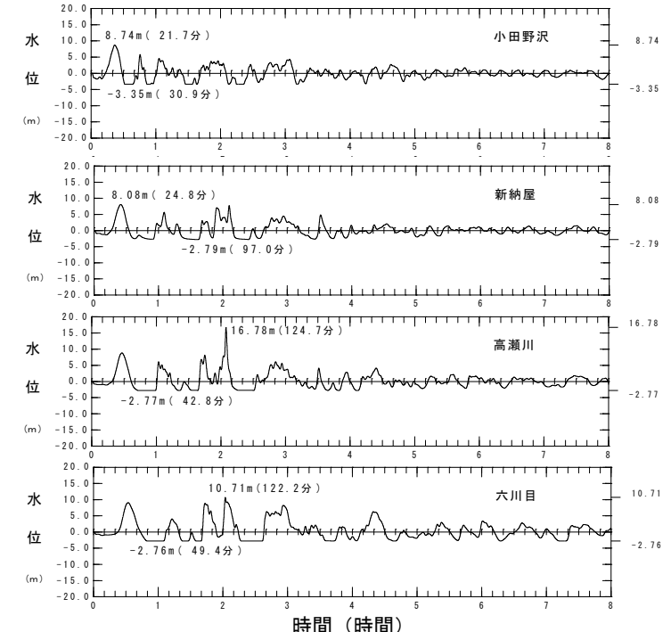
内閣府(2020a) (102) モデル
