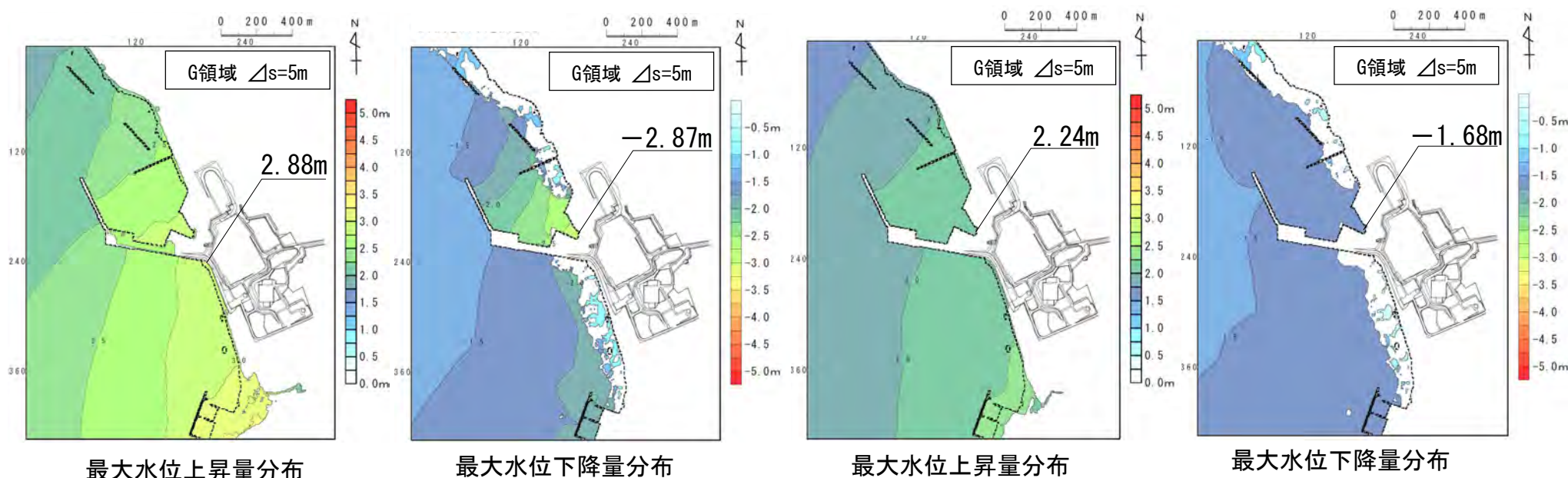
十勝沖・根室沖から色丹島沖及び択捉島沖の破壊特性を考慮した特性化モデル
