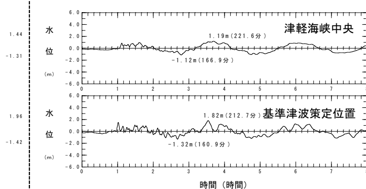
基準波源モデル⑥
