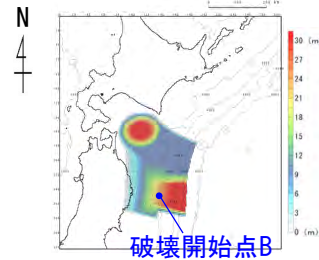
内閣府(2020a) (102) モデル
