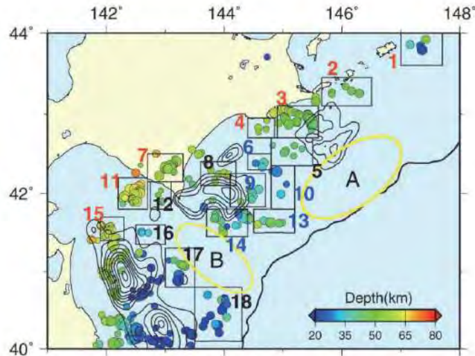
第1図. 北海道南東沖の小繰り返し地震グループの分布 (丸印). 丸の色はグループの地震の平均の深さを示す。コンターはYamanaka and Kikuchi (2004) (132)によるM7以上の地震すべり量分布。矩形は第3図で平均の積算すべりを推定した領域を示す。黄色楕円は繰り返し地震活動が低い場所。
