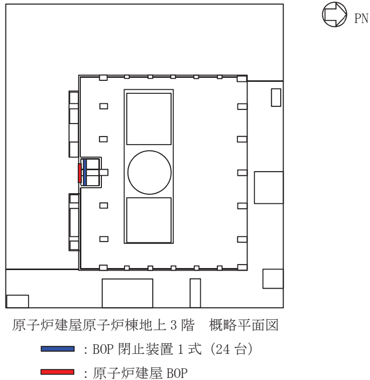
図 7-2 BOP 閉止装置の設置位置
