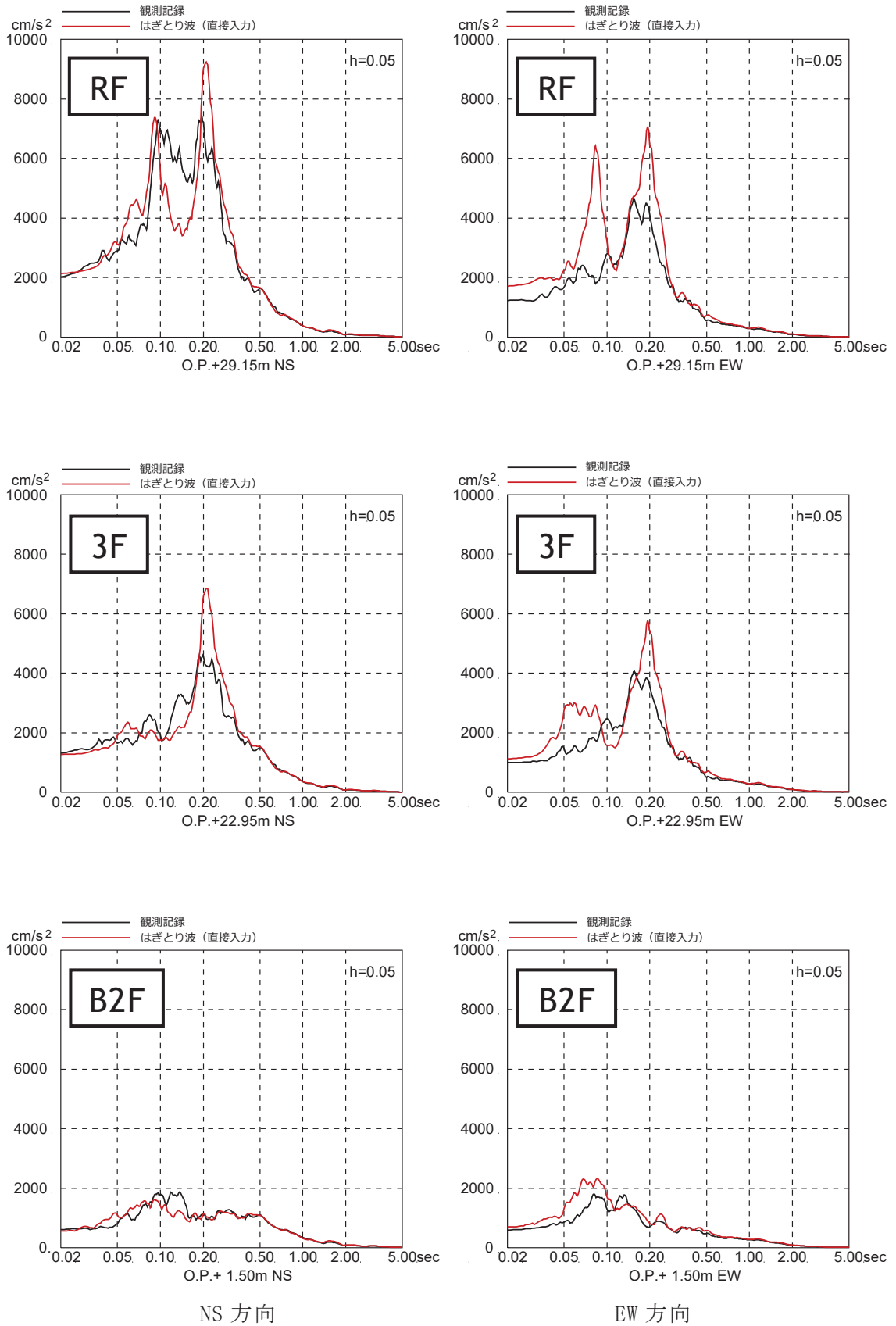
図 3. 1-7 3.11 地震のはぎとり波を入力に用いた場合のシミュレーション解析結果 (制御建屋)
