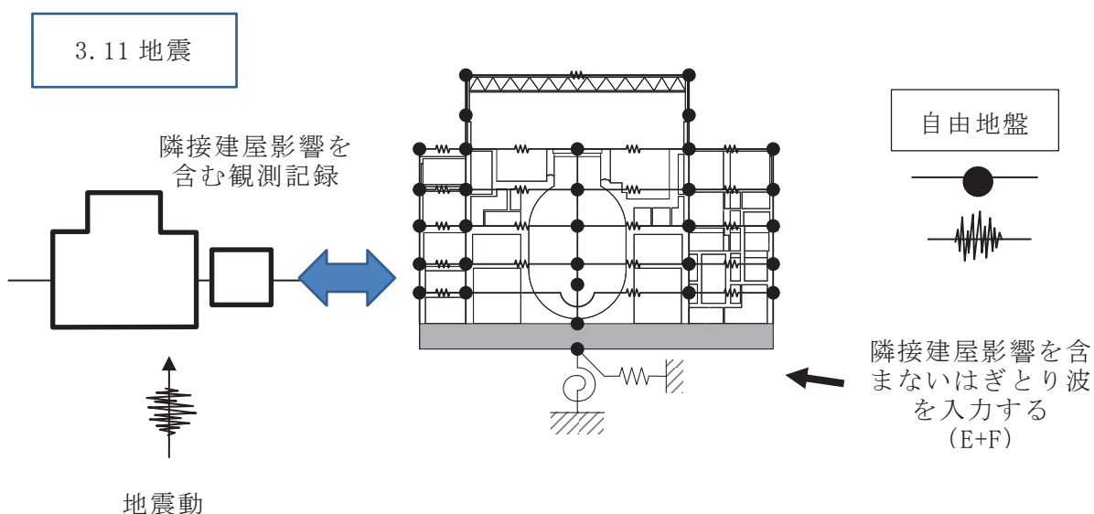
図3.1-5 3.11地震によるシミュレーション解析概要（原子炉建屋の例）
