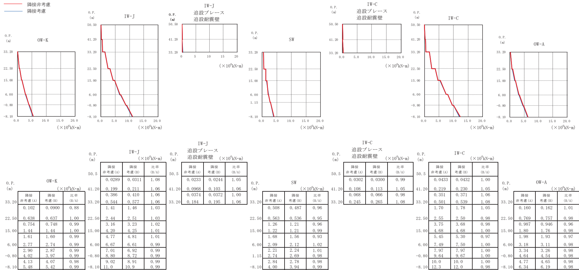
図 3.2-17 最大応答曲げモーメントの比較 (O2R/B, NS 方向)
