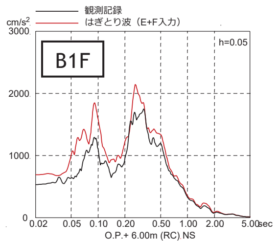
図 3. 1-6(1) 3.11 地震のはぎとり波を入力に用いた場合のシミュレーション解析結果 (原子炉建屋, NS 方向)
