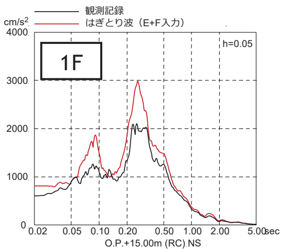
図 3. 1-6(1) 3.11 地震のはぎとり波を入力に用いた場合のシミュレーション解析結果 (原子炉建屋, NS 方向)
