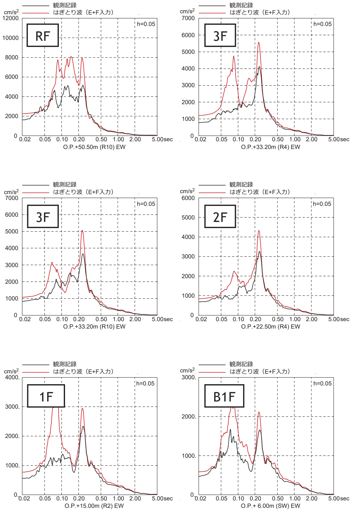
図 3. 1-6 (2) 3.11 地震のはぎとり波を入力に用いた場合のシミュレーション解析結果 (原子炉建屋, EW 方向)
