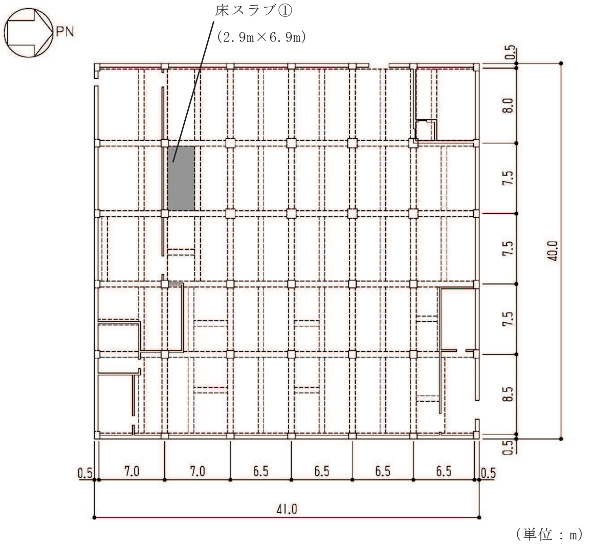
図 8-2(2) スラブの評価を記載する部材の位置 (3F, 0. P. 22.95m)
