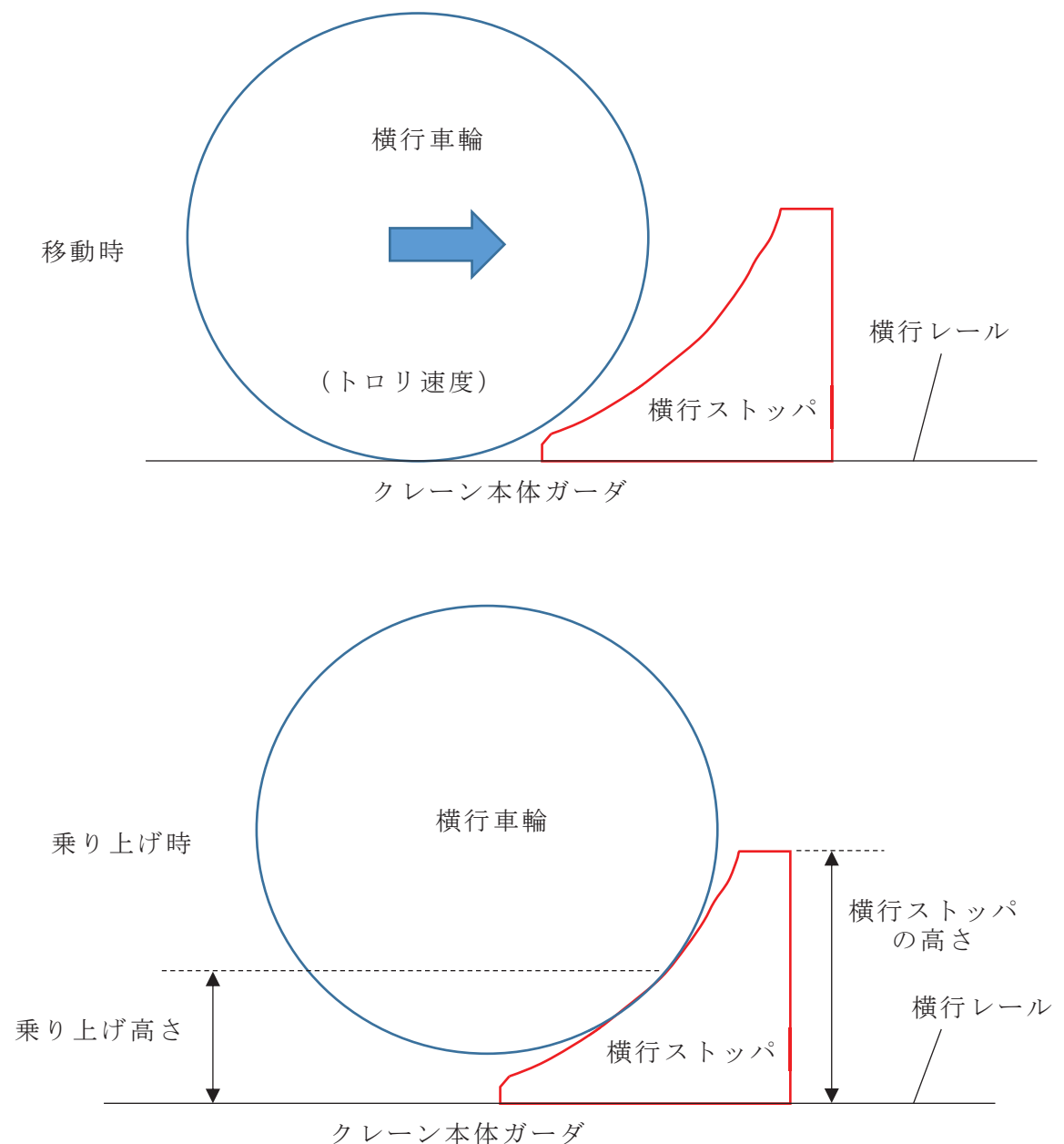
図 12-5 横行車輪と横行ストッパの接触概念図
