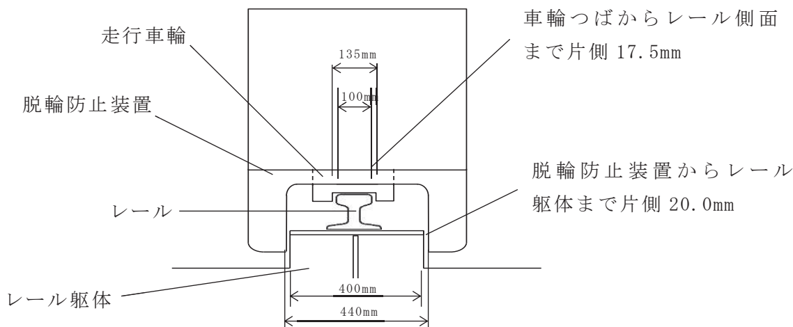
図 11-1 走行車輪と脱輪防止装置の隙間関係
