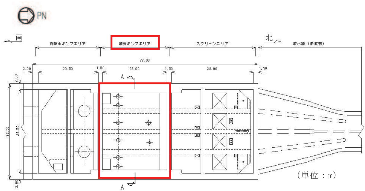
(海水ポンプ室平面図)
