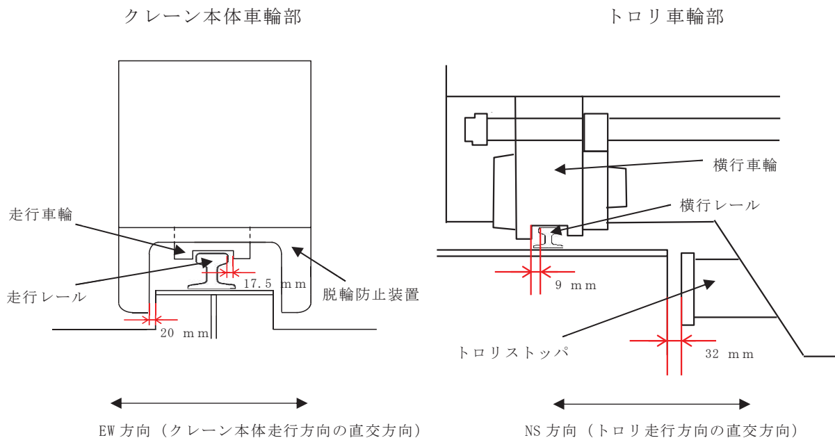
図 1-5 クレーン本体車輪部及びトロリ車輪部概要図
