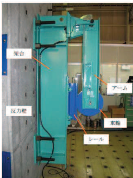
図 1-8 車輪反発係数試験体*
