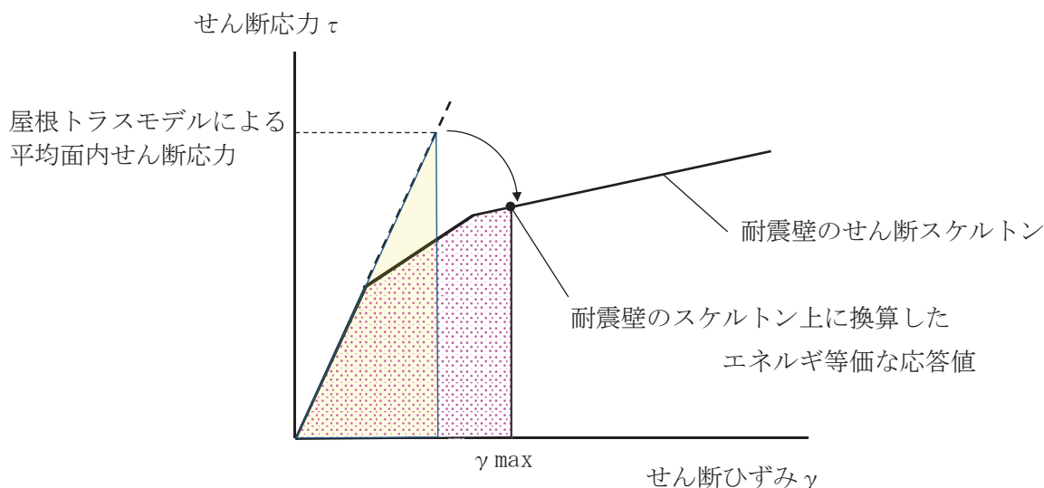
図 3-10 エネルギー一定則に基づく各耐震壁のせん断ひずみの評価方法
