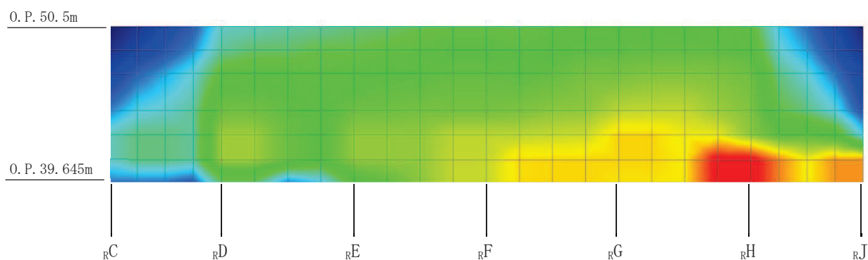
(a) 屋根トラスモデル
