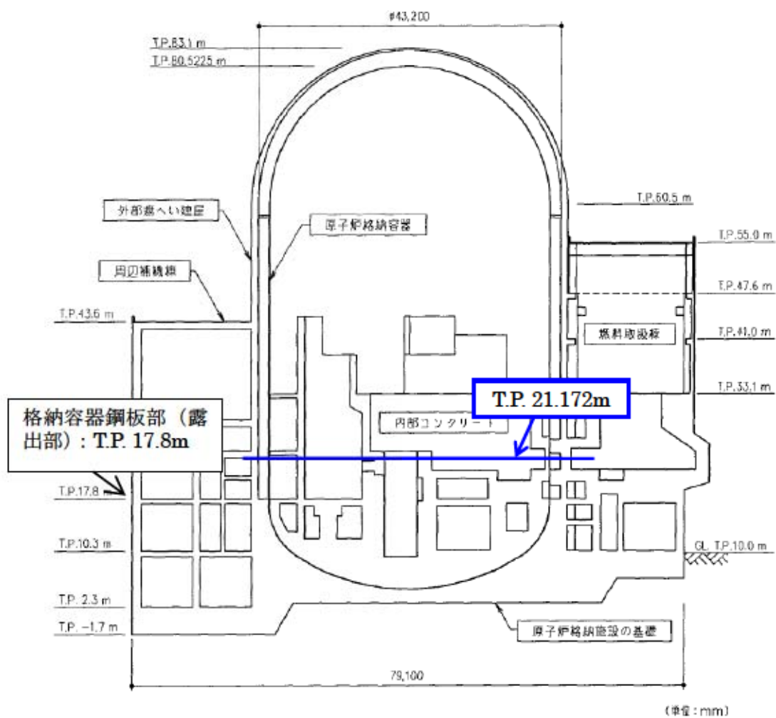
図2 原子炉格納容器断面図
