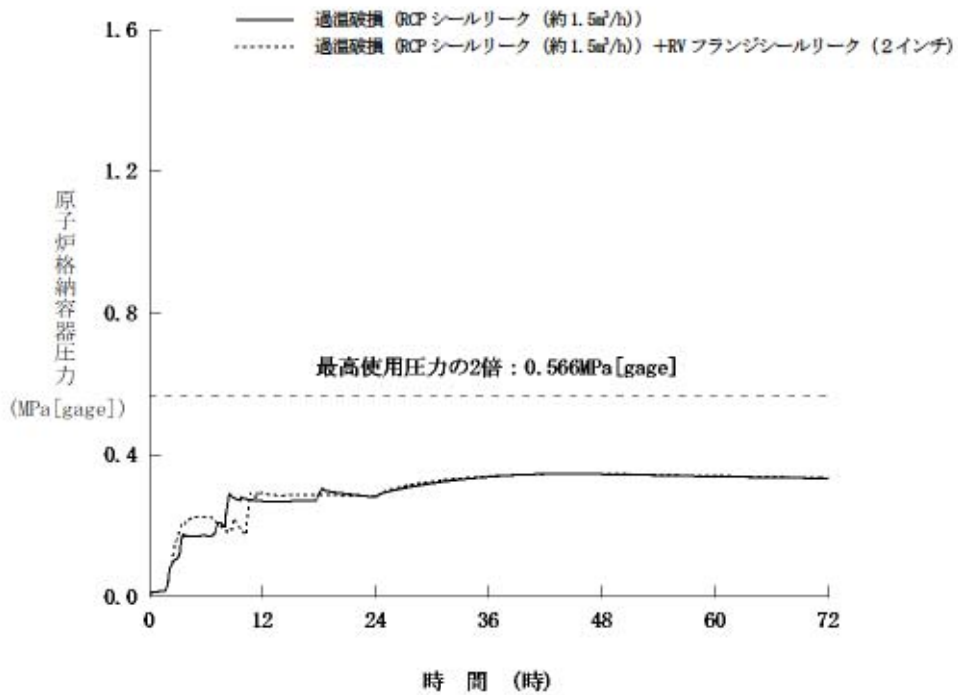
図 3-5 原子炉格納容器圧力 (RCP シールリーク (約 1.5m³/h) + RV フランジシールリーク (2インチ))
