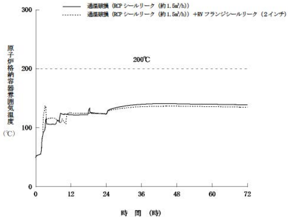
図 3-6 原子炉格納容器雰囲気温度 (RCP シールリーク (約 1.5m³/h) + RV フランジシールリーク (2インチ))
