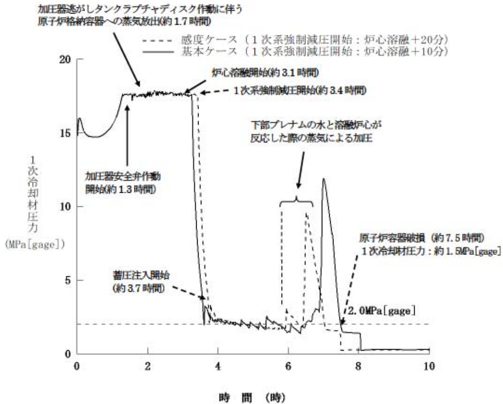
図1 1次冷却材圧力の推移 (加圧器逃がし弁開放操作開始が遅くなる場合)
