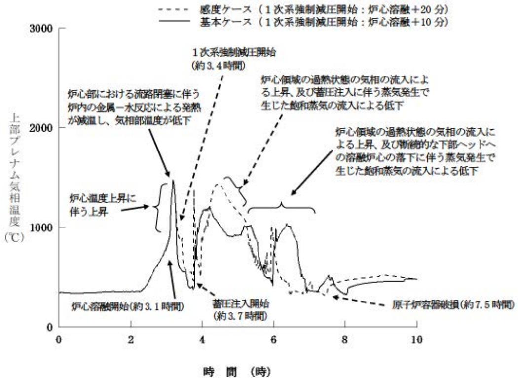
図2 上部プレナム気相温度の推移 (加圧器逃がし弁開放操作開始が遅くなる場合)
